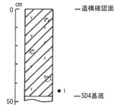
第18図 SD4覆土断面の土層柱状図
