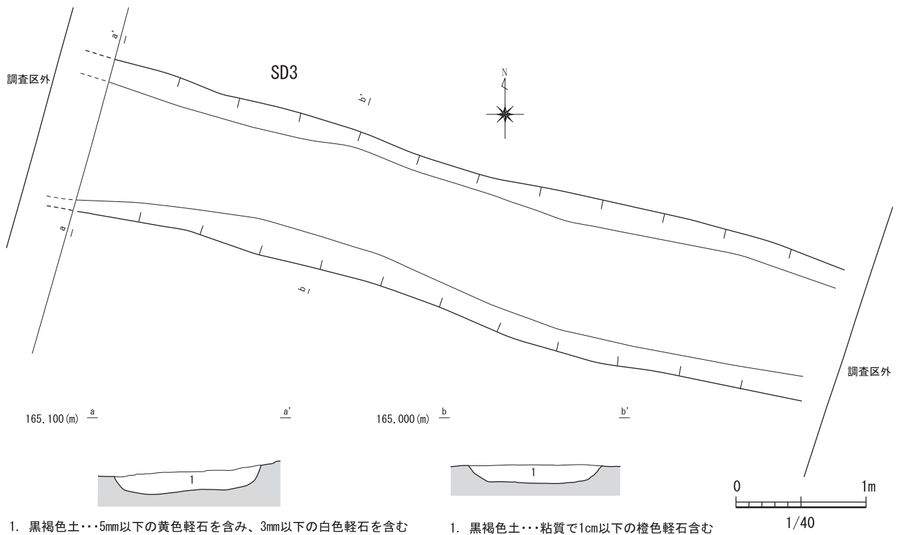
第8図 SD3 実測図 (S=1/40)
