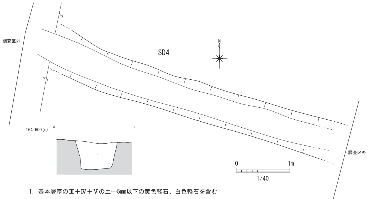
第9図 SD4 実測図 (S=1/40)
