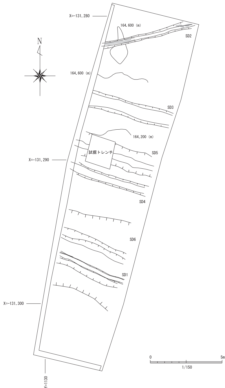
第5図 外ノ口遺跡遺構配置図 (S=1/150)
