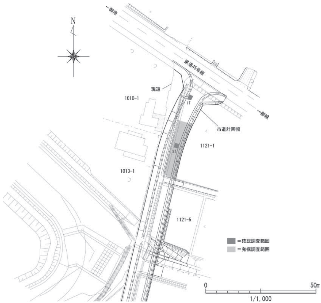
第3図 調査トレンチ配置図 (S=1/1,000)
