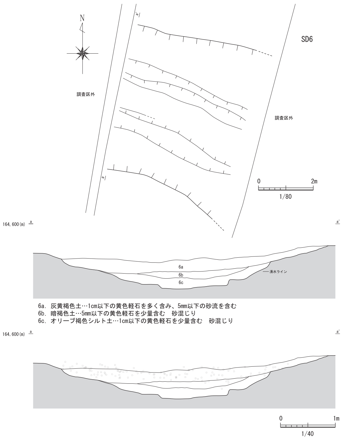
第11図 SD6実測図 (S=1/40 1/80)
