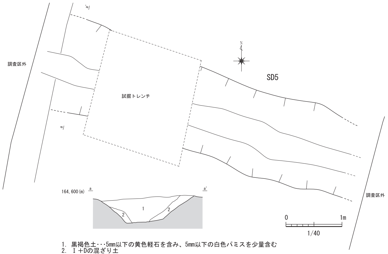
第10図 SD5 実測図 (S=1/40)
