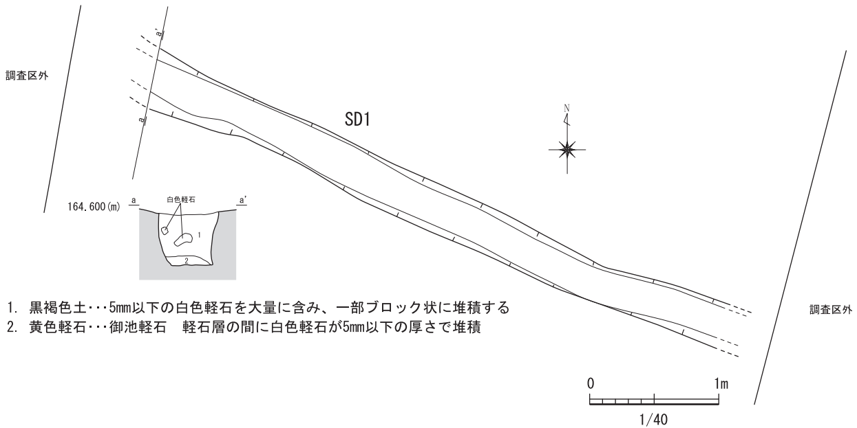
第6図 SD1 実測図 (S=1/40)
