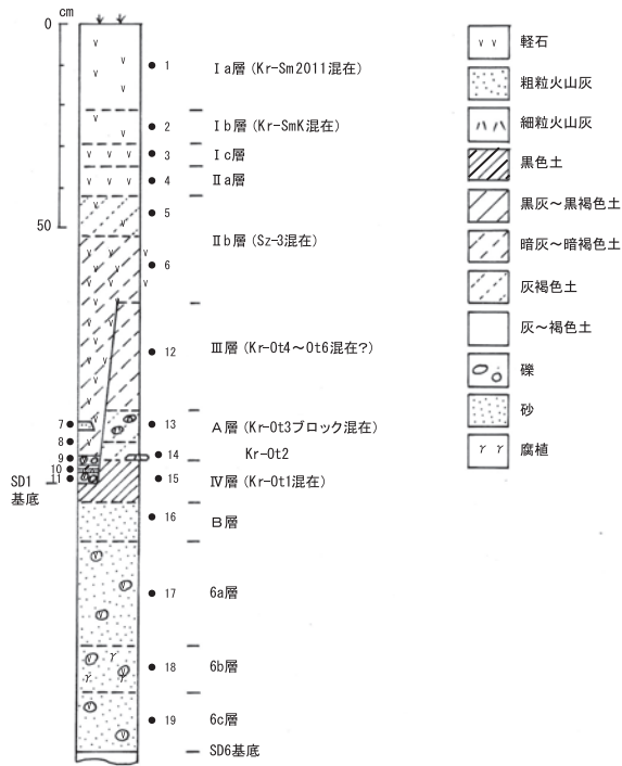
第17図 SD6・SD1覆土断面の土層柱状図
