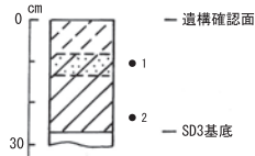
第20図 SD3覆土断面の土層柱状図
