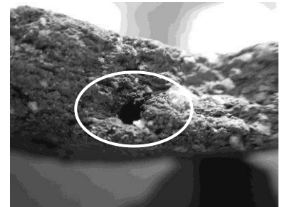
図 4-4 圧痕 (ISKD-R050)
