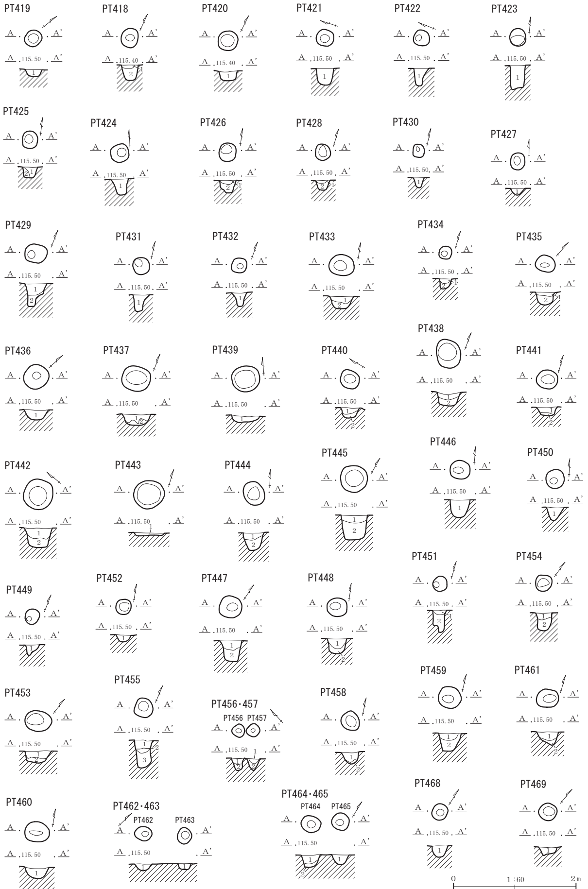
第46図 ピット (9)
