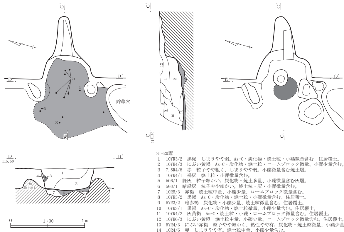
第28図 SI-20
