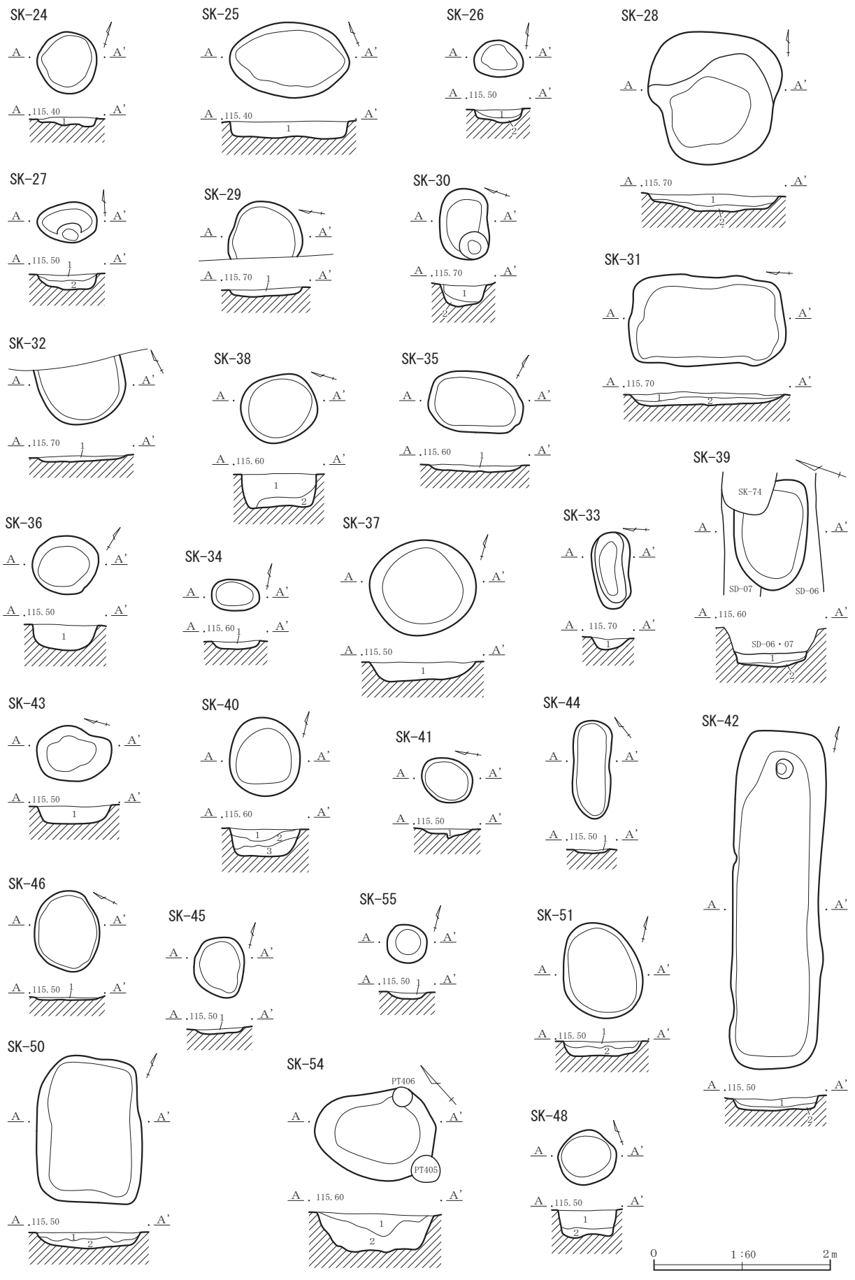
第63图 土坑 (2)
