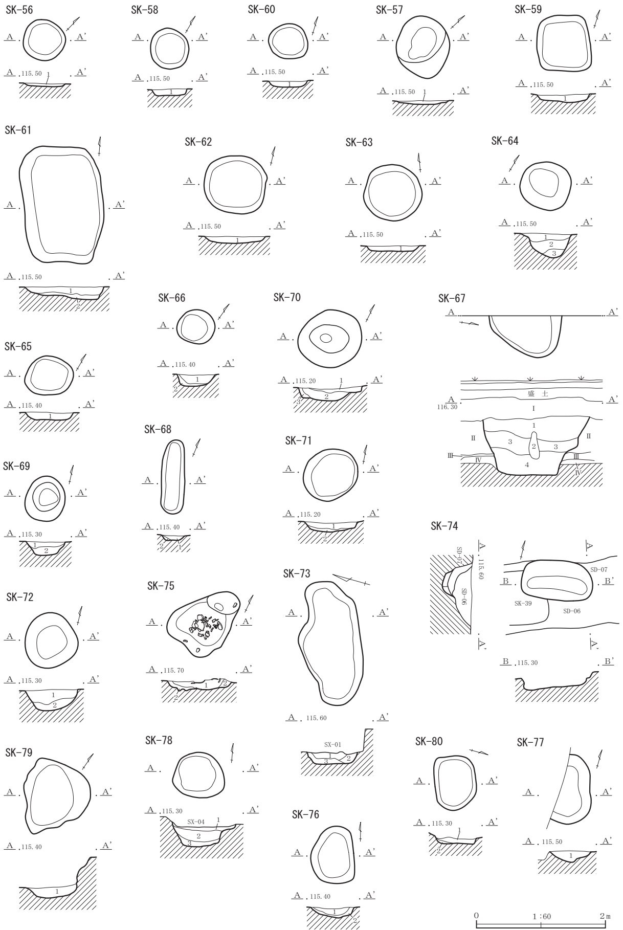
第64图 土坑 (3)
