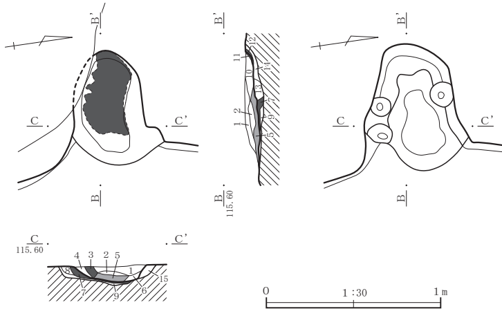
第33図 SI-25・27
