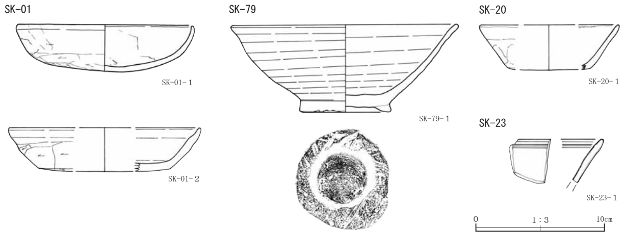
第68図 土坑（7）
