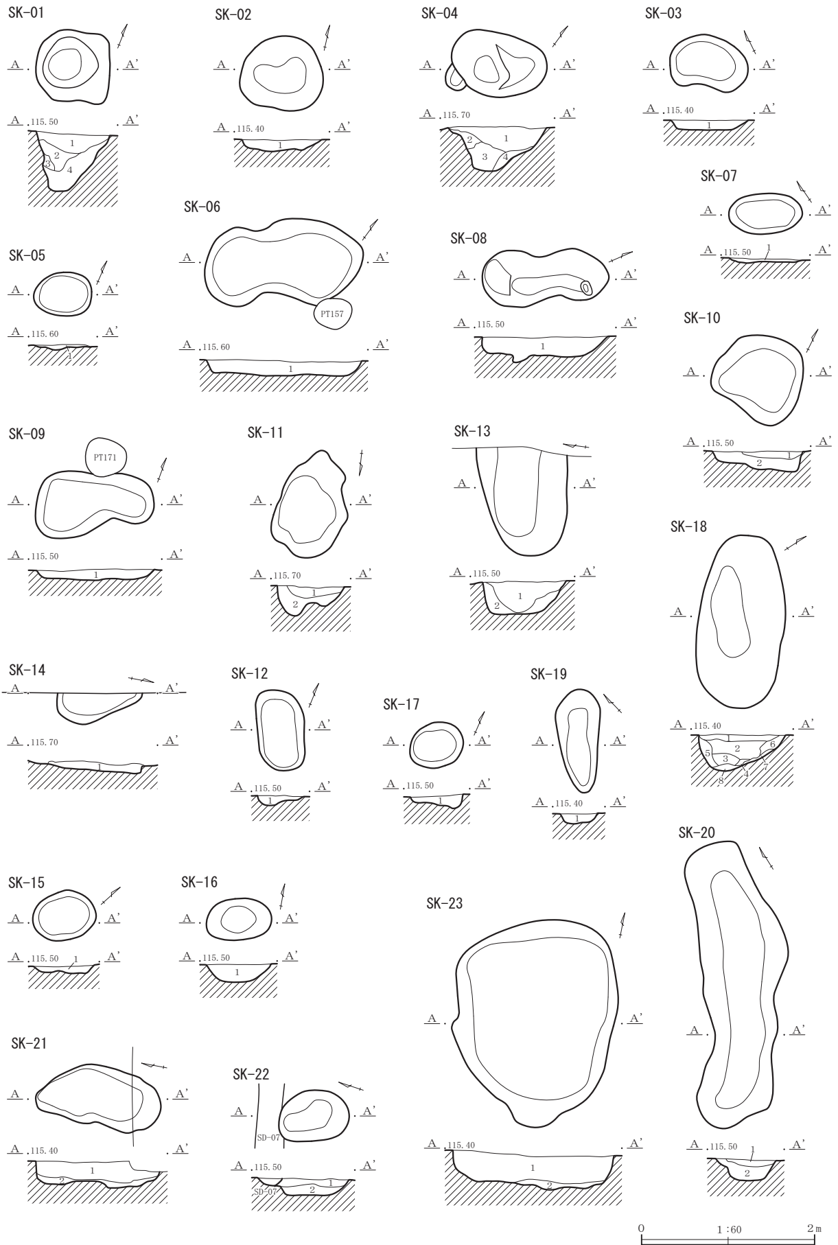
第62图 土坑 (1)
