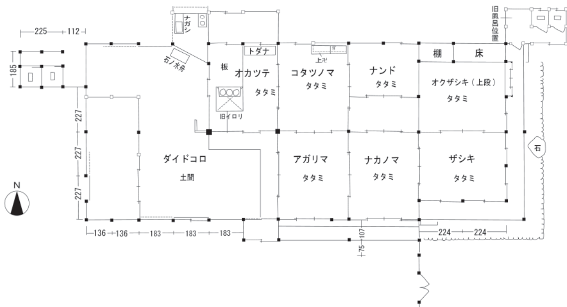
中村家住宅 平面図
