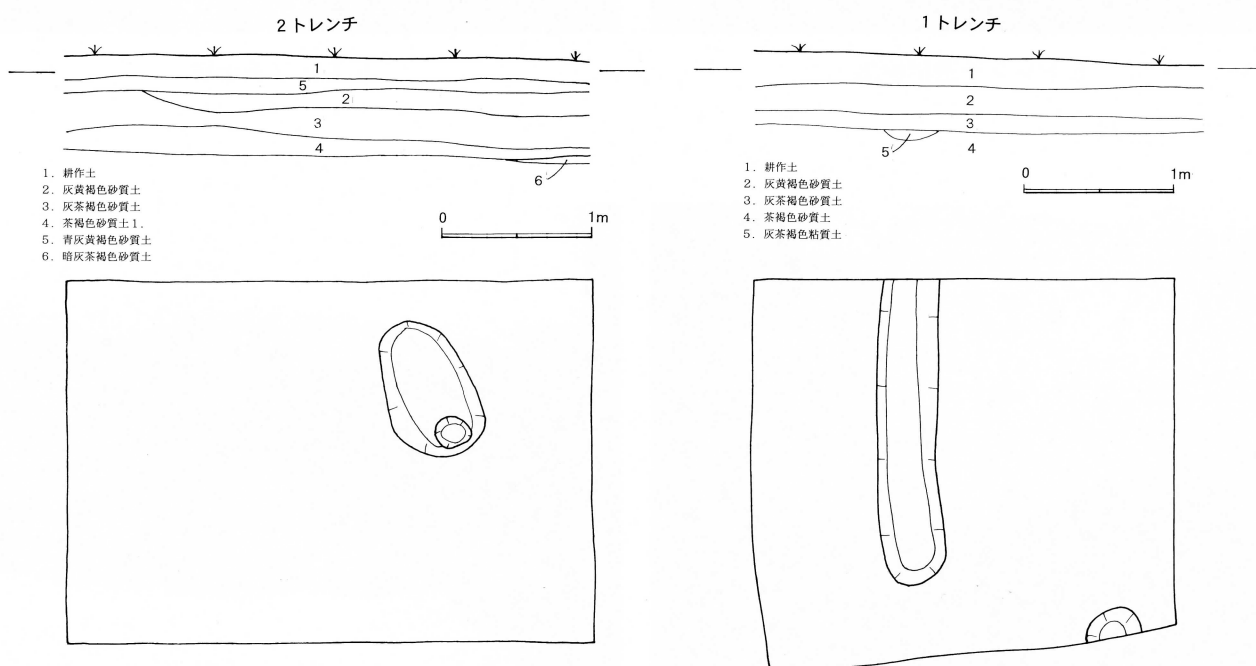
第21図 平面図
