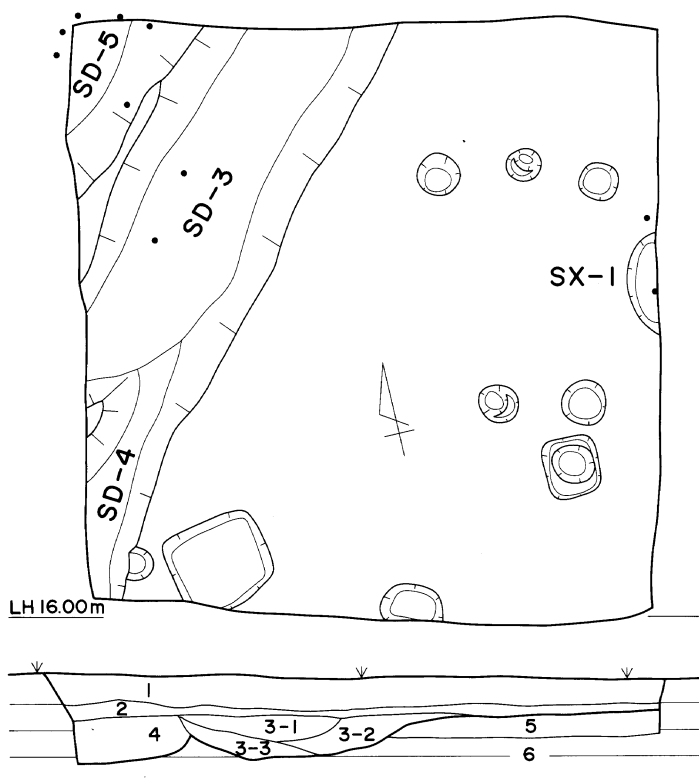
第3図 第2グリット平面図
