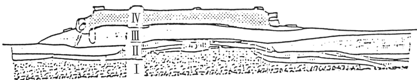
基壇築成図
