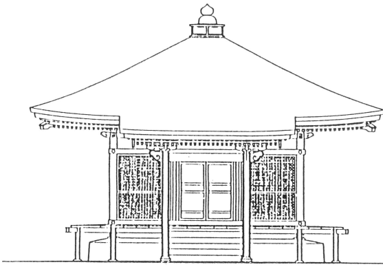
図 6 竣工正面図
