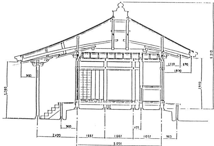
図 9 竣工縦断面図 (桁行)
