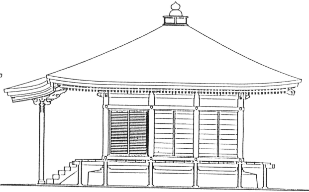
図 7 竣工側面図
