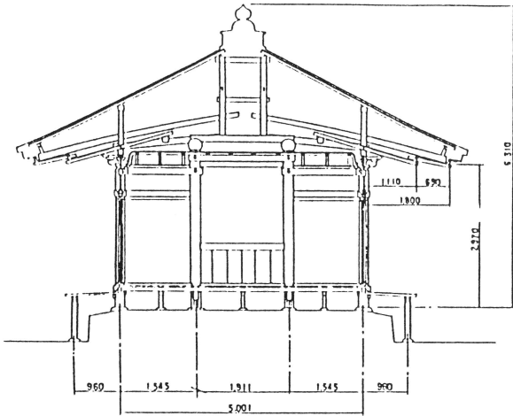
図 8 竣工横断面図 (梁行)
