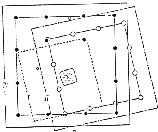
図2 基壇築成平面図
