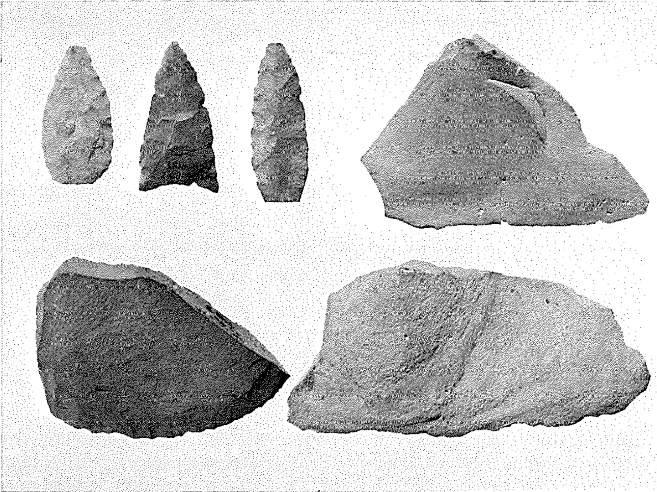
石器類
