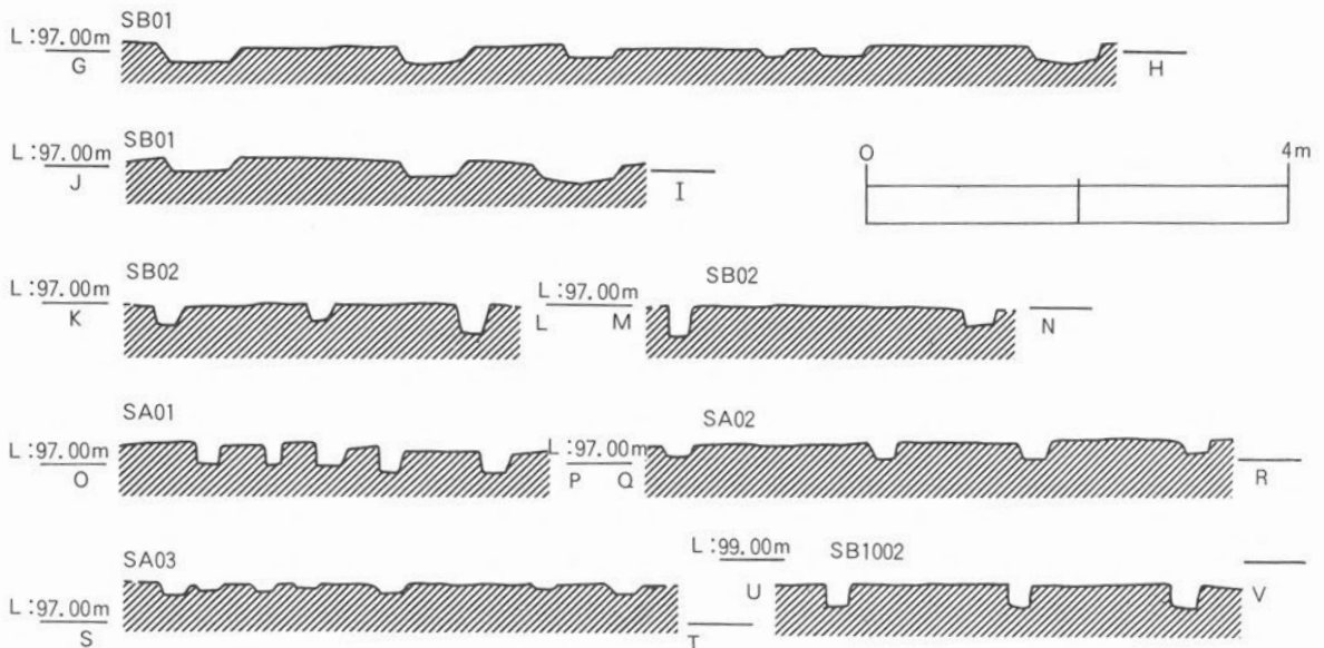
図6 SB・SAエレベーション
