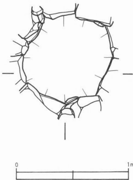
图7 S E01平面、立面图
