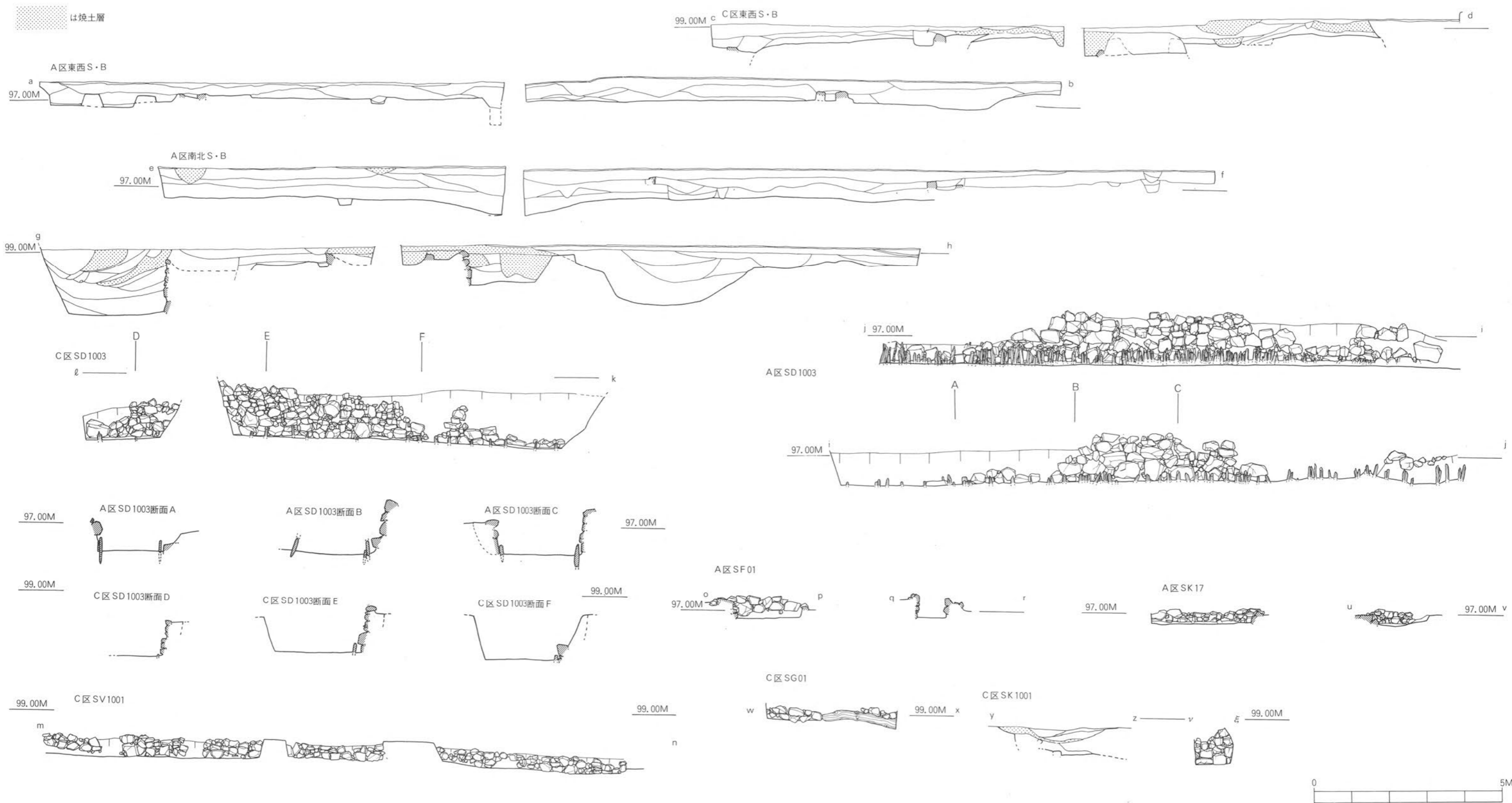
图5 土层构造立面图
