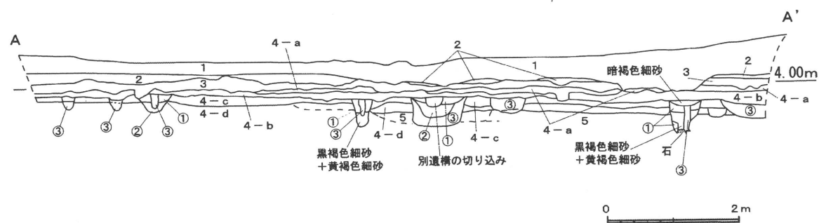
1 トレンチ平面図・断面図
