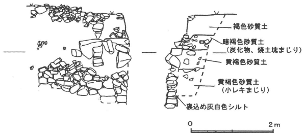
第3地点護岸石垣立面図・断面図
