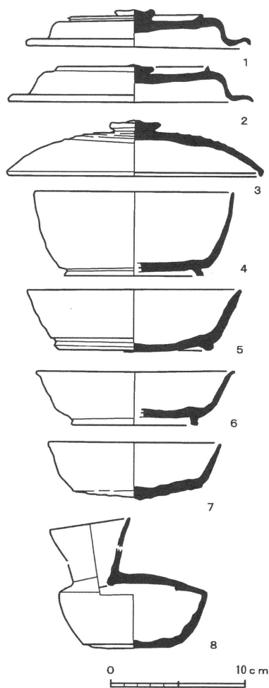
土坑9出土遺物実測図
