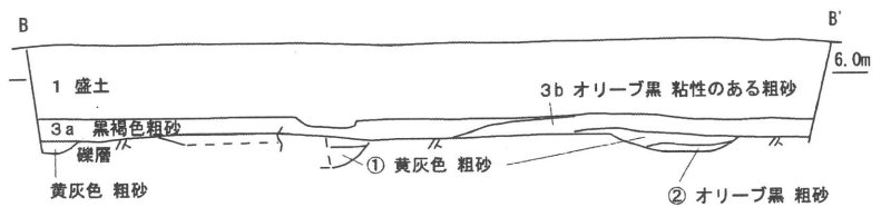
6トレンチ
