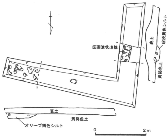
第2地点調査区平面図・断面図
