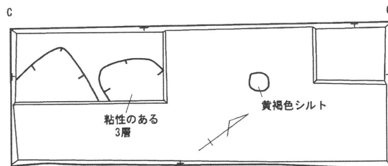
8トレンチ
