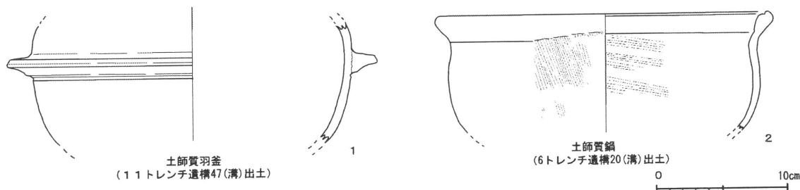
遺物実測図
