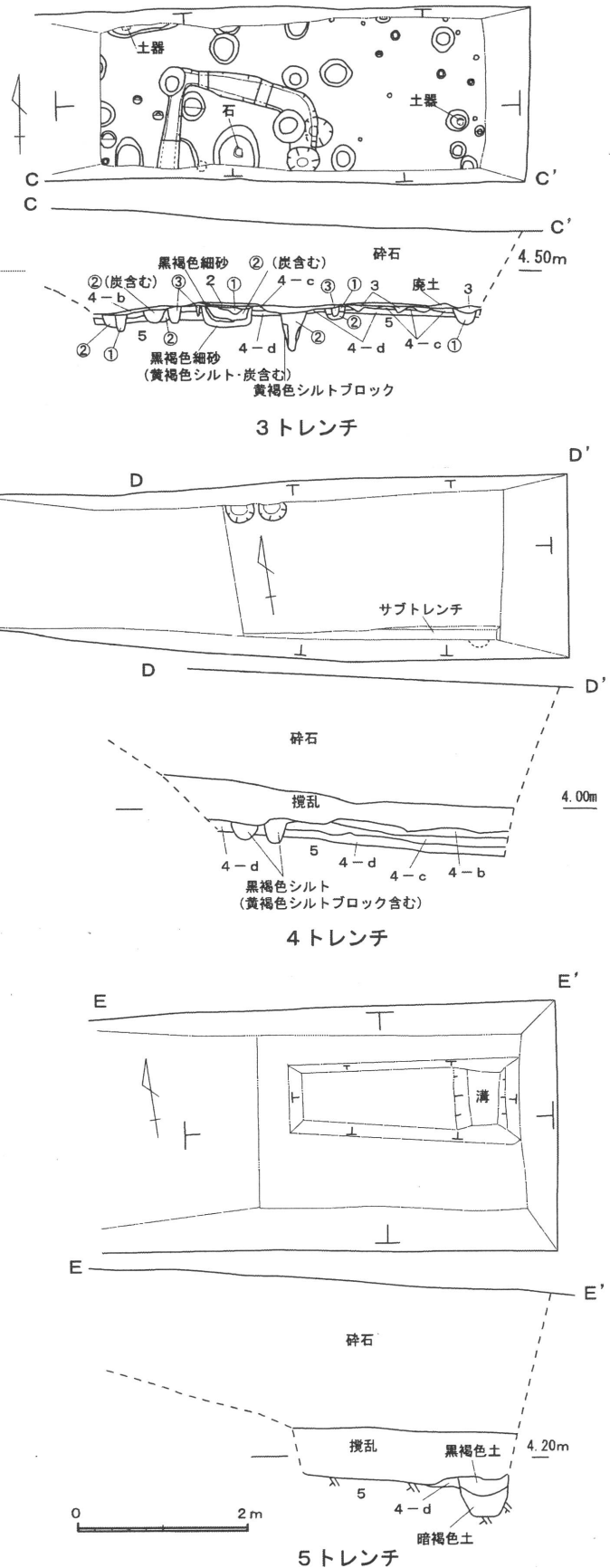
トレンチ平面図・断面図
