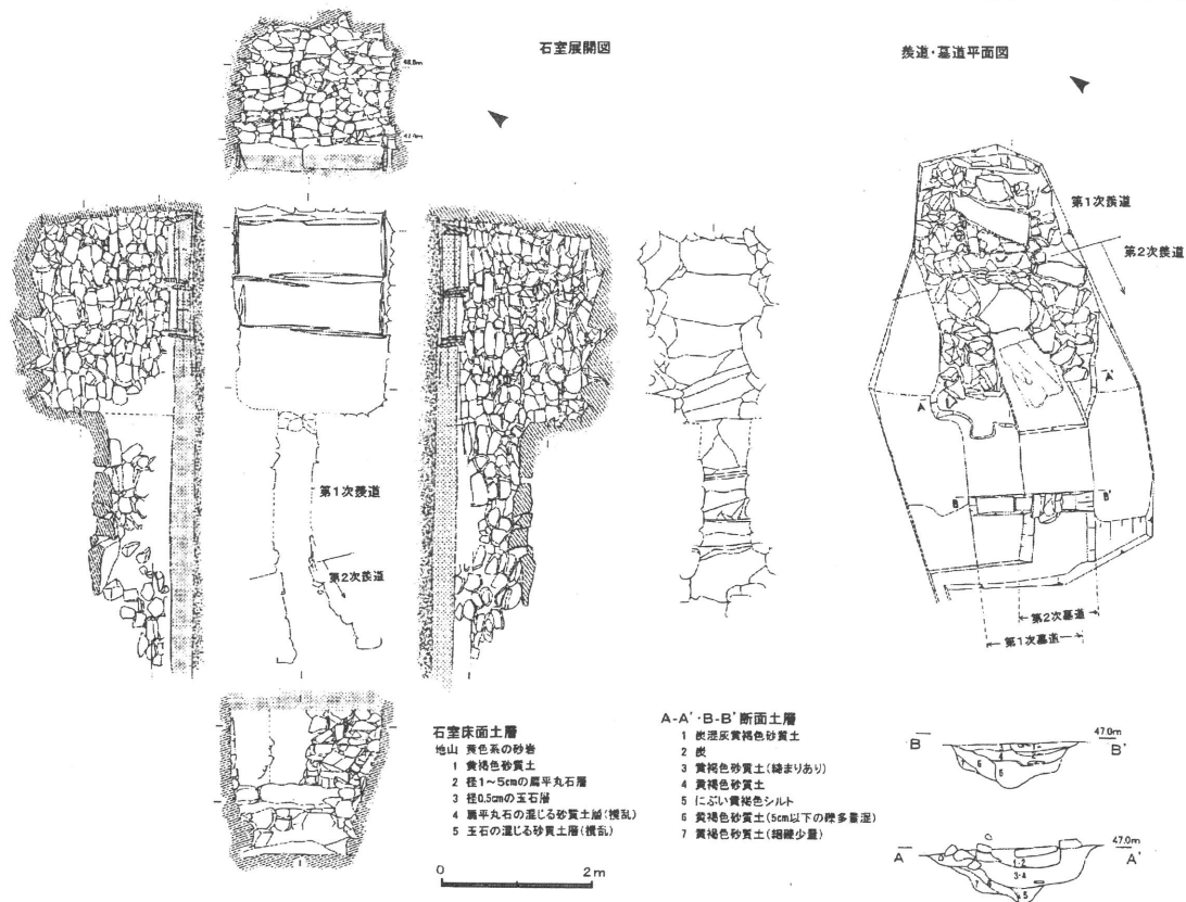
石室実測図（報告書より引用）
