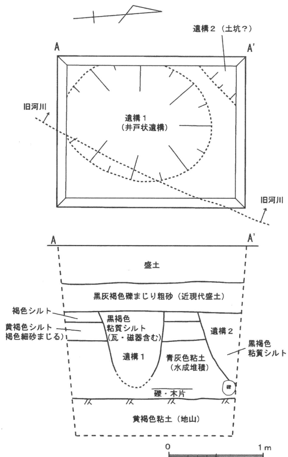
トレンチ図 (01-69)
