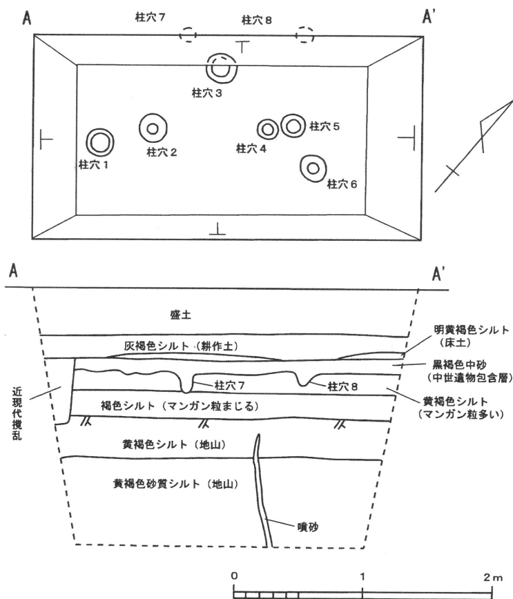
トレンチ平面図・断面図
