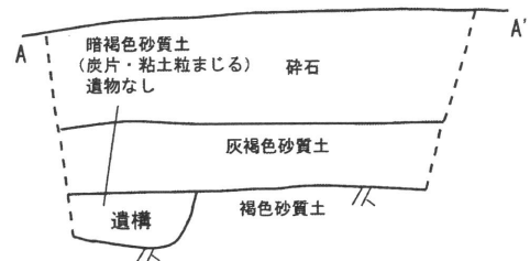
渋田遺跡遺構平面図・断面図(②01-114)
