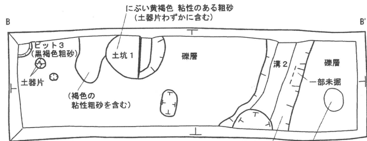
7トレンチ
