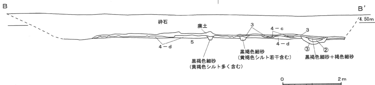
2 トレンチ平面図・断面図
