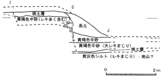
第1地点土層断面図
