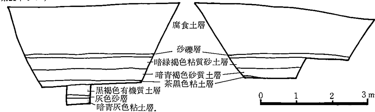
第21トレンチ
