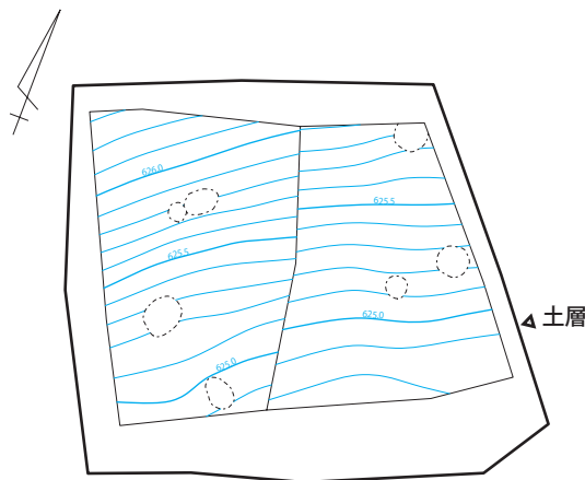
第 20 図 トレンチ配置図 (1/120)・土層図 (1/20)
