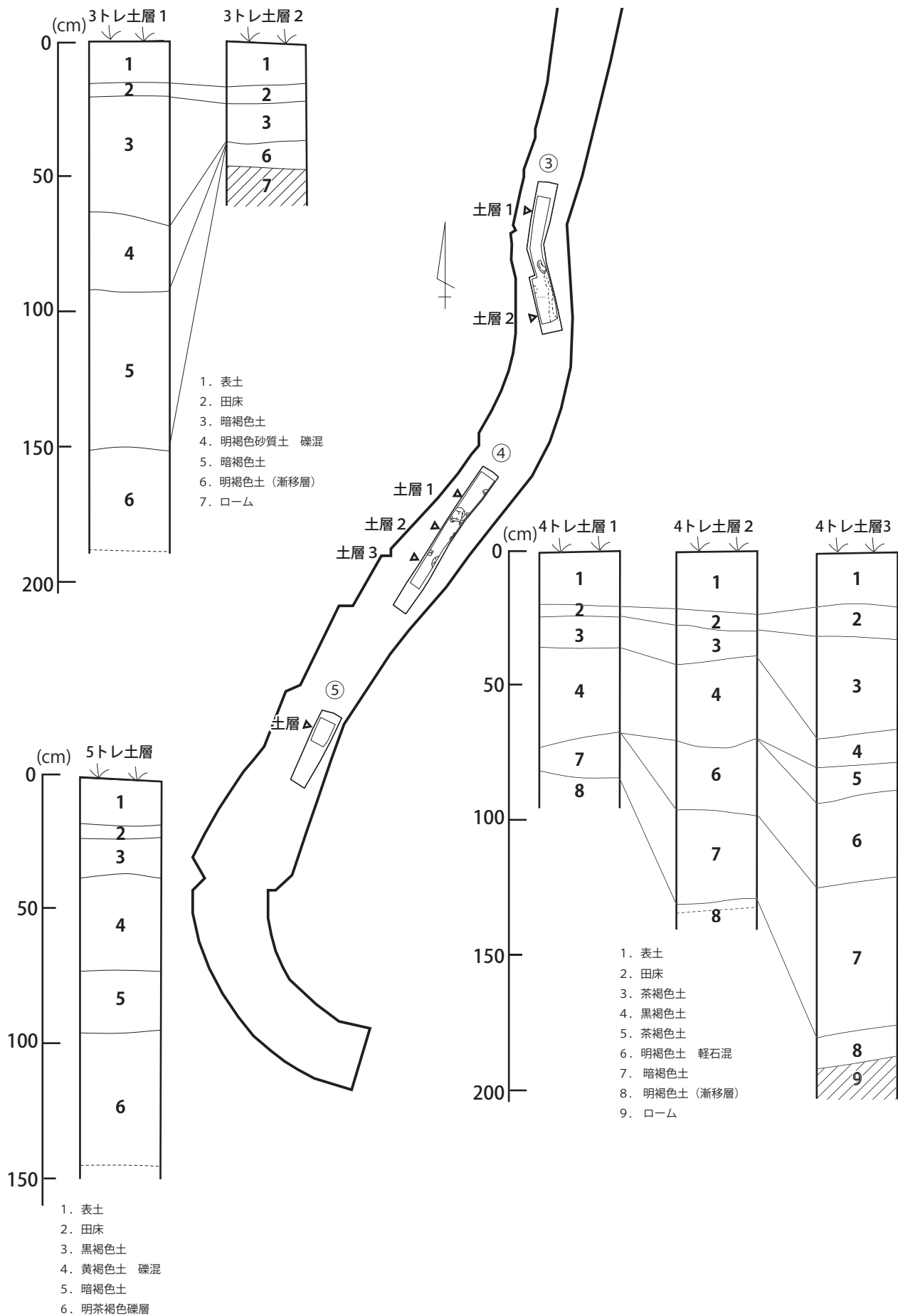
第 29 図 トレンチ配置図<3~5トレ> (1/500)・土層図 (1/20)
