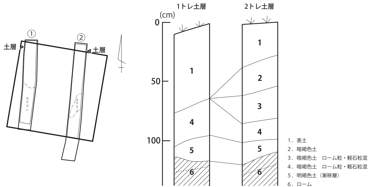
第 17 図 トレンチ配置図 (1/300)・土層図 (1/20)
