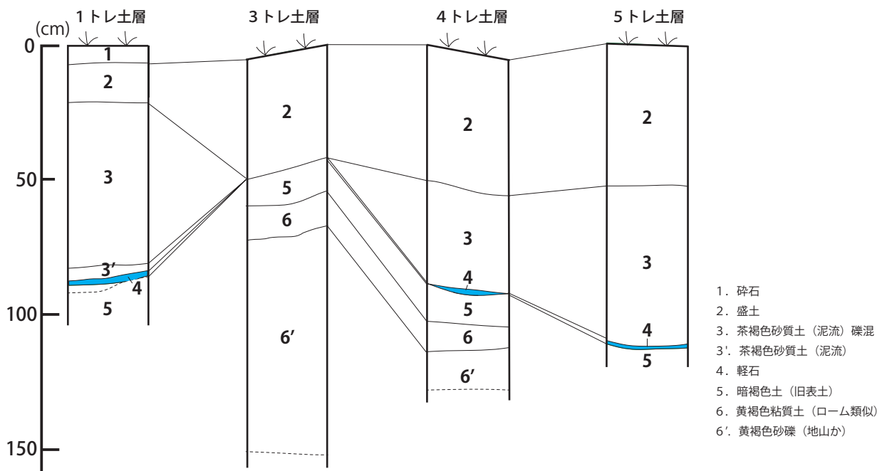
第 23 図 トレンチ配置図 (1/800) ・土層図 (1/20)
