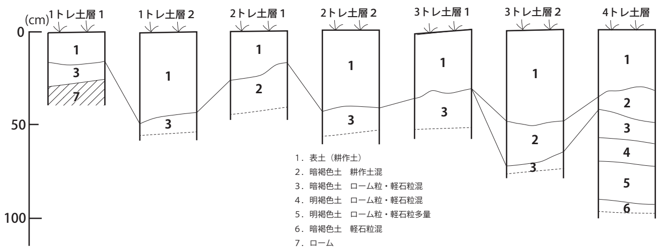
第 14 図 トレンチ配置図 (1/200) ・土層図 (1/20)
