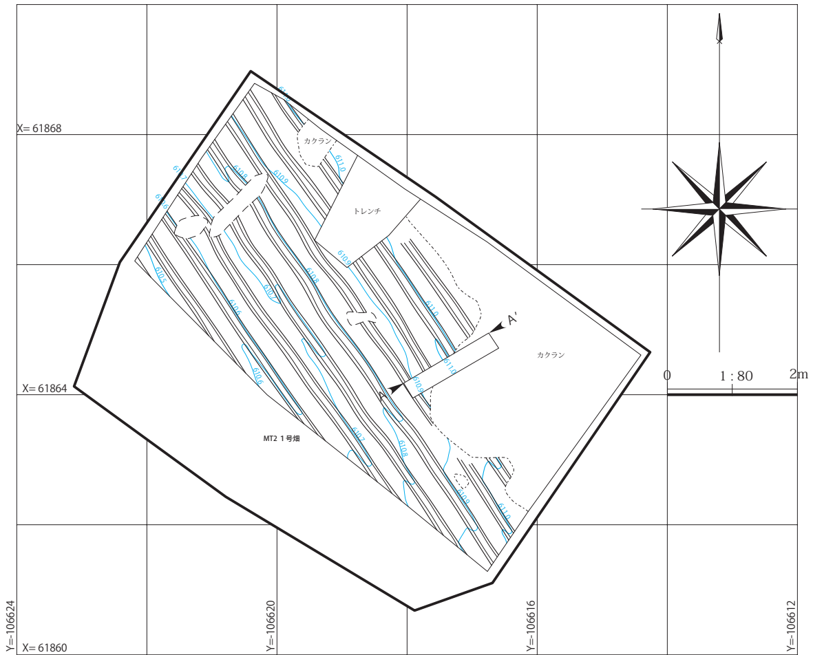
第5図 町遺跡Ⅱ全体図 (1/80)
