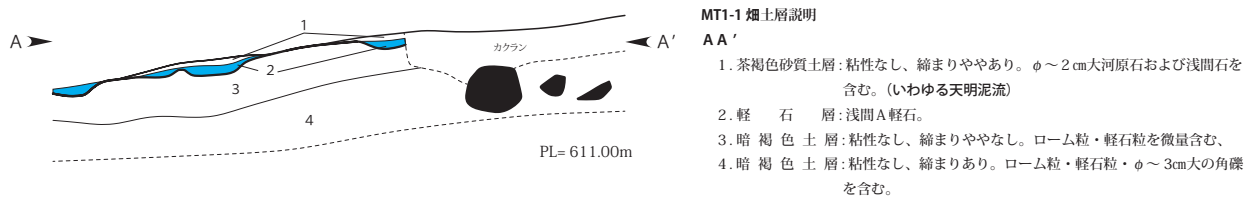
第6図 MT2 1号畑サブトレ土層図 (1/20)
