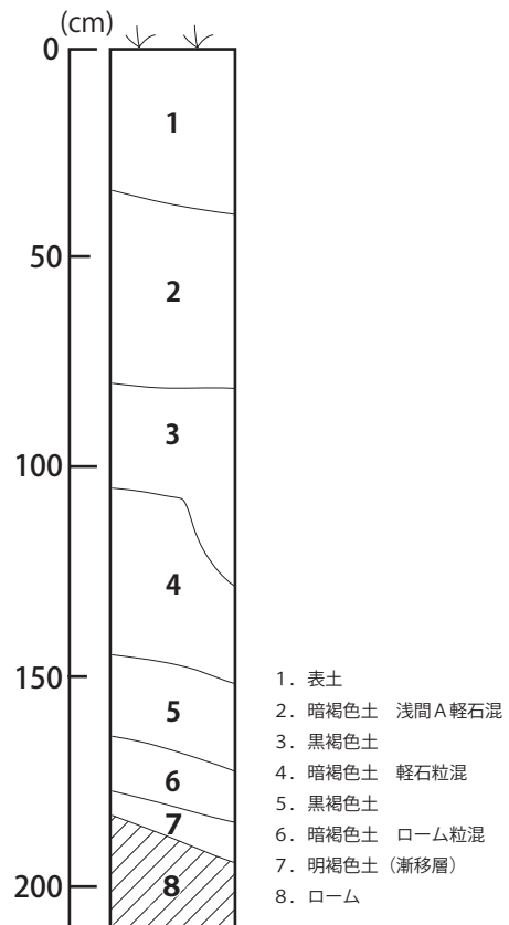
第 20 図 トレンチ配置図 (1/120)・土層図 (1/20)
