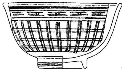
图9 遗物实测图1 (盖·碗 (1/2))
