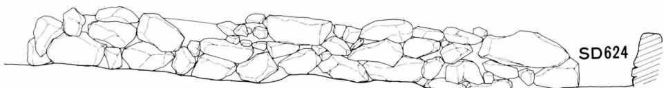
石組溝SD625 西立面図(道路SS621 横断部)
