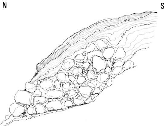
◀ 同上 西面石垣実測図
