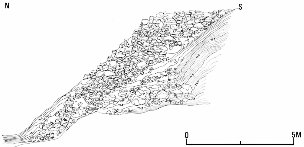
中の御殿北西隅石垣実測図
