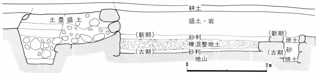
挿図1 土壘・道路断面図
