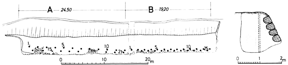
石垣グラウト工法図
