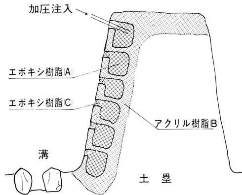
樹脂加工断面図
