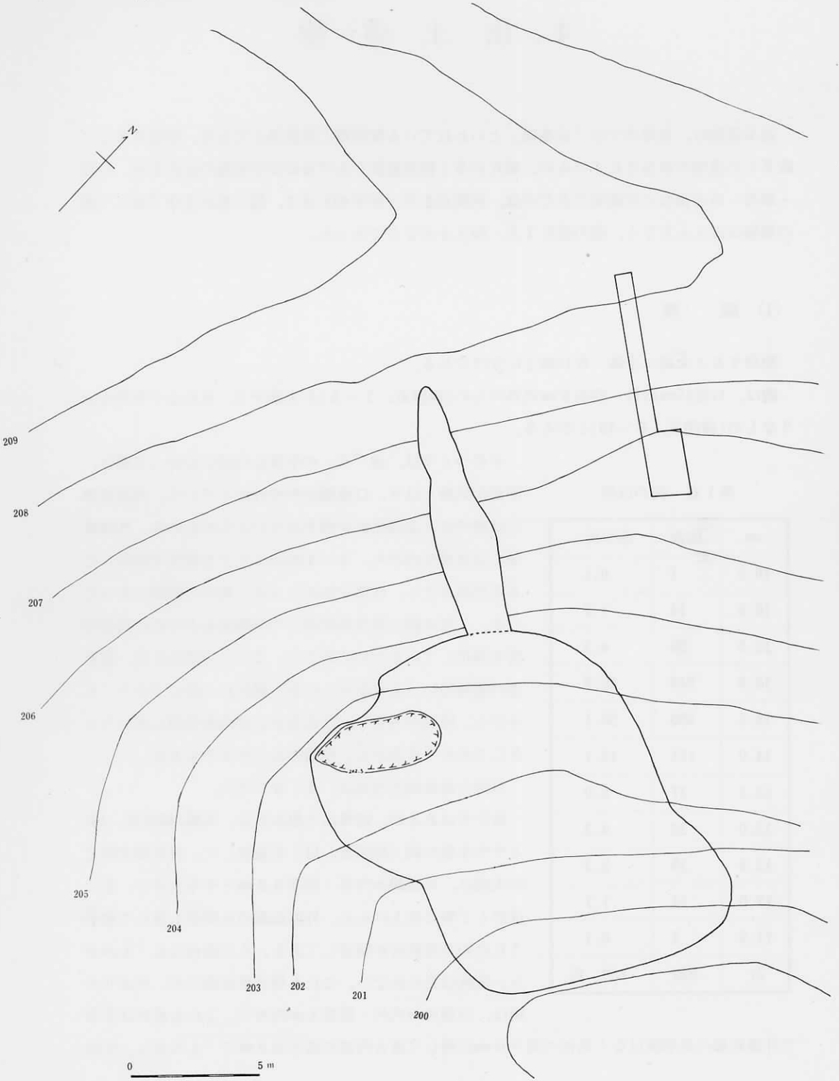
插图四 柿下古窠实测图
