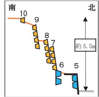
石積み 5~10 断面図
