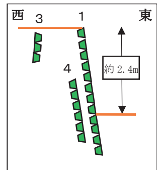
石積み 1・3・4 断面図
