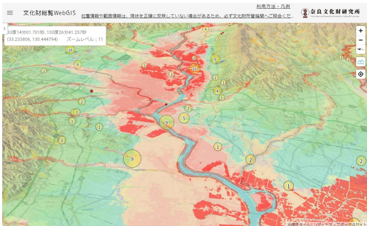
図1 文化財総覧 WebGIS にて筑後川流域を表示 (令和 5 年 6 月の大雨浸水想定区域とハザードマップ)
