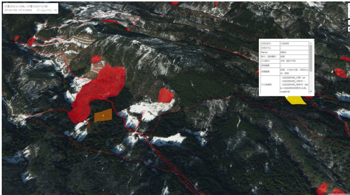
図1 石川県珠洲市、文化財(黄色い点とオレンジ)・斜面崩壊箇所(赤)を表示
