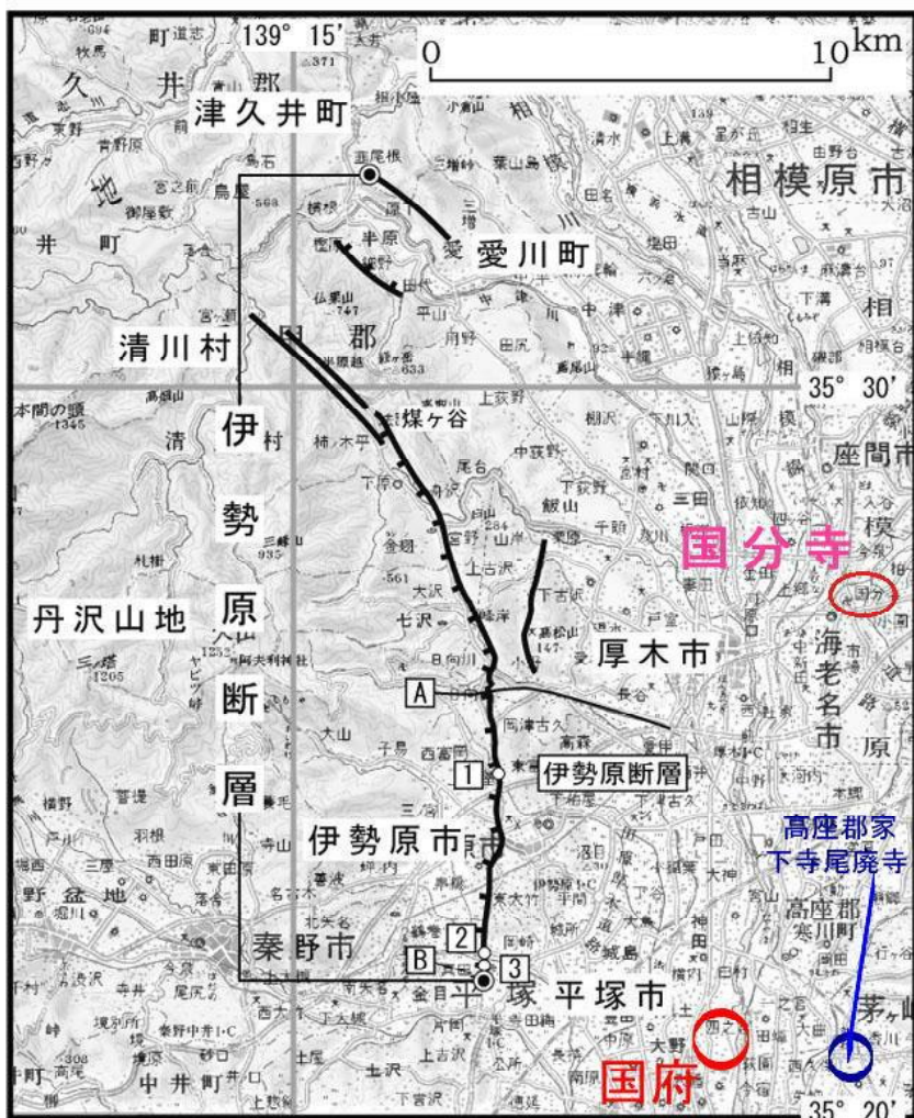
地震調査研究推進本部 H.P. の掲載図「伊勢原断層」に加筆
