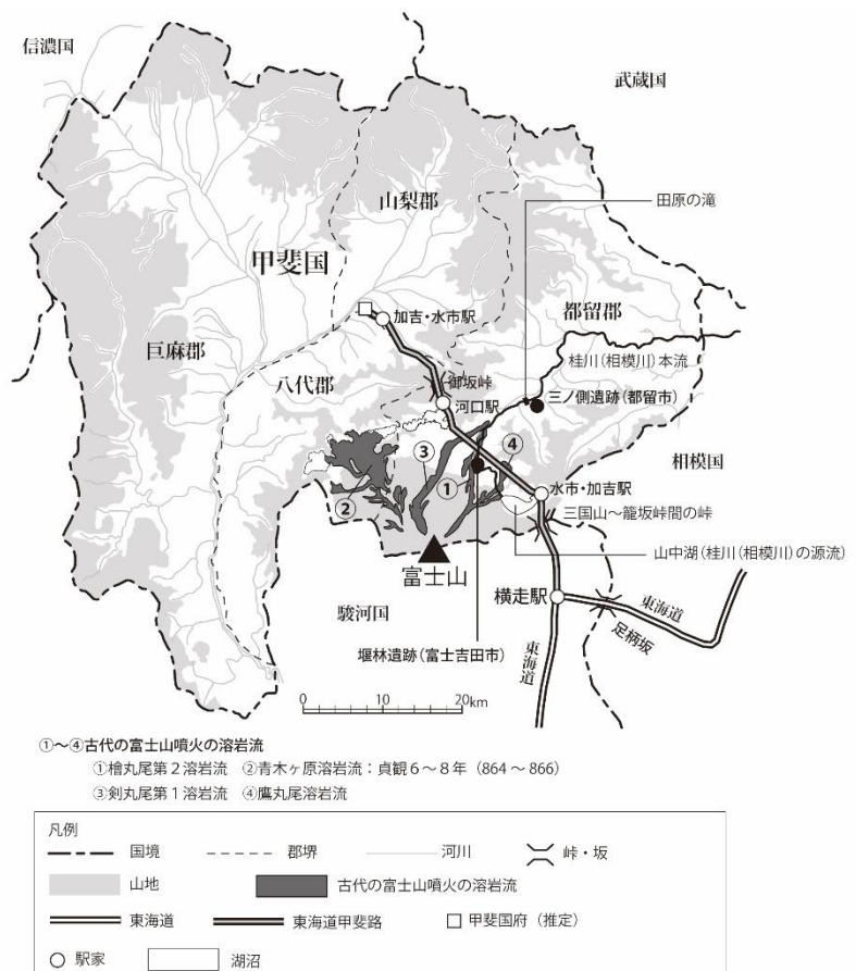
図6 古代東海道甲斐路と溶岩流・遺跡位置図 (杉本 2020 より転載・改変)
