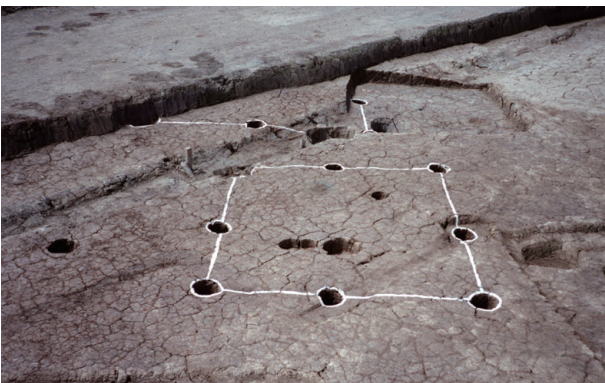
4 第9・10号掘立柱建物跡
