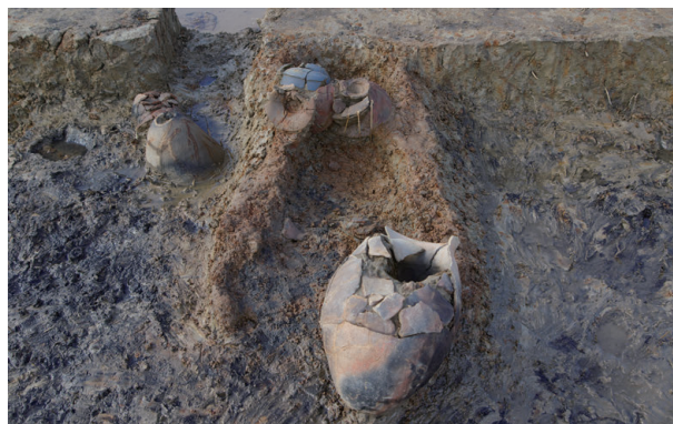
7 第 112 号住居跡カマド遺物出土状況 (3)
