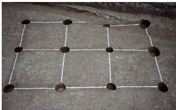
3 第4号掘立柱建物跡
