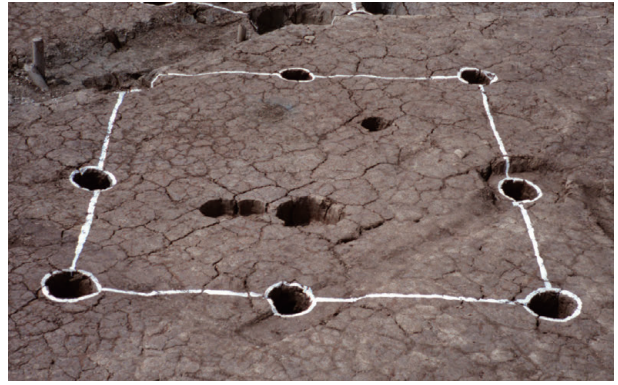
5 第9号掘立柱建物跡
