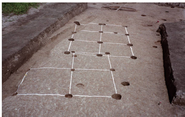
4 第4・5号掘立柱建物跡
