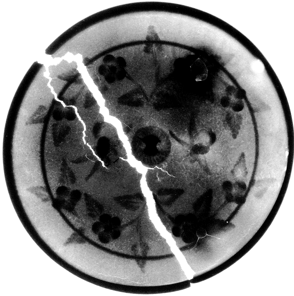
第106号土壙出土山吹双鳥鏡 X 線透過写真
