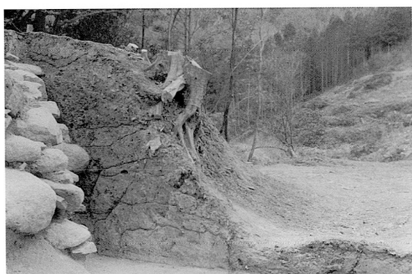
西トレンチの断面
