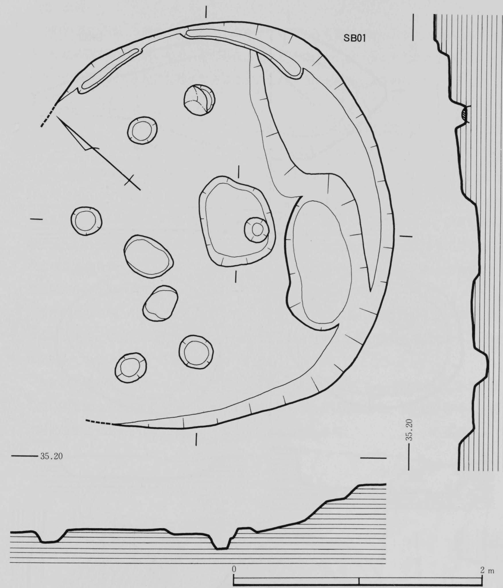
第5図 竪穴住居実測図
