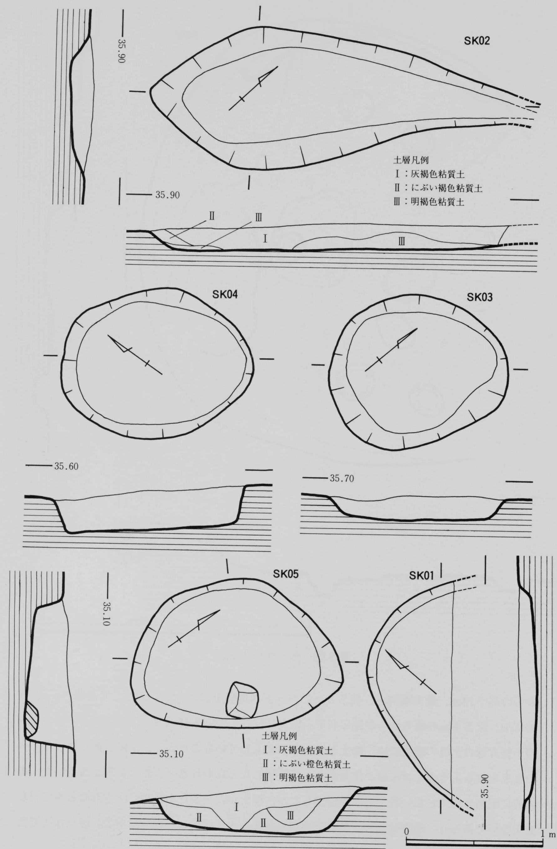
第6図 土坑実測図
