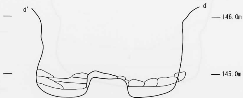
図10 d-d' 断面より間仕切り障壁見通図
