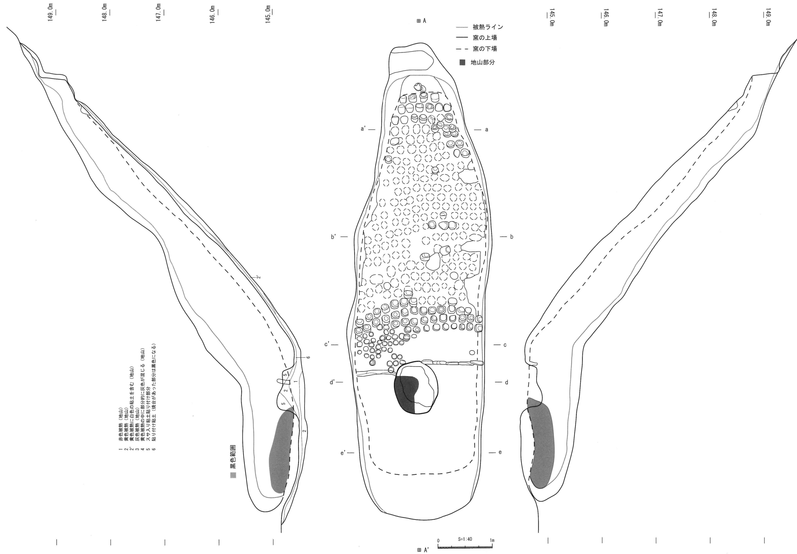
図5 窯体平面図及び立面図
