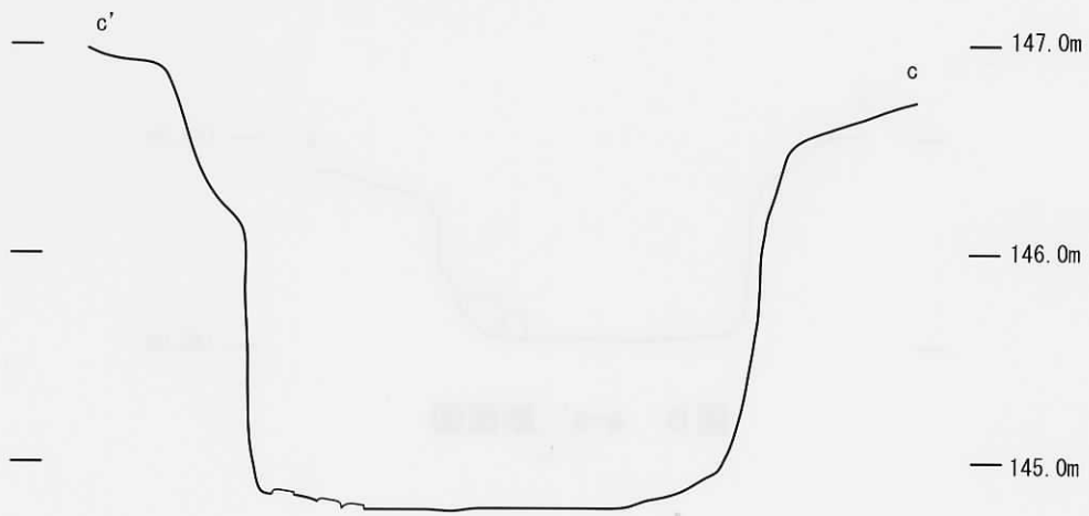
図9 c-c' 断面図
