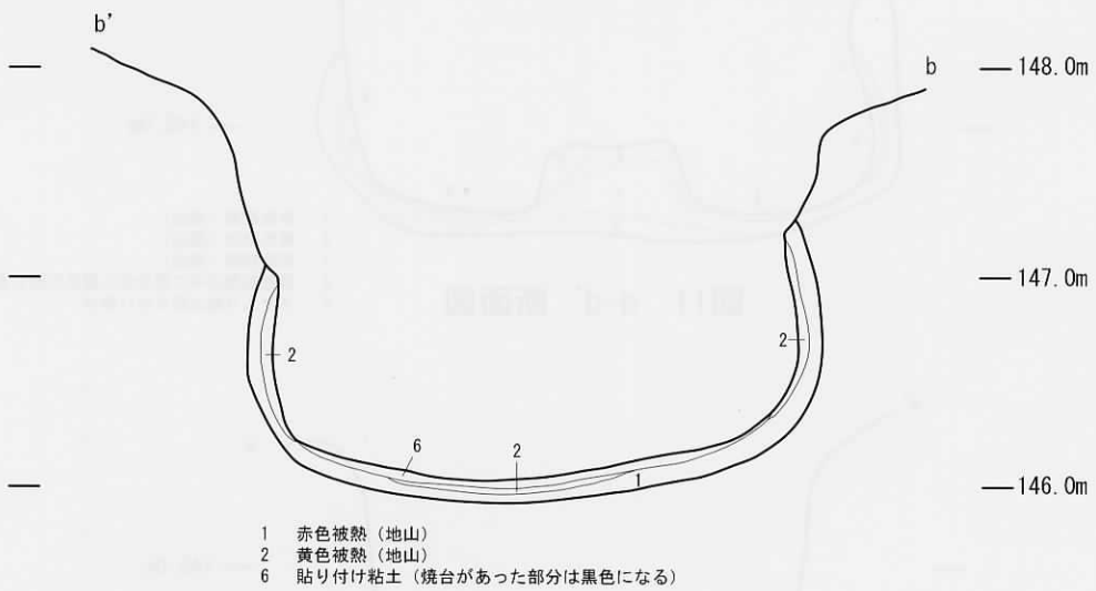
図8 b-b' 断面図
