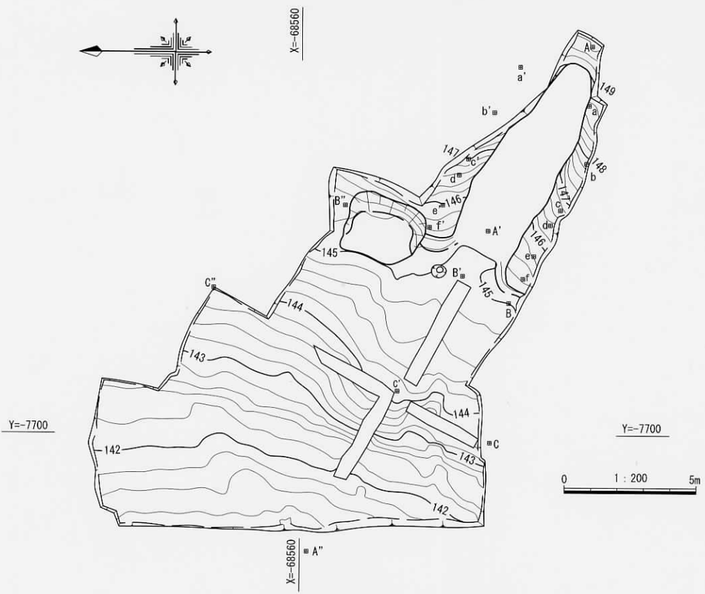
图4 大森笹洞5号古窯跡調査後地形測量図
