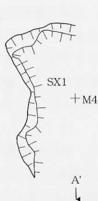
第8図 寺洞2号墳石室実測図(1)
