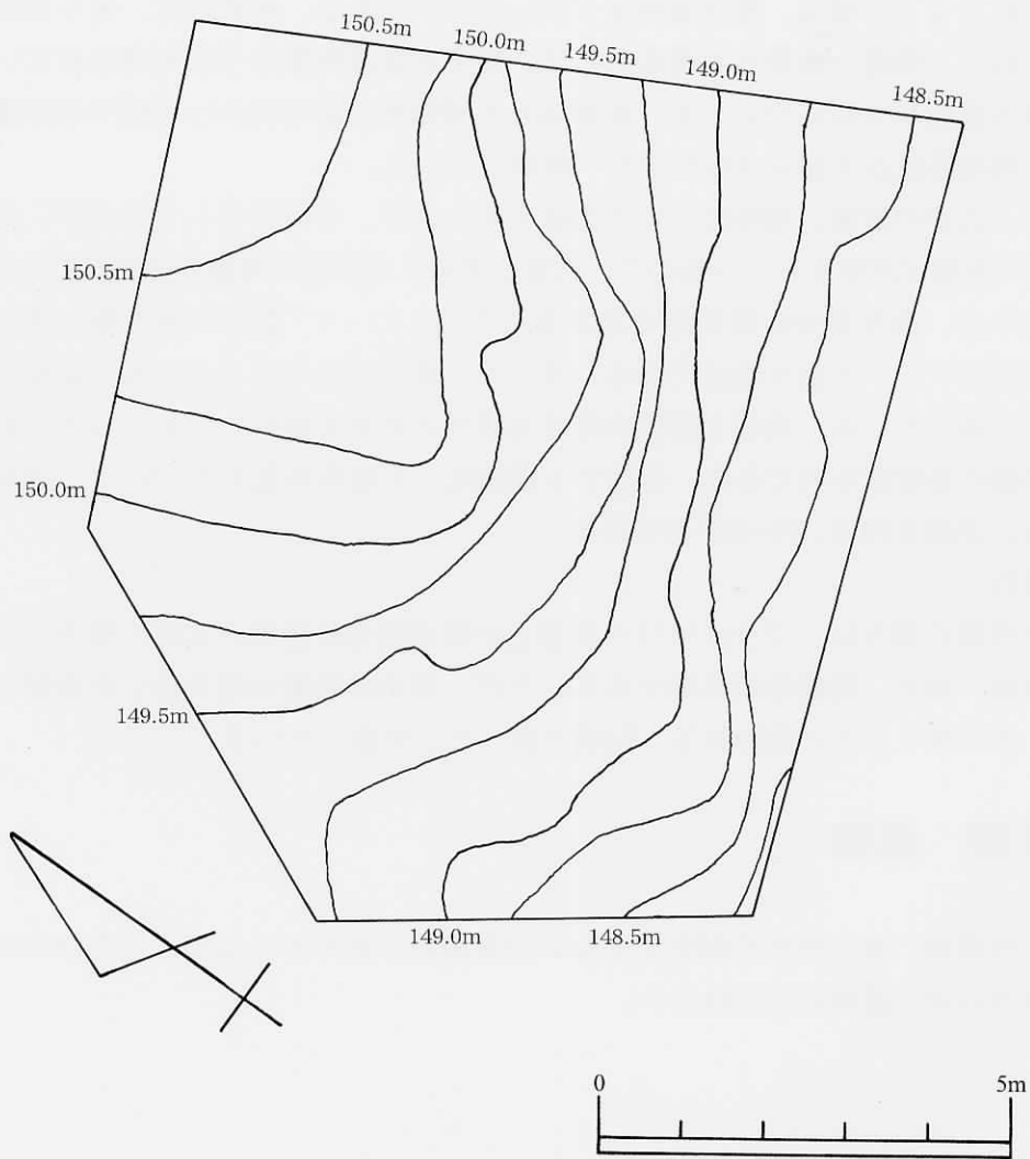
第7図 寺洞2号墳現況測量図
