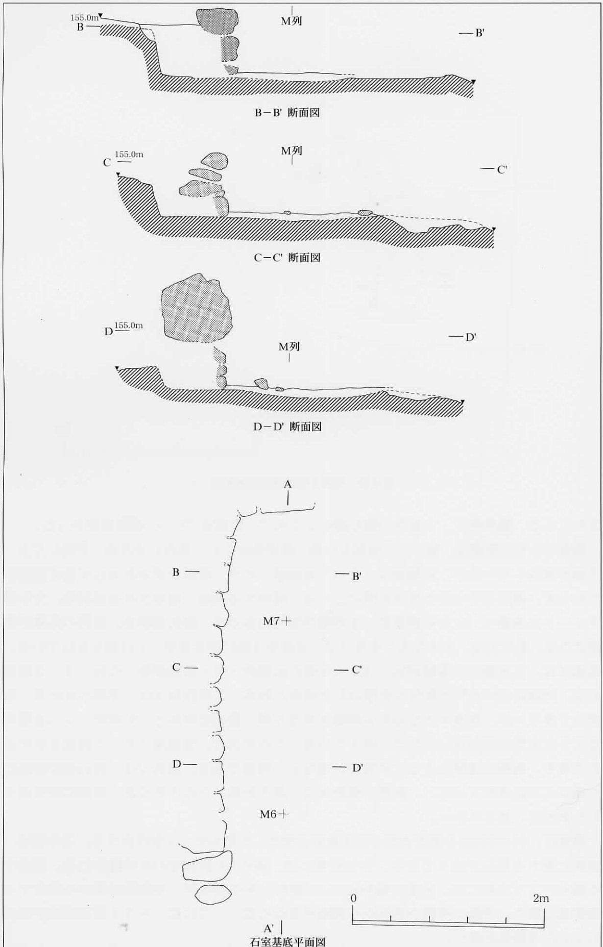
第5图 寺洞1号墳石室実測图(2)
