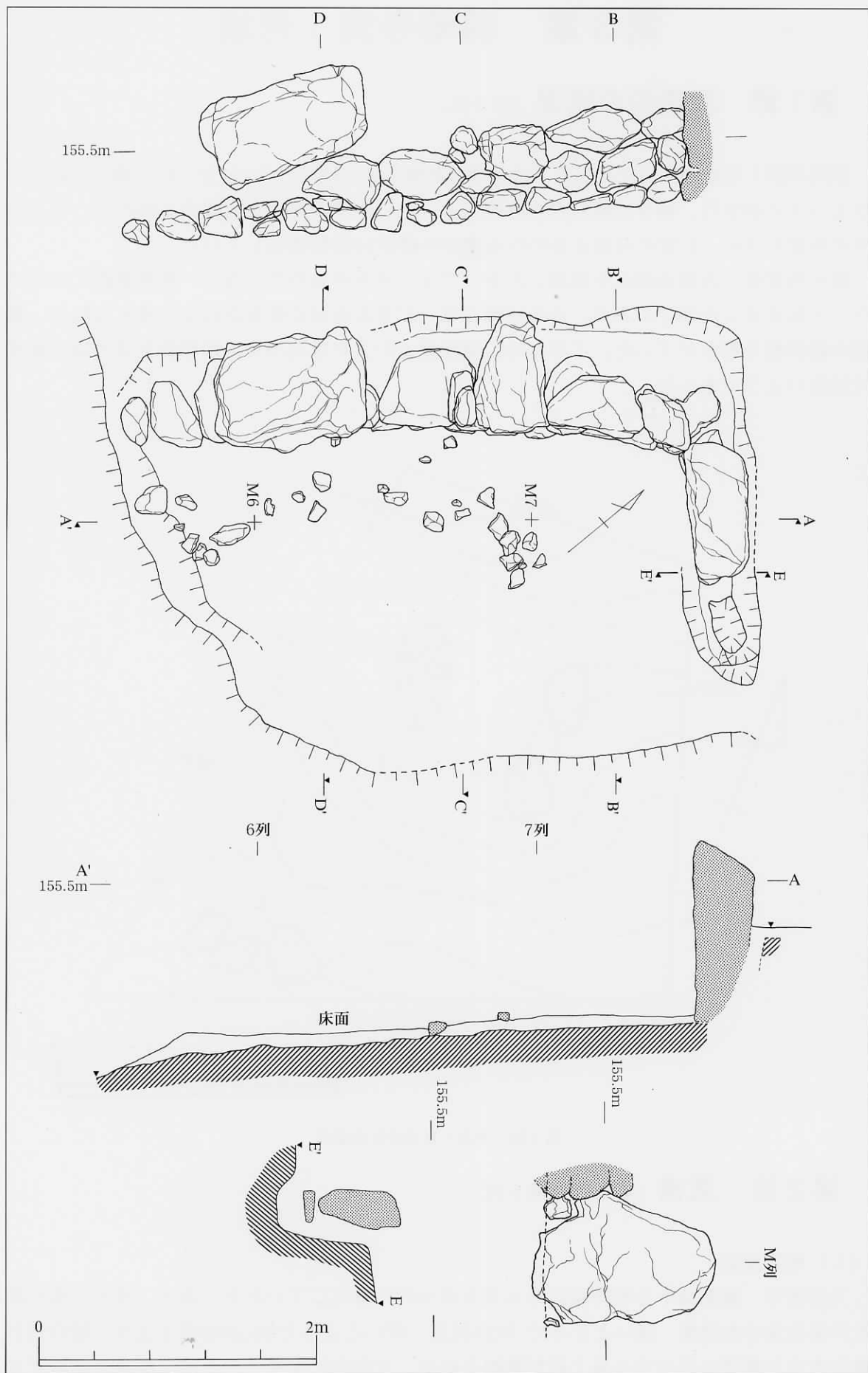
第4図 寺洞1号墳石室実測図(1)
