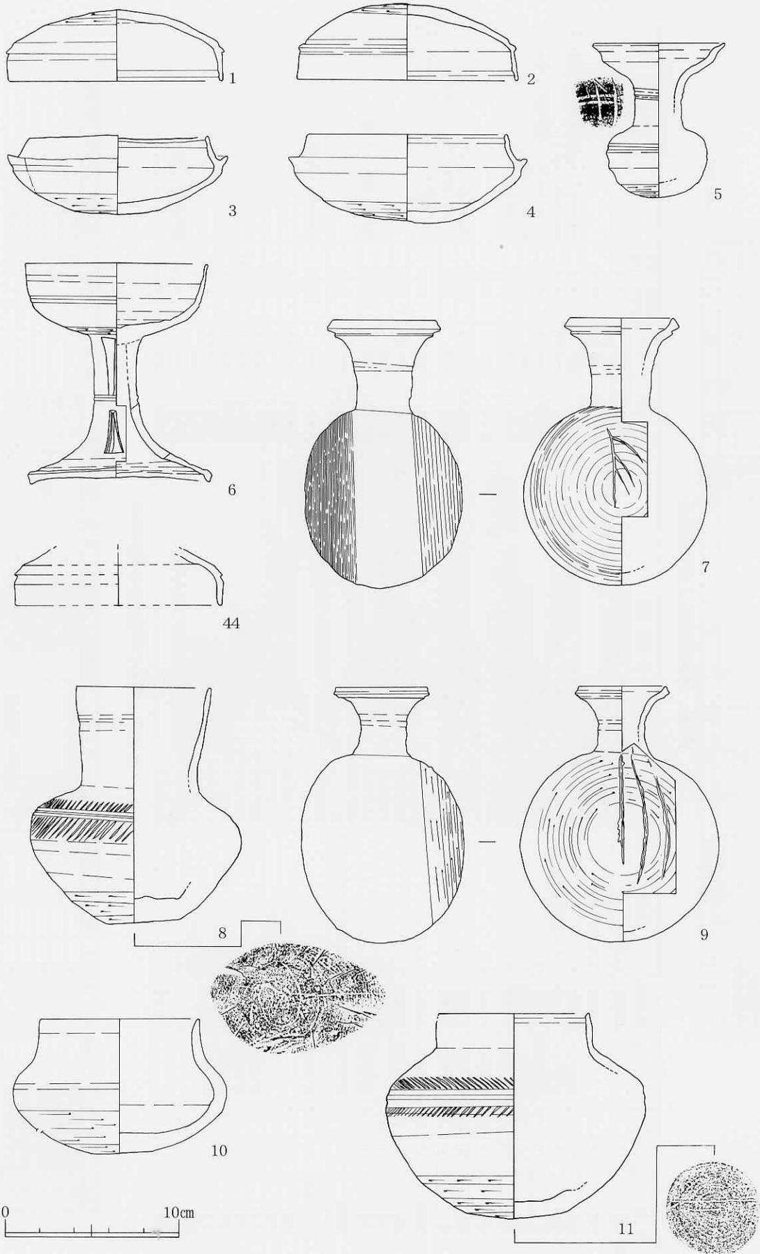
第12図 寺洞2号墳出土遺物実測図(1)
