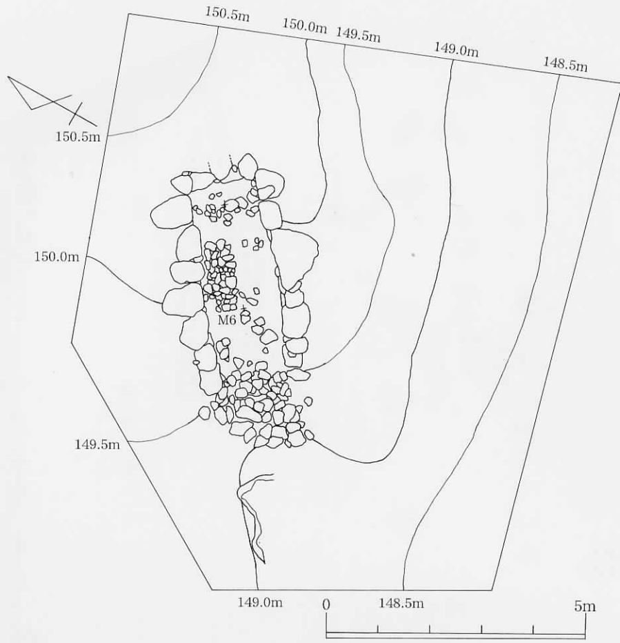
第10図 寺洞2号墳調査後測量図
