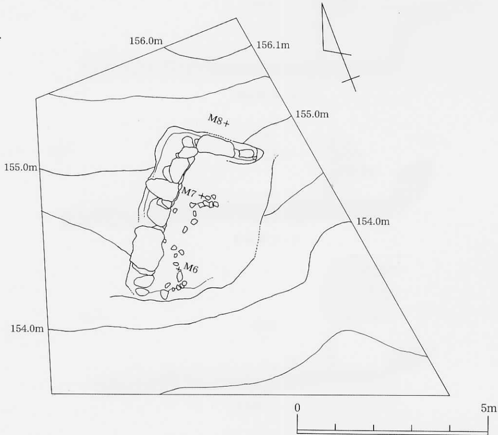
第6図 寺洞1号墳調査後測量図
