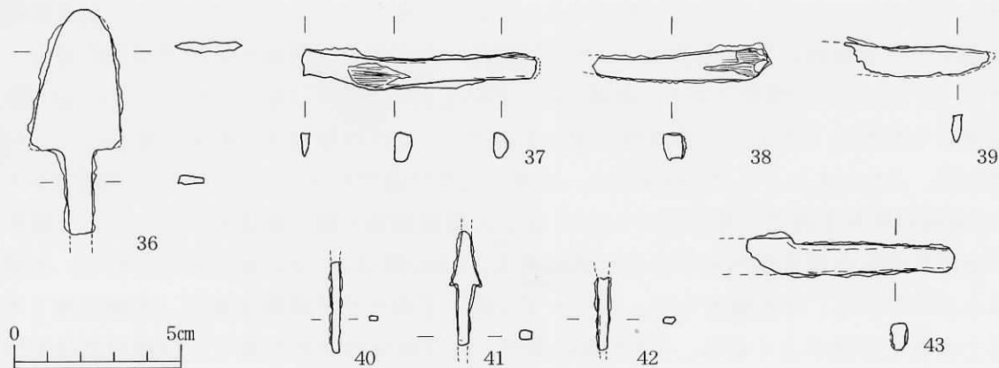
第15図 寺洞2号墳出土遺物実測図(4)
