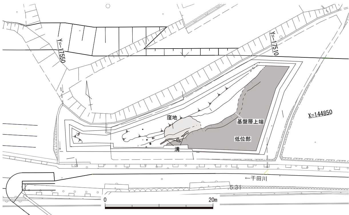
遺構配置図 (1/400)
