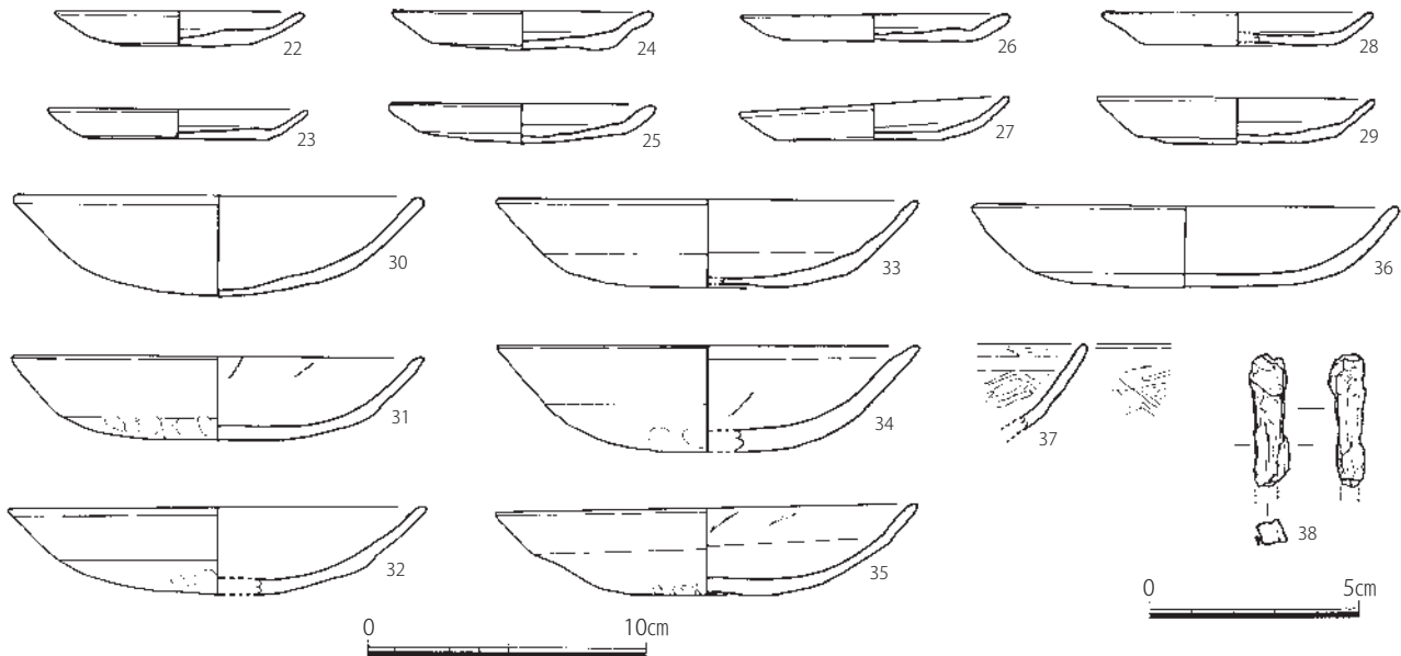
Fig. 108 253SE015 黒褐色土・暗灰色粘土出土遺物実測図 (1/3、21・38は1/2)
