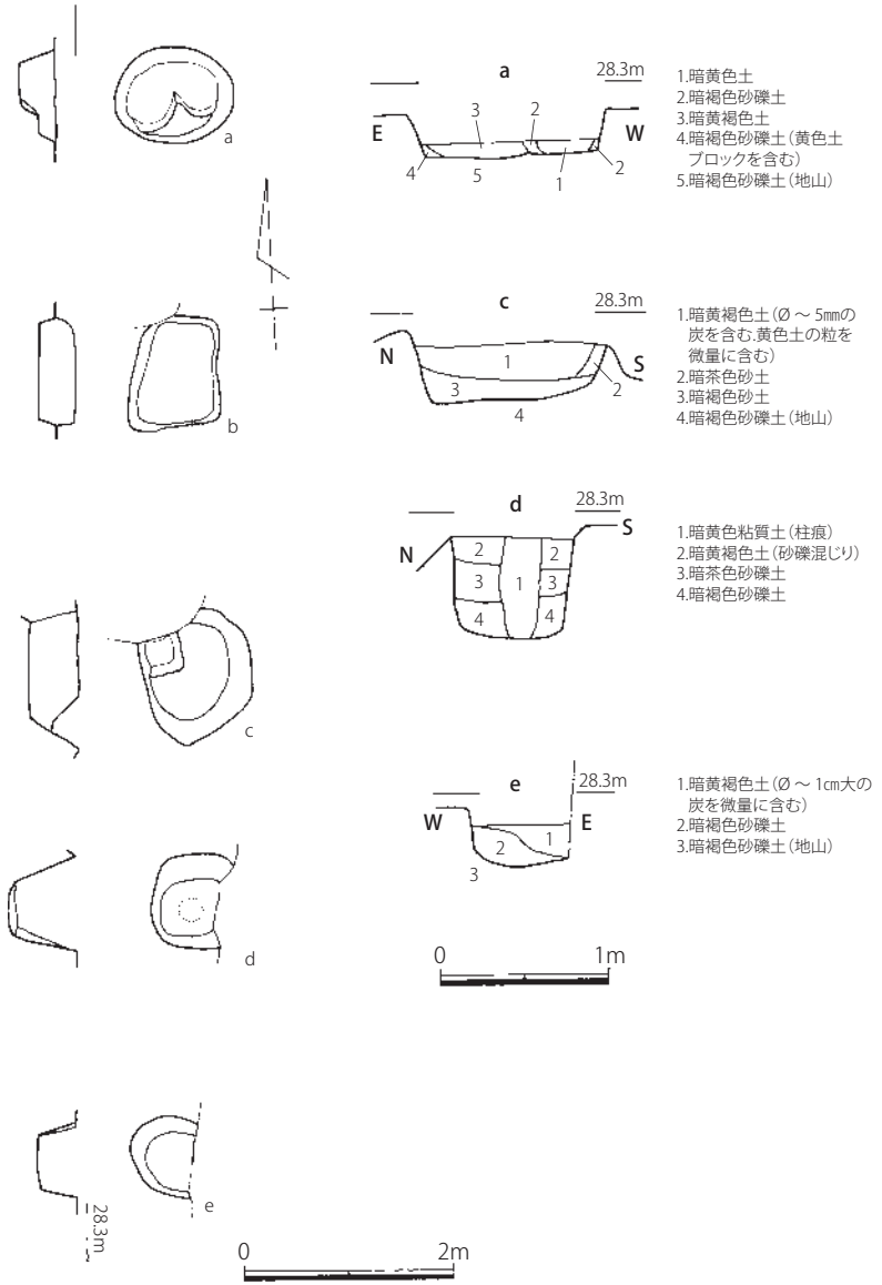
Fig. 132 322SA140 遺構実測図 (1/80、1/50)
