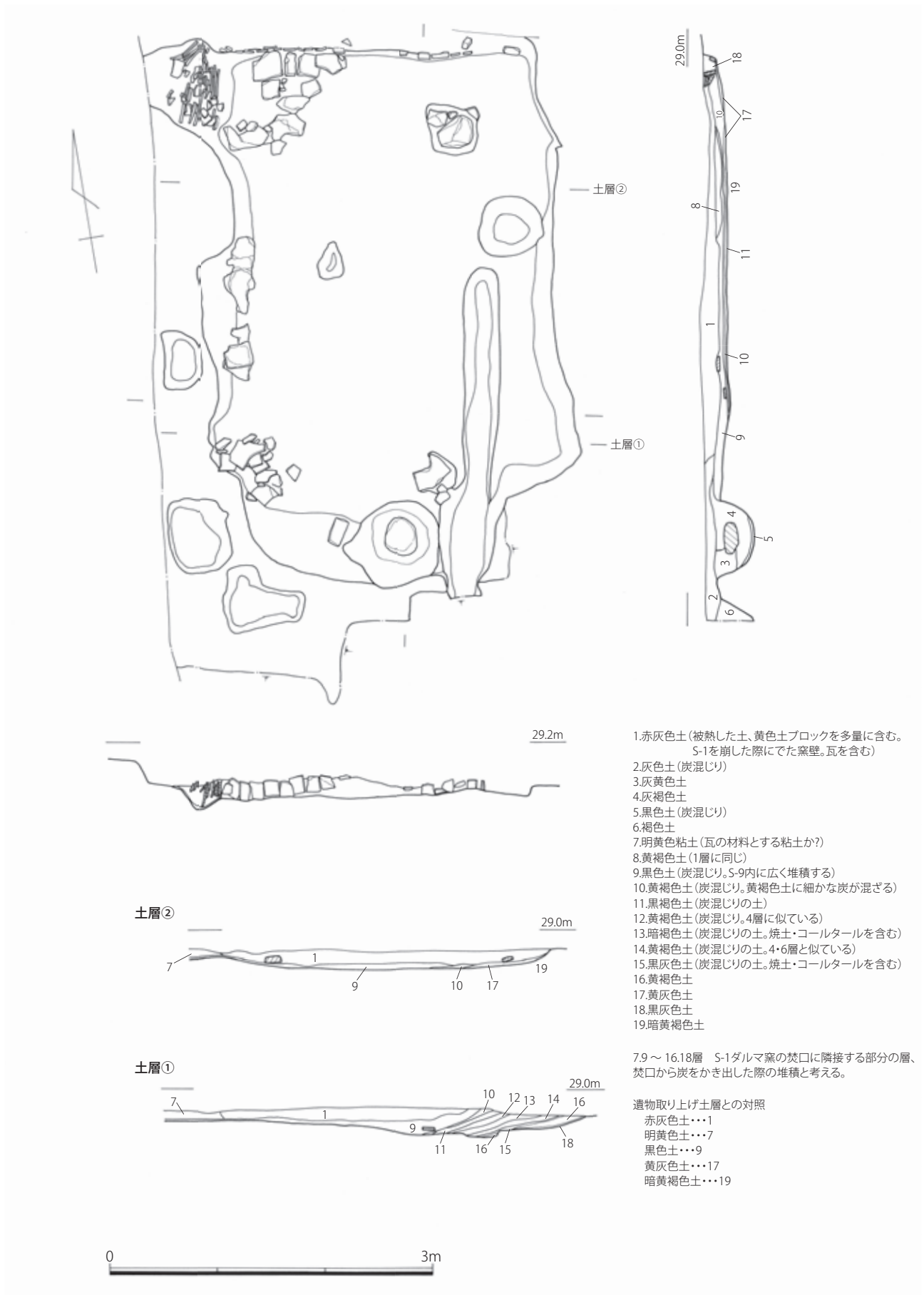
Fig. 126 322SX009 遺構実測図 (1/50)
