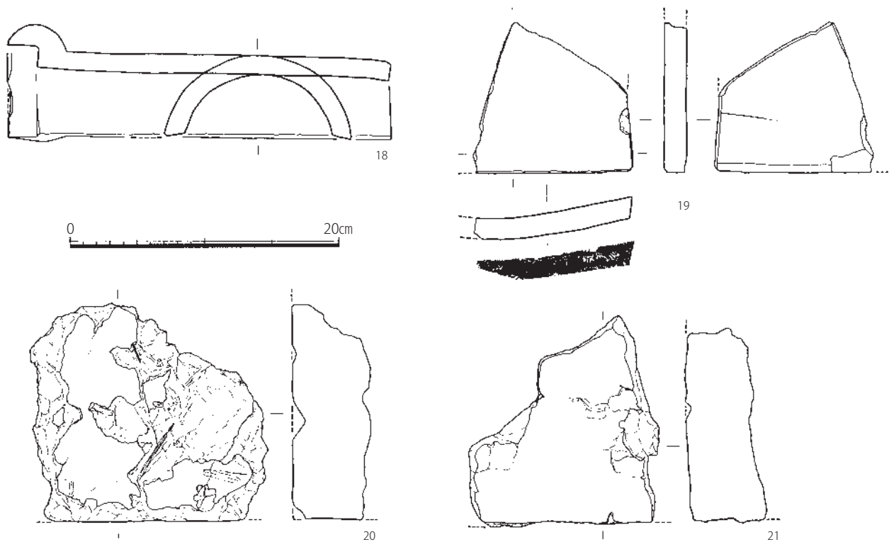
Fig. 138 322SX001・009 周辺出土遺物実測図 (1/4)
