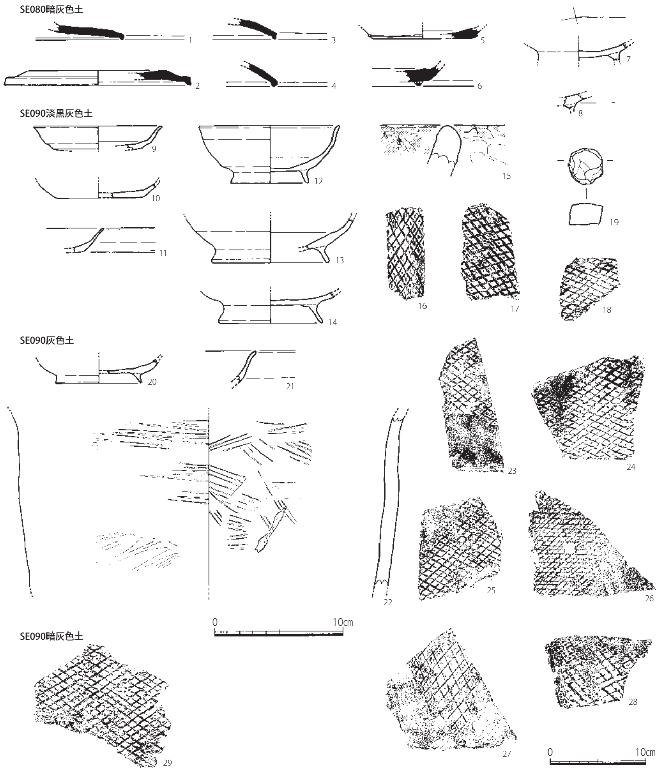
Fig. 66 175SE080・090 出土遺物実測図 (1/3、瓦は1/4)
