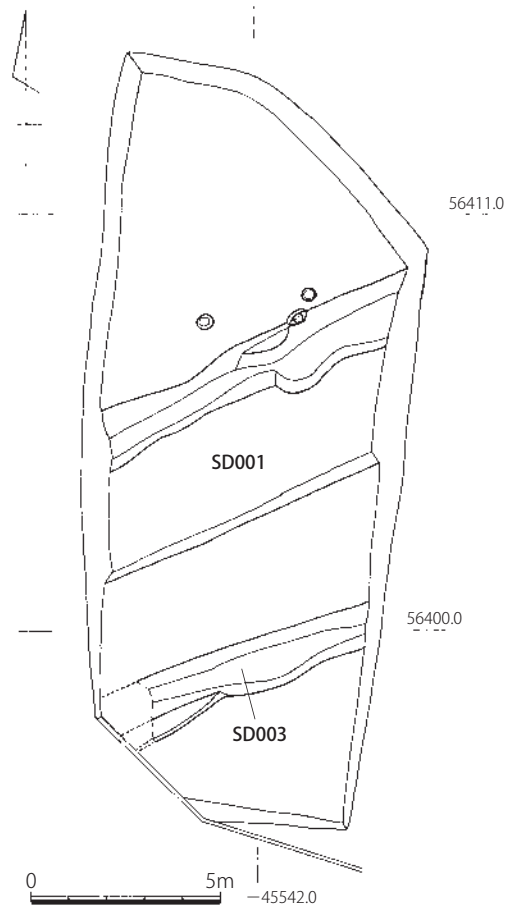
Fig. 11 第40次調査 遺構全体図 (1/200)
