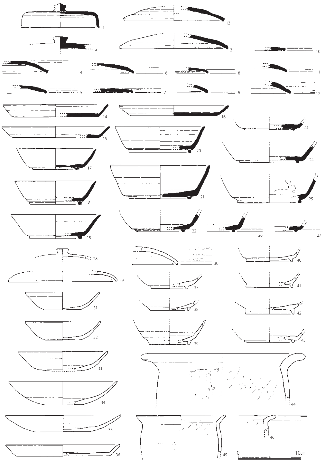
Fig. 72 175SK015 黑色土出土遺物実測図① (1/3)
