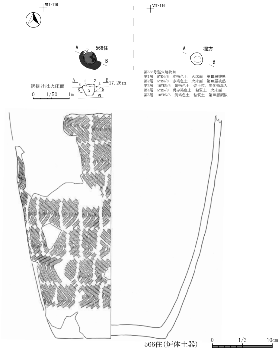
4図 第566号竪穴建物跡及び出土土器
