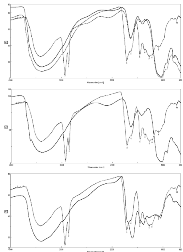
図2 土器付着物の赤外吸収スペクトル図 (番号は分析 No. を示す) (実線: 試料、点線: 生漆、数字: 生漆の赤外吸収位置)
