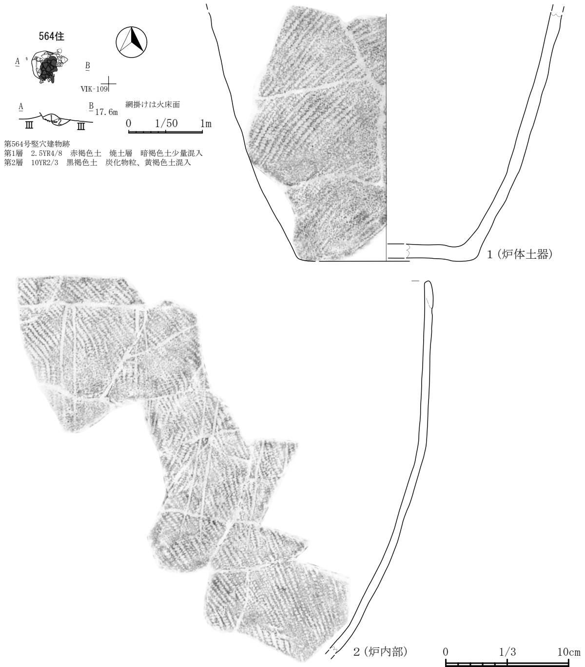
2図 第564号竪穴建物跡及び出土土器
