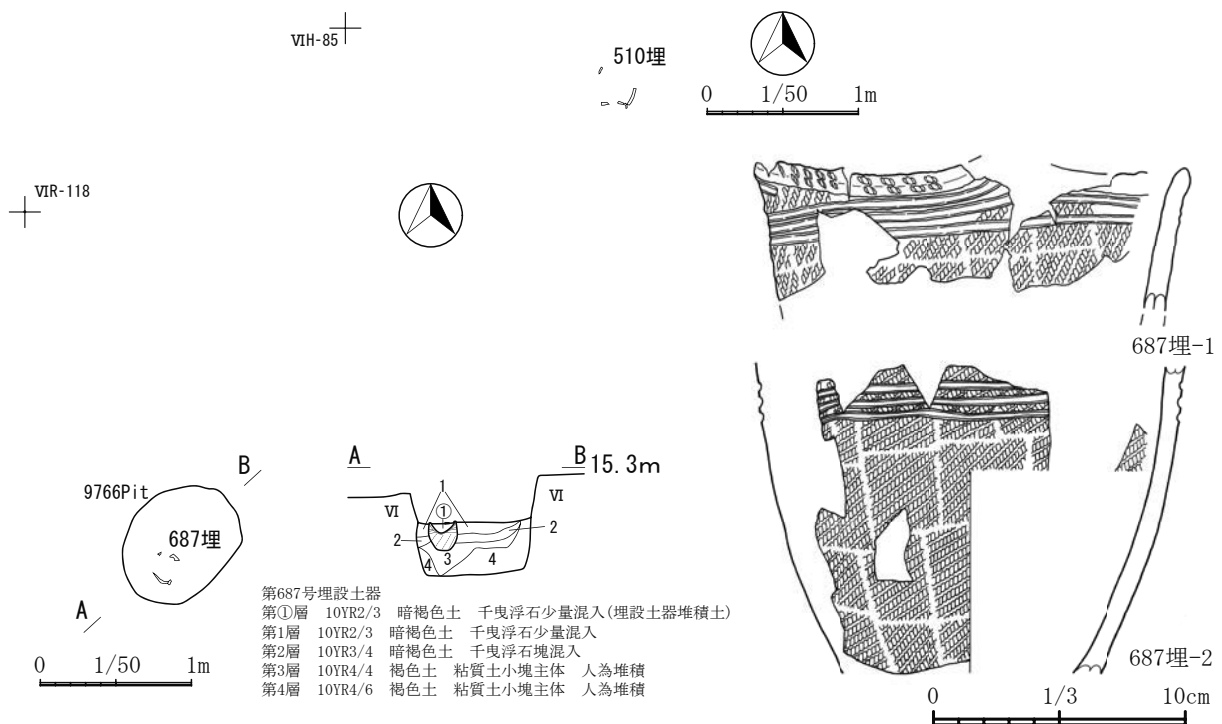
9 図 第 510・687 号埋設土器及び出土遺物
