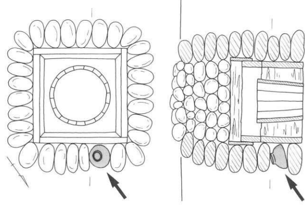
図3 金屋南遺跡 SE05 漆器椀出土状況模式図 (約1:40)
