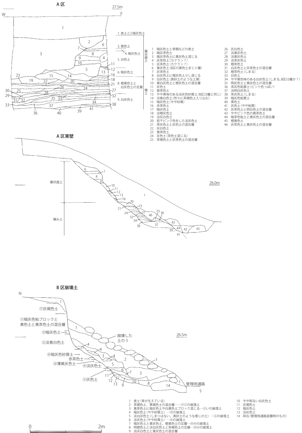
Fig. 23 第 49 次調査 A・B 土層実測図 (1/50)
