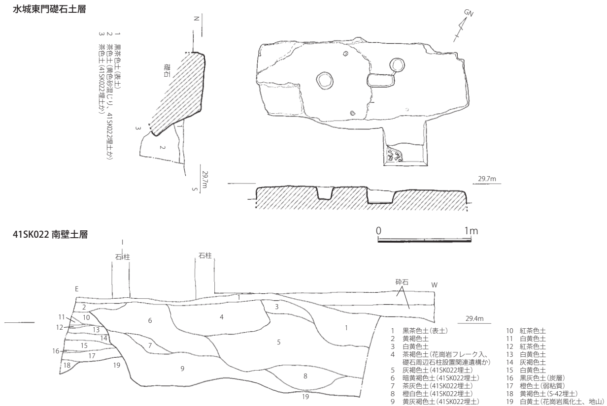
Fig. 6 水城東門礎石・41SK022 遺構実測図 (1/40)
