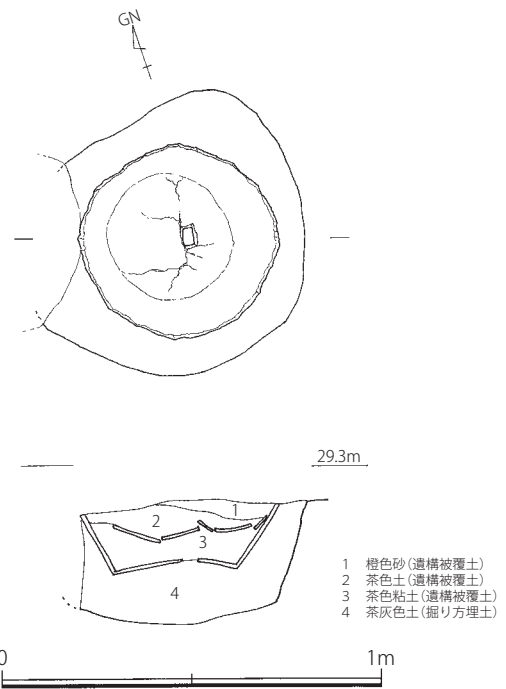
Fig. 7 41SX001・033 遺構実測図 (1/40、1/20)
