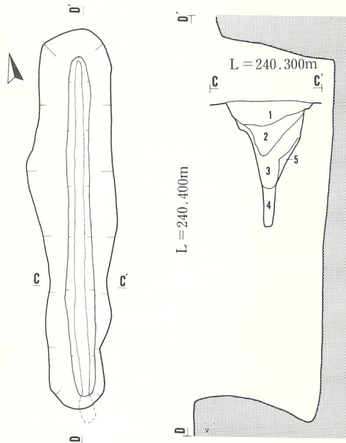
第103号陥し穴状遺構
