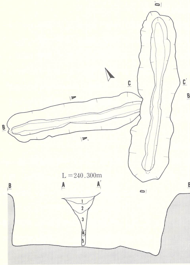
第106号 陥し穴状遺構
