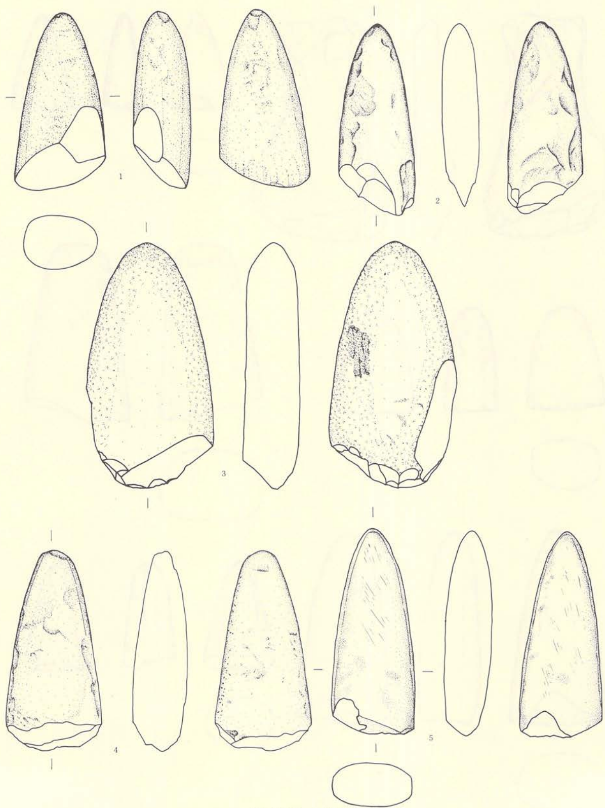
DR154 石斧 (1/2)
