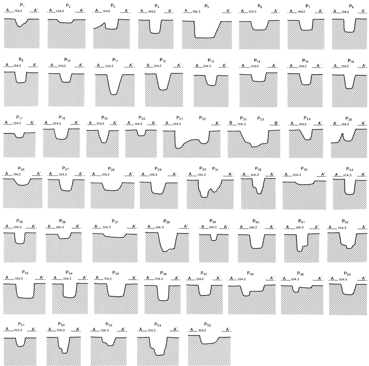
第42図 柱穴断面図
