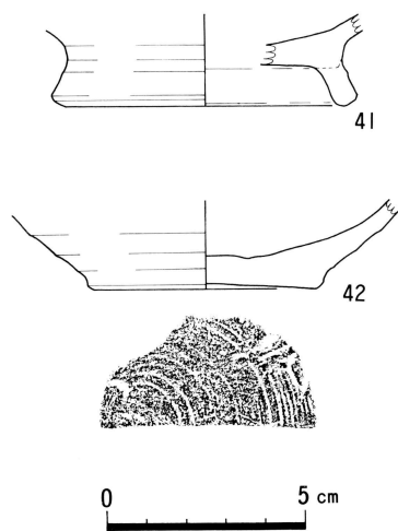
図15 土師器実測図
