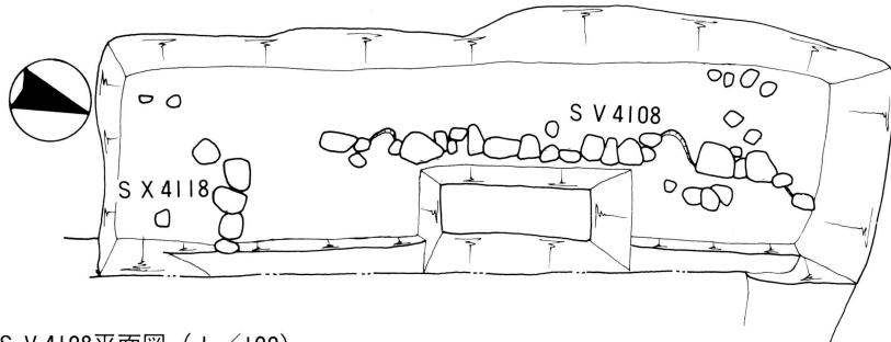
図8 S V 4108平面図 (1/100)
