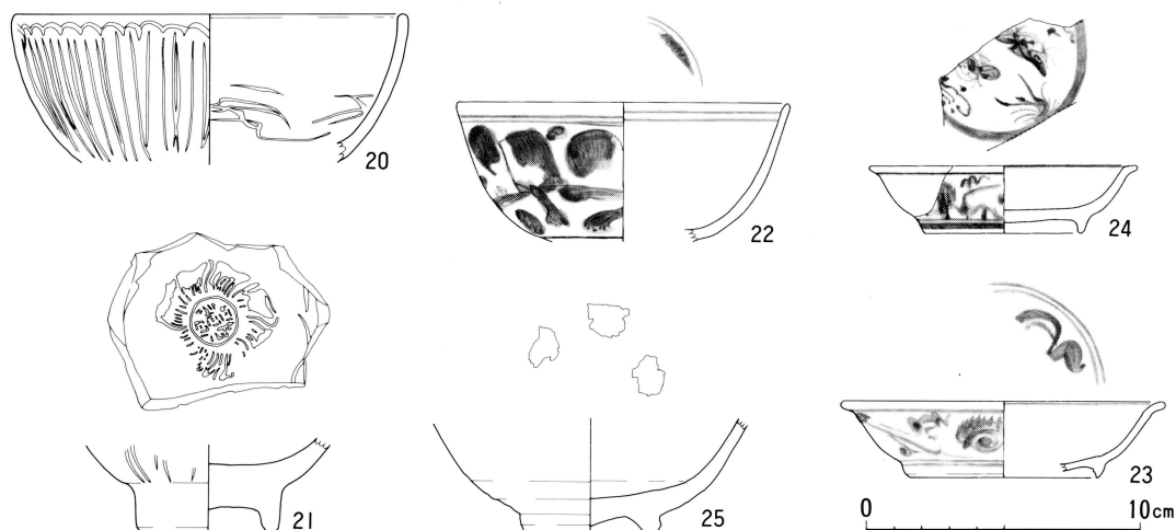
図12 輸入陶磁器実測図
