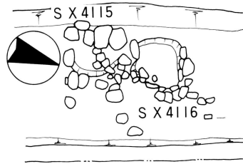
図5 S X4115・4116平面図 (1/100)
