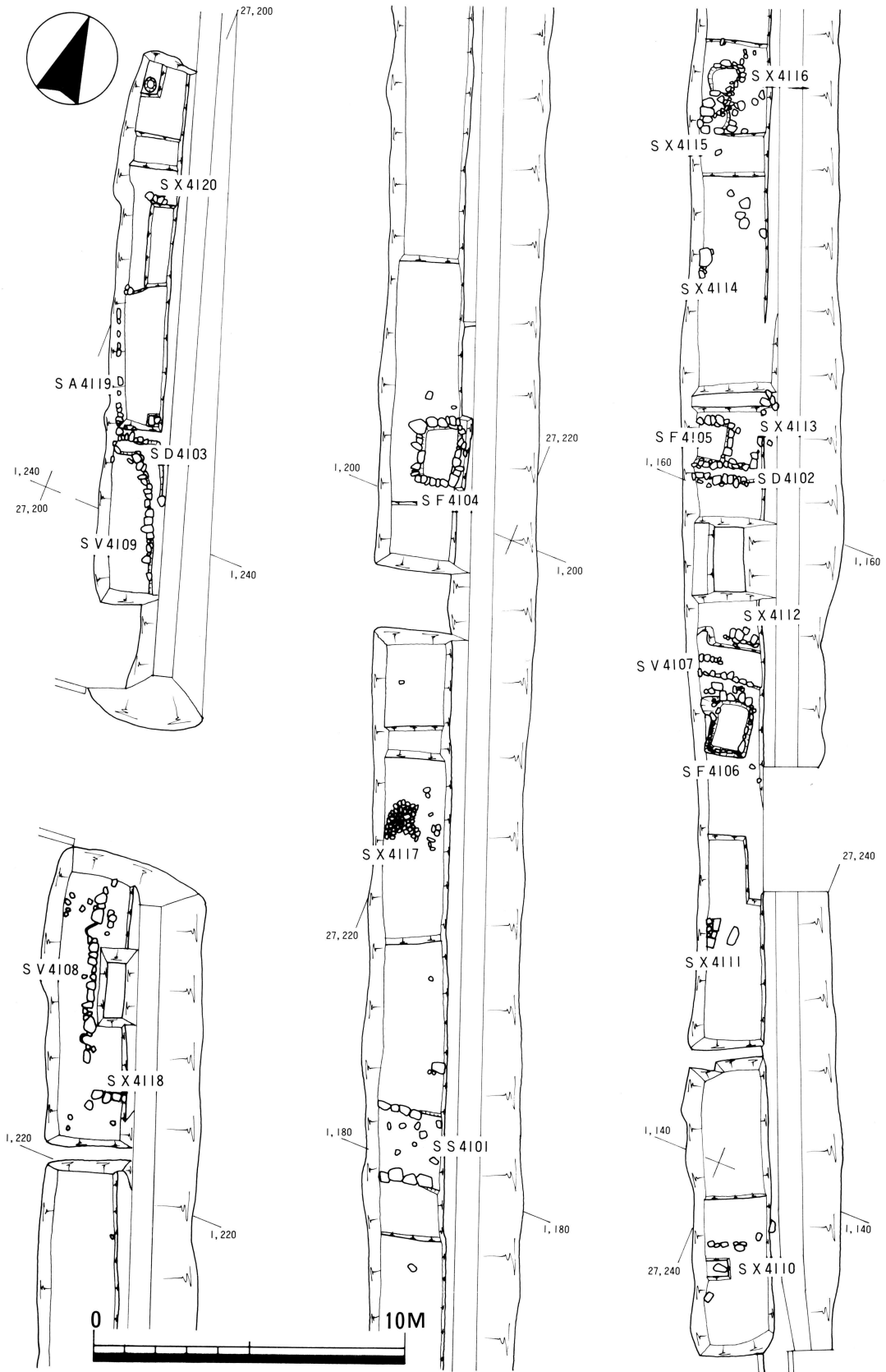
図4 第76次調査区全測図 (1/200)
