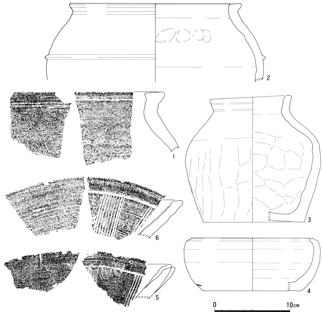
图10 越前烧实测图
