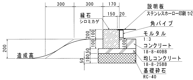
第17図 説明板(炉跡) 詳細図
