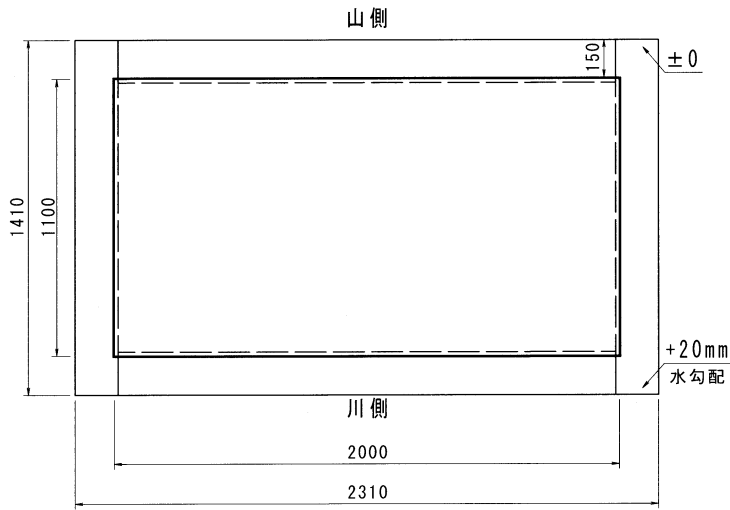
平面図 S=1/30
