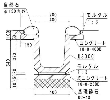
河川縦溝 S=1/20
