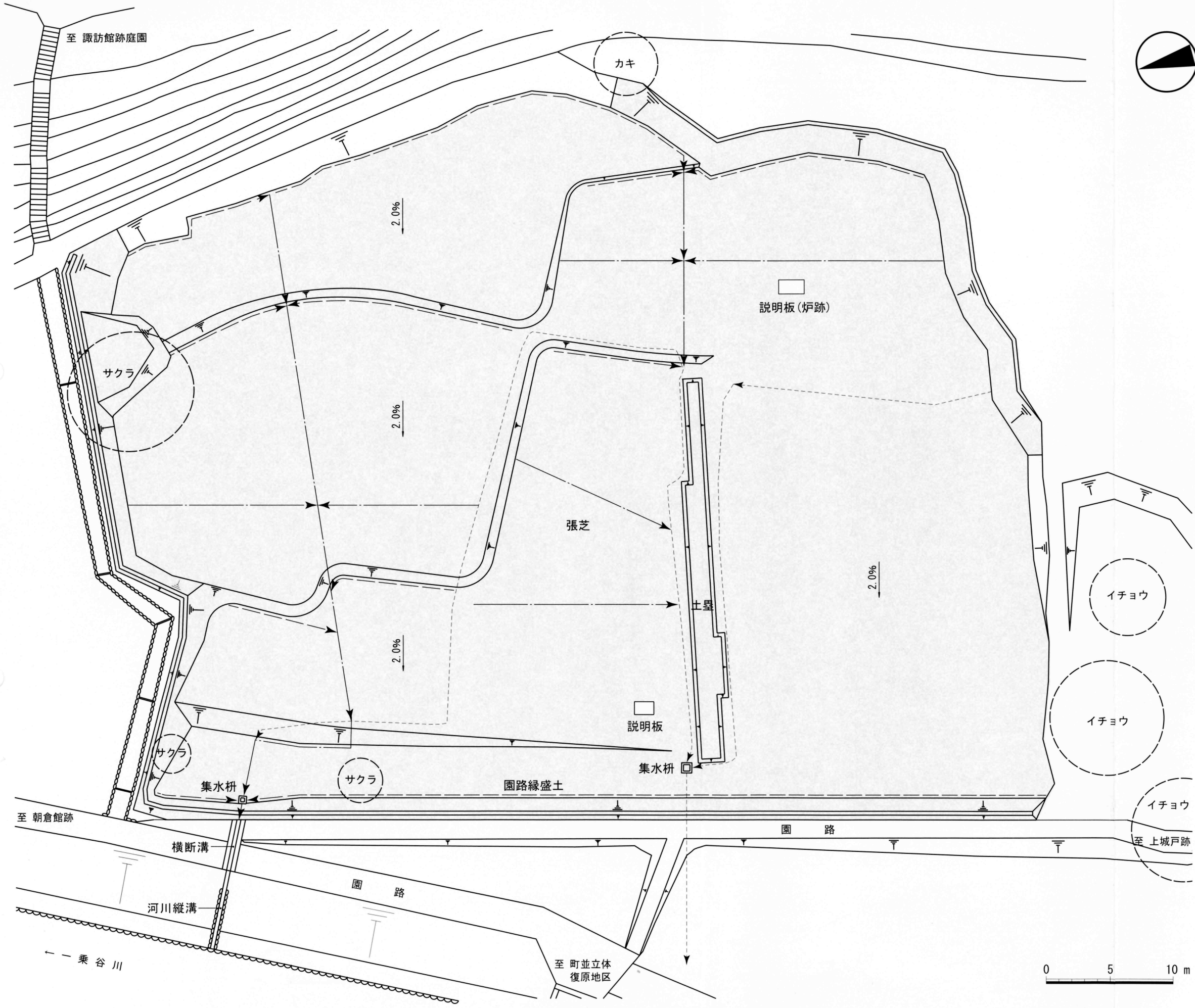
第16図 第124次調査区(米津)整備工事平面図(S=1/300)
