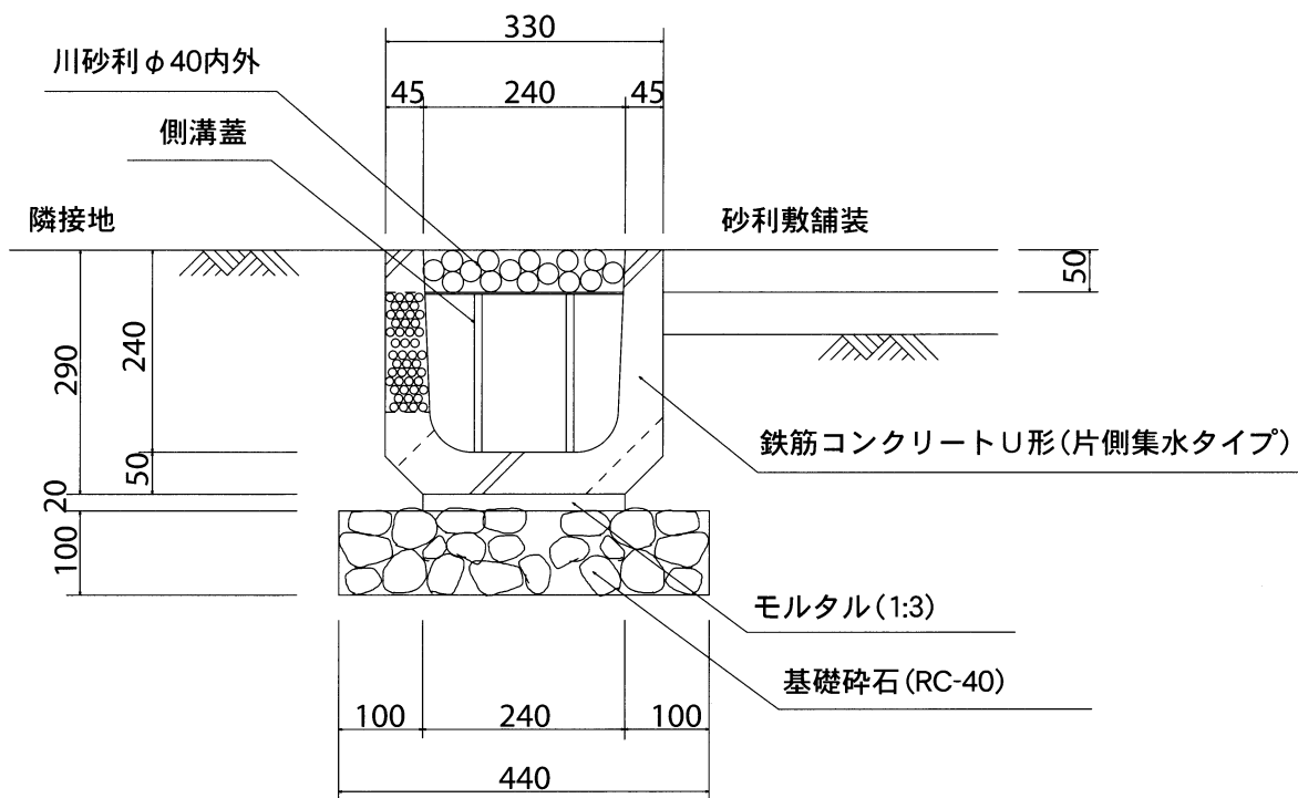
挿図11 片側透水側溝断面図 (S=1/10)
