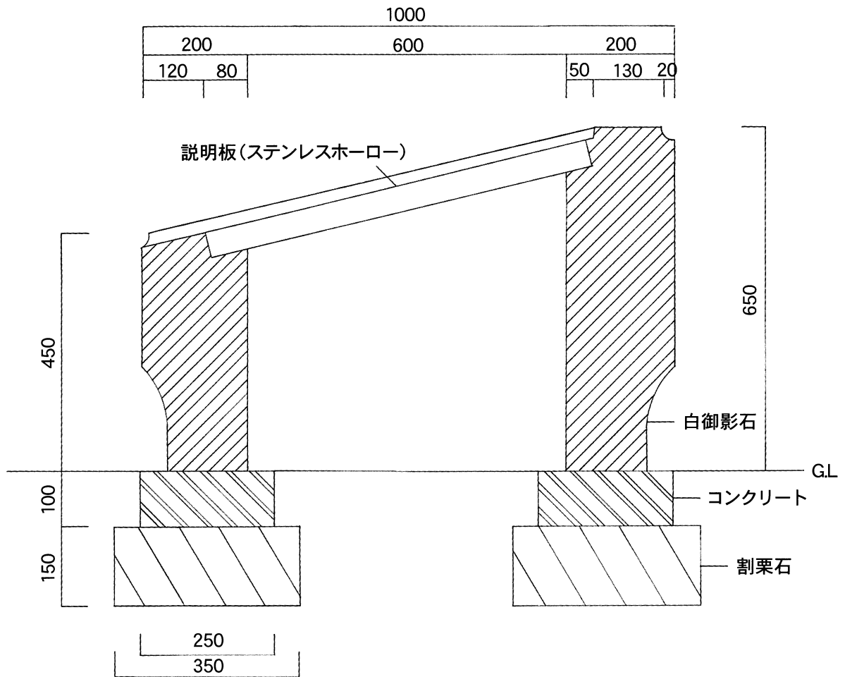
挿図12 説明板断面図 (S=1/10)
