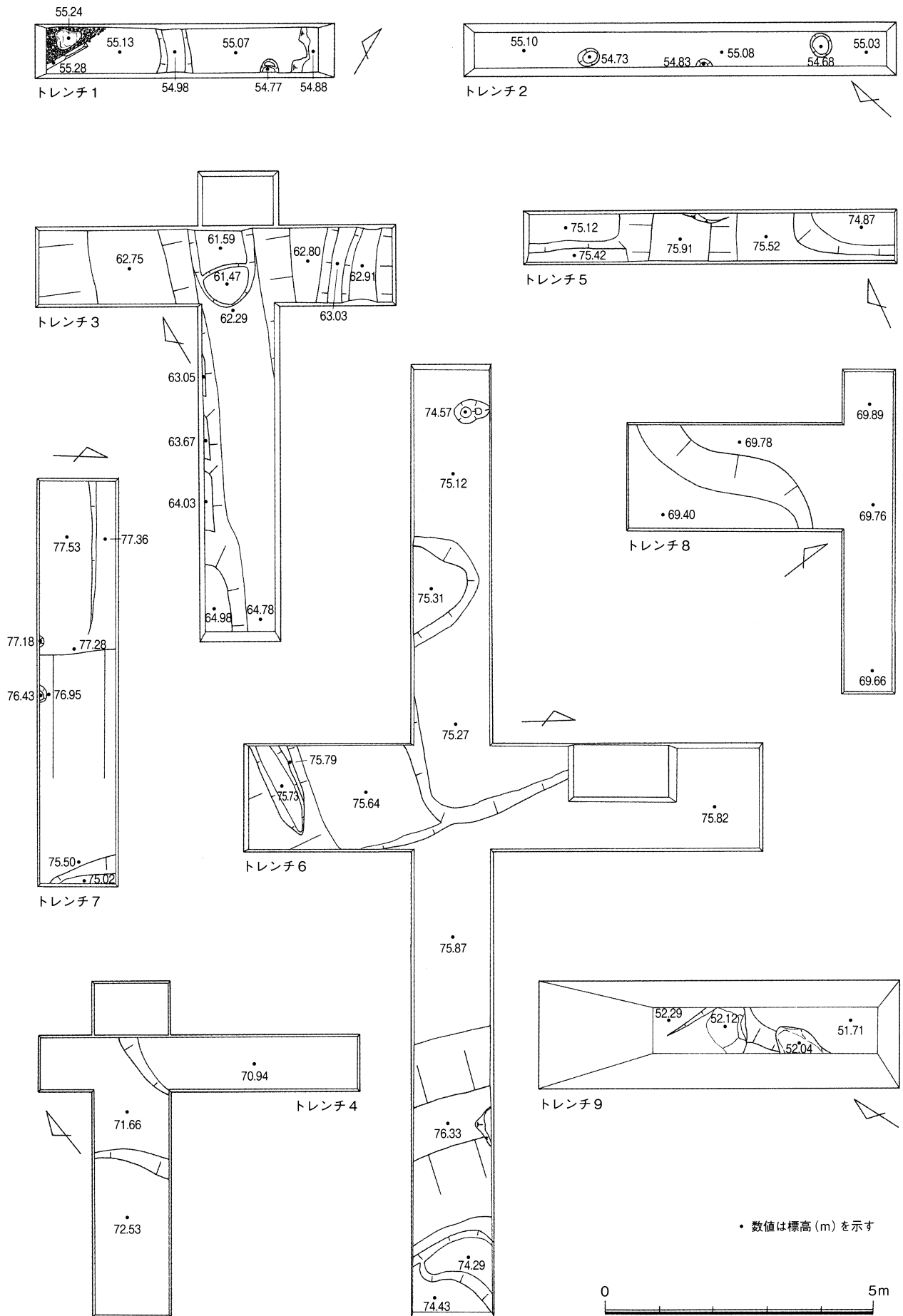
第15図 月見槽地区試掘調査遺構平面図 (S=1/100)
