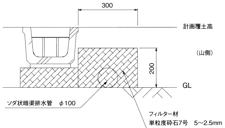
第19図 暗渠排水管 S=1/10
