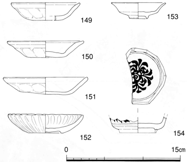
挿図2 SK5874 出土遺物実測図
