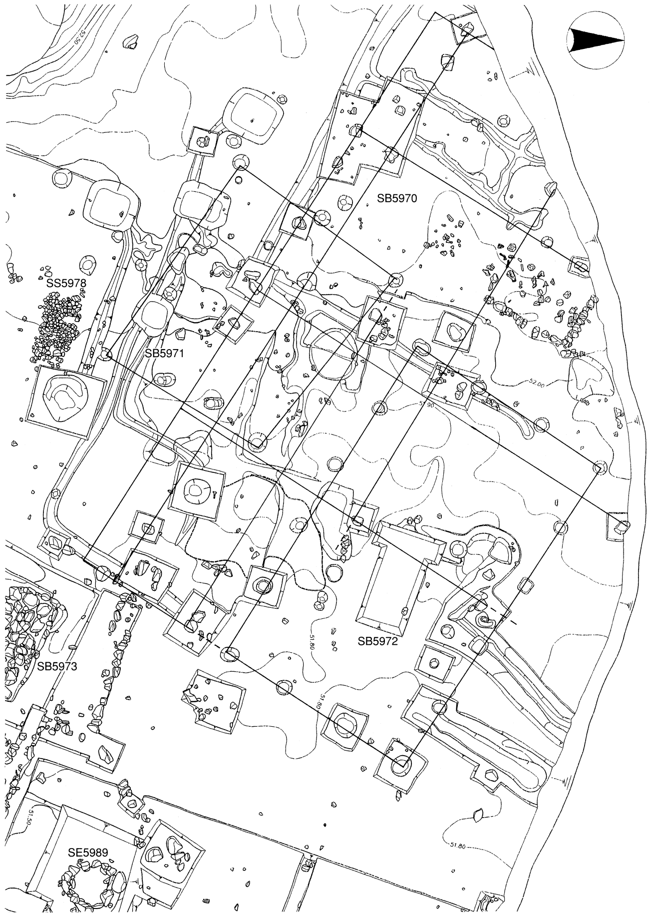
第5図 SB5970・5971・5972詳細図 (S=1/100)
