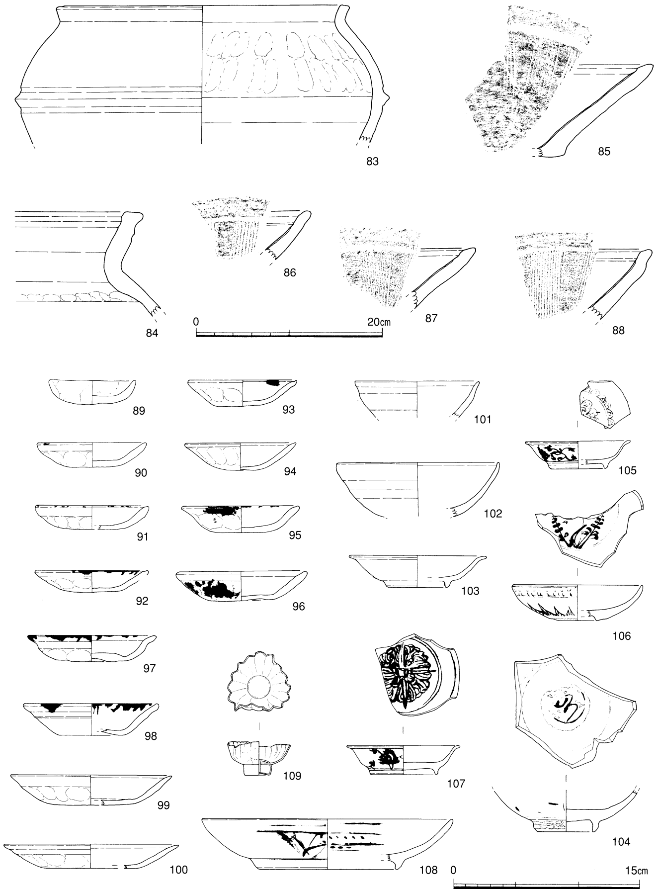
第11図 第118次調査出土遺物 (5)
