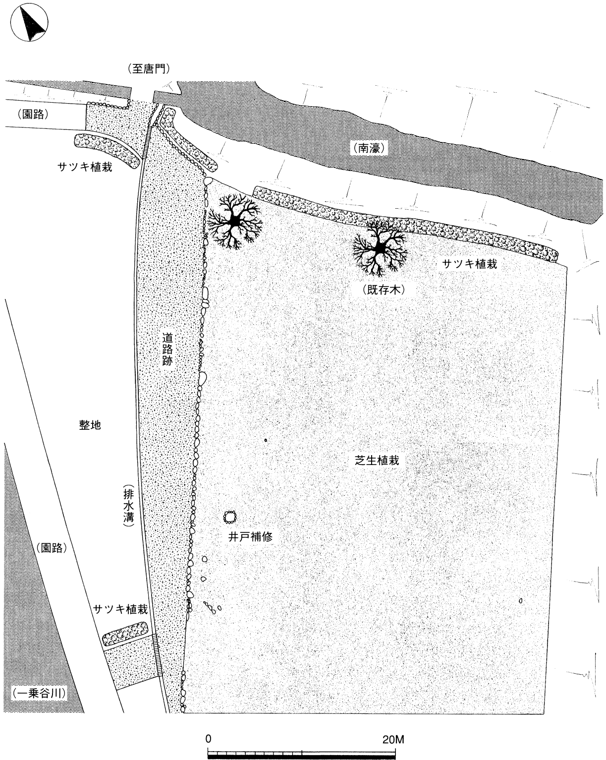
第14図 第109次調査区新御殿整備全体図 (1/400)
