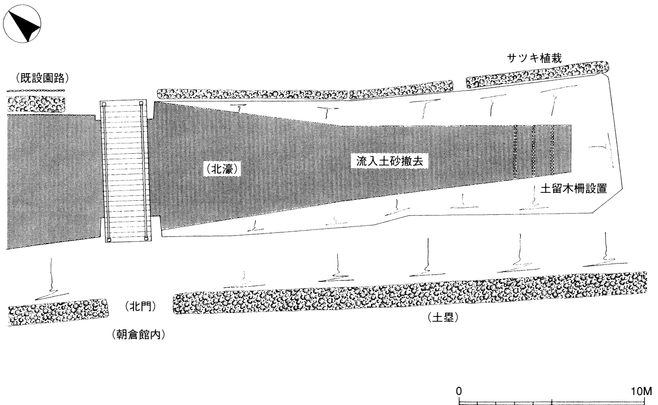
第16図 朝倉館北濠復旧整備図 (1/200)
