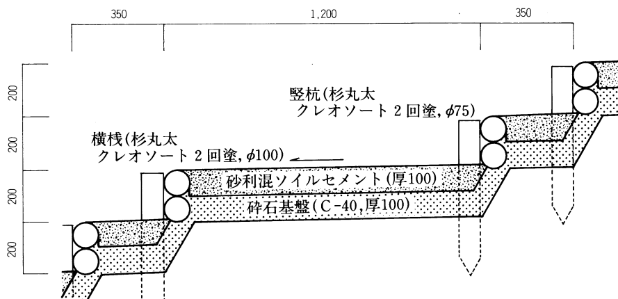
第23図 登り階段 (断面詳細図 1/20)
