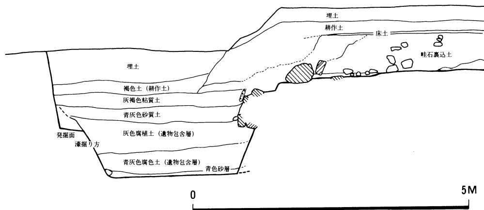
第 6 図 濠 S D 2261 土層断面図
