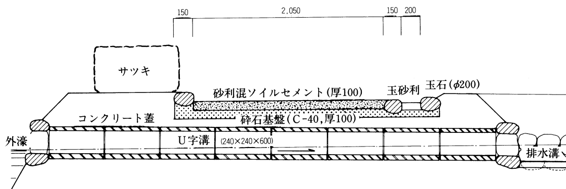
第21図 園路・暗渠(断面詳細図 1/40)
