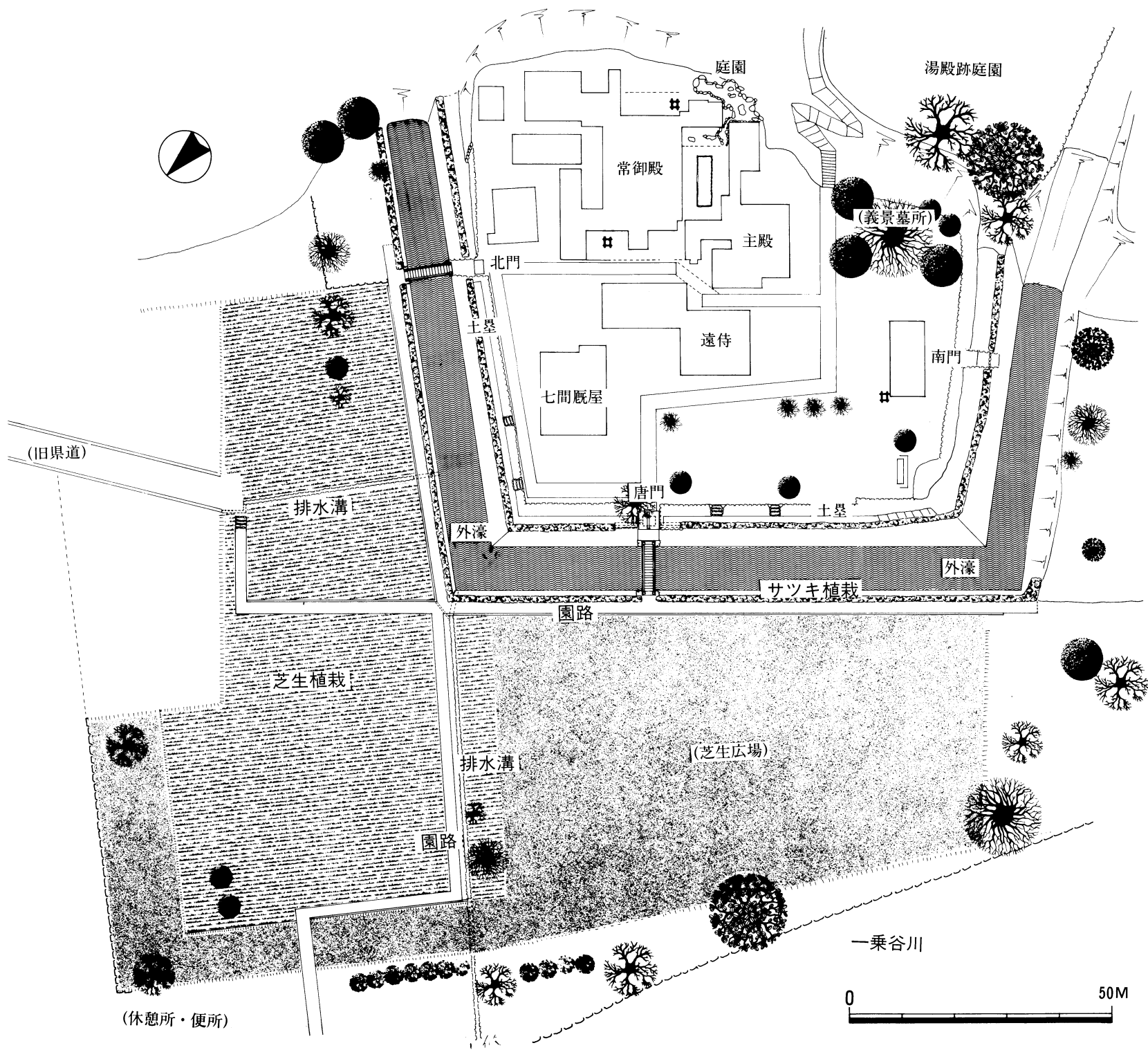
第22図 朝倉館外郭修景工全体図 (1/1000)
