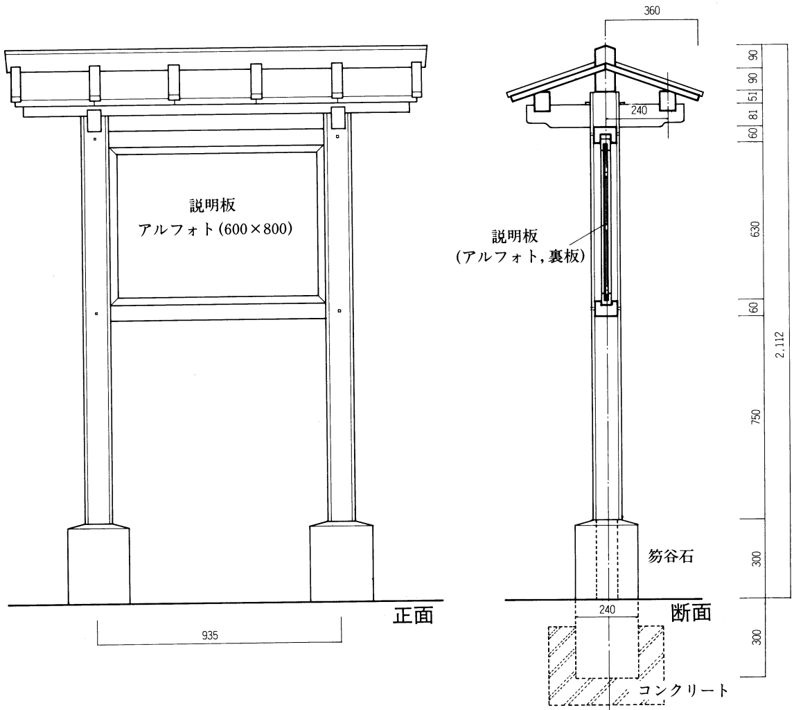
第20図 木製説明板詳細図 (1/20)
