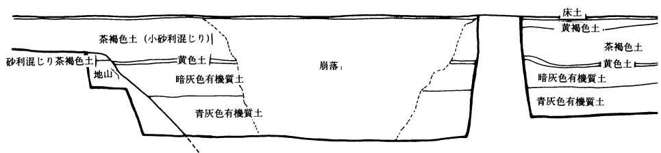
第3図 S D 2255濠土層断面図
