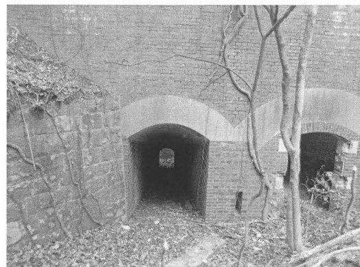
横墻の砲側庫と隧道
