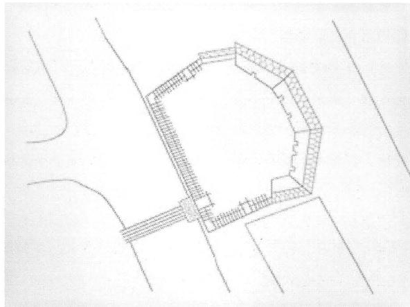
炬口台場 平面図
