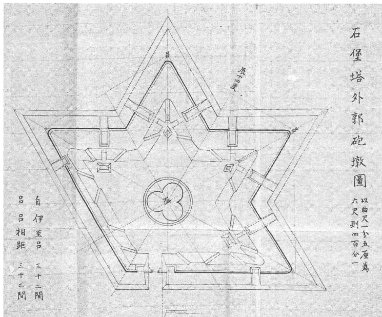
「(和田岬)石堡塔外郭砲墩圖」
