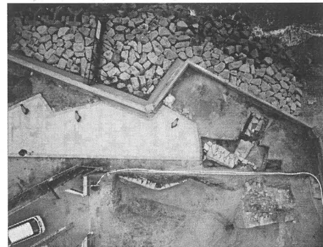
第1・2次調査垂直空中写真
