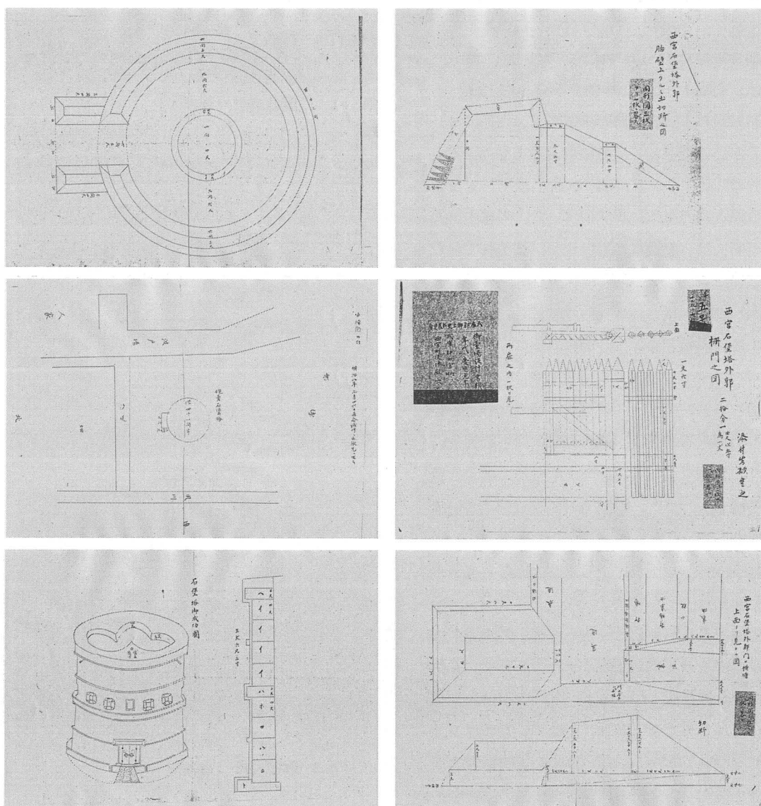
西宮砲台図面（写）
