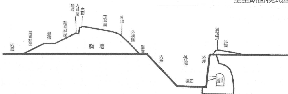
堡壘断面模式图
