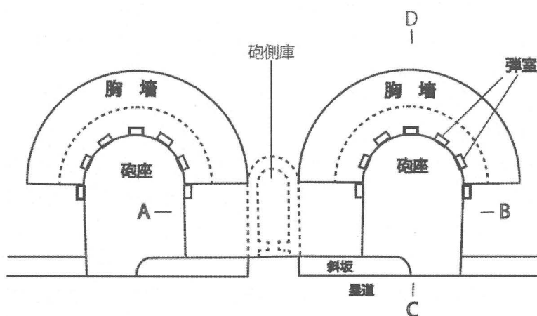
砲座平面模式图
