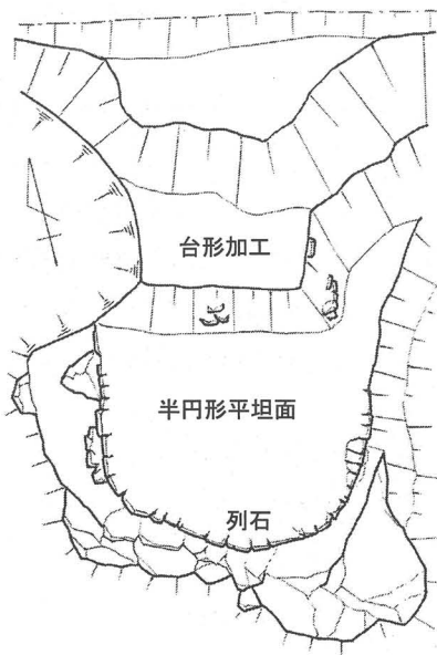
室津1号(左)、2号(右)台場平面図
