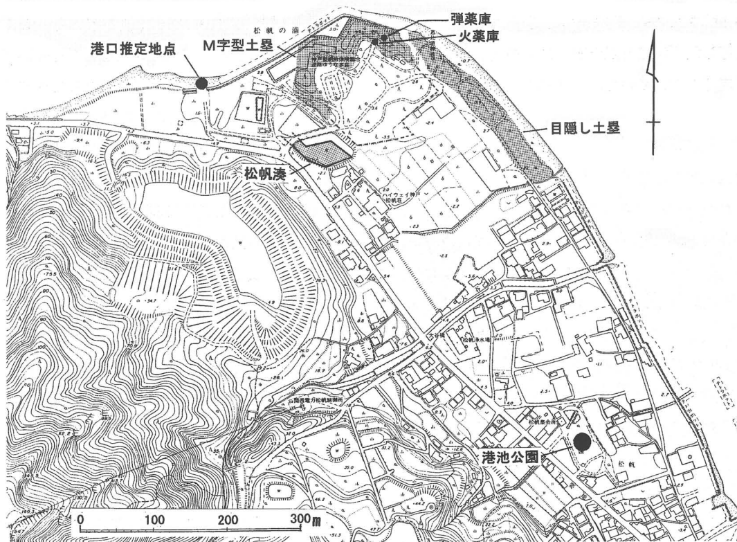
松帆台場主要遺構配置図
