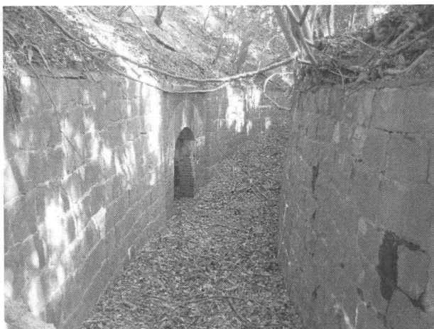
隧道出口部の外濠
