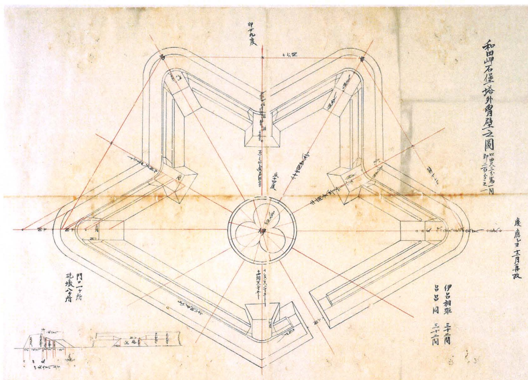
「和田岬石堡塔外胄壁之圖」慶應元年十二月再改 (神戸市立博物館蔵)
