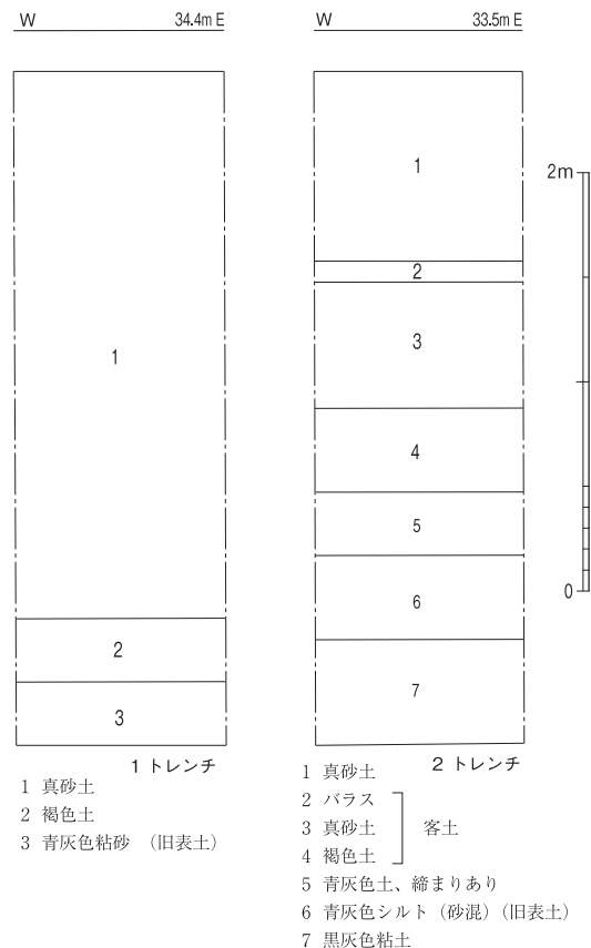
Fig.7 第 248 次調査土層略測図 (1/40)
