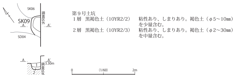
第24図 第9号土坑実測図 (SK09)
