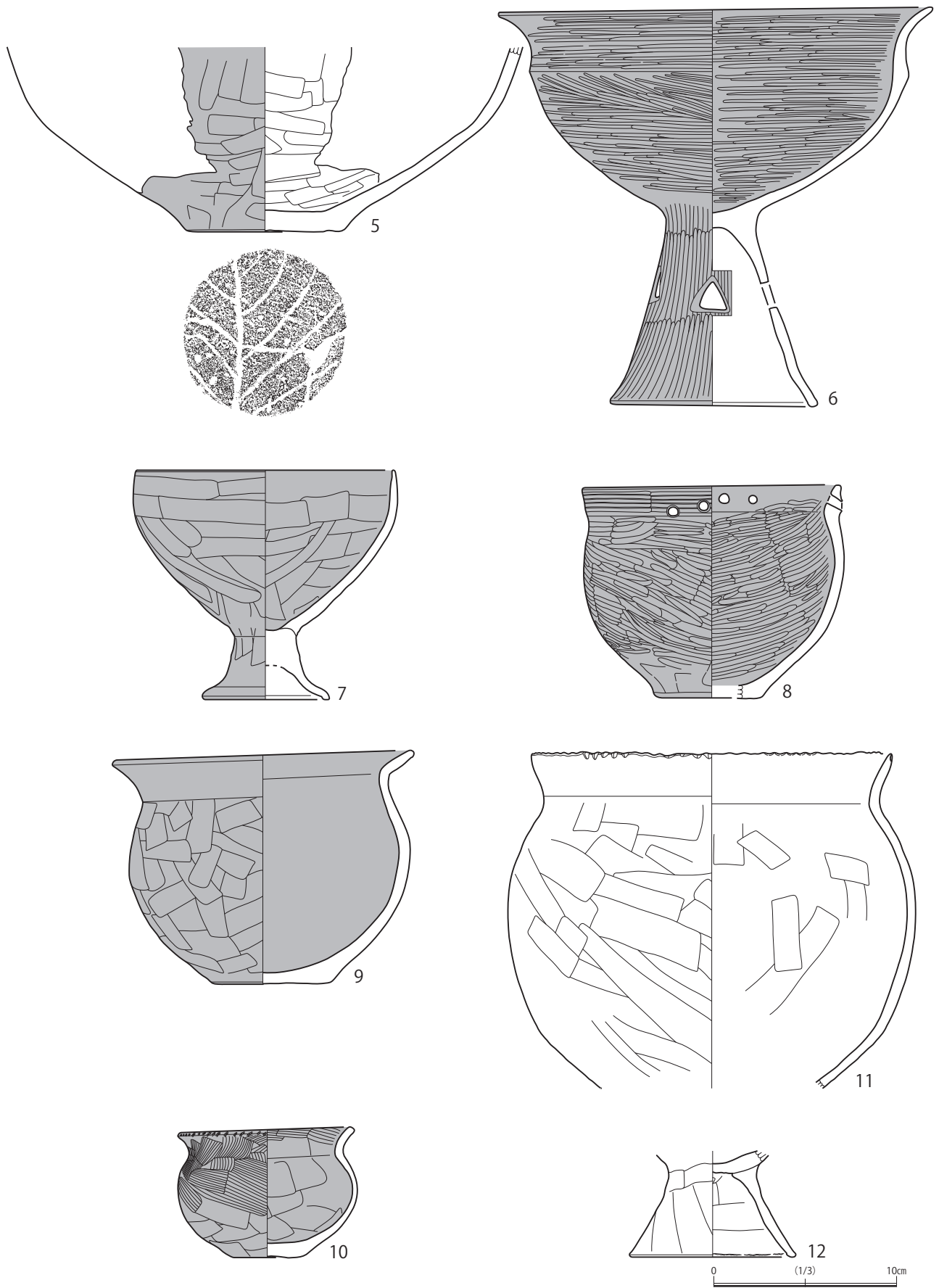
第10图 第1号周沟状遺構出土遺物実測図(2)
