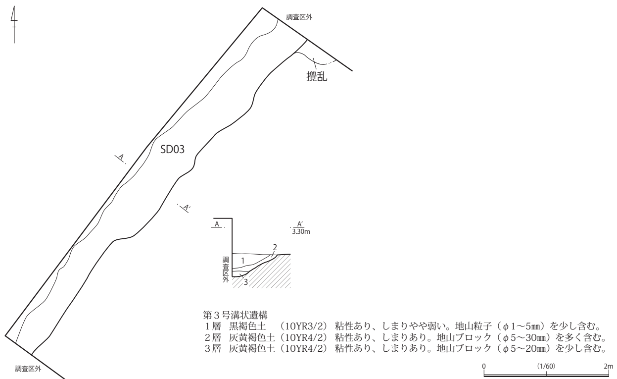
第26図 第3号溝状遺構実測図（SD03）
