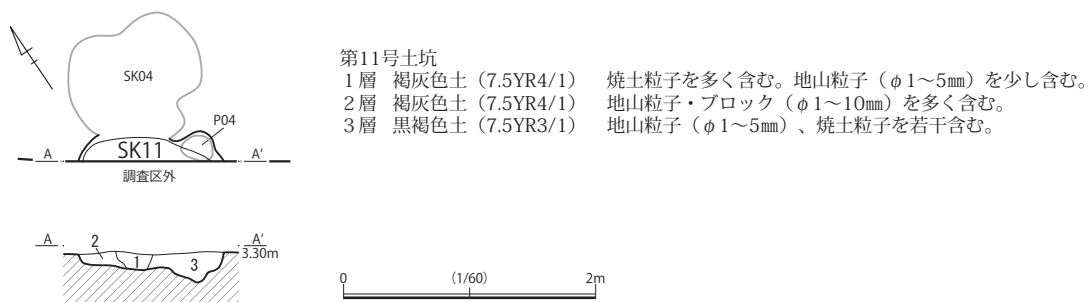
第25図 第11号土坑実測図 (SK11)
