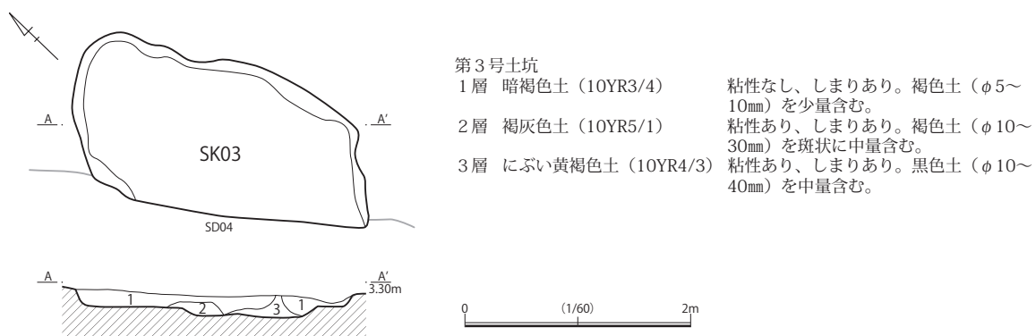
第16図 第3号土坑実測図 (SK03)
