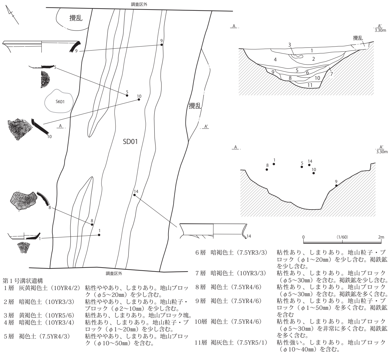
第11図 第1号溝状遺構実測図 (SD01)
