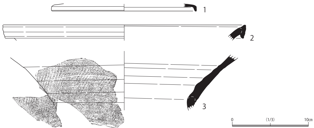
第14図 第2号溝状遺構出土遺物実測図
