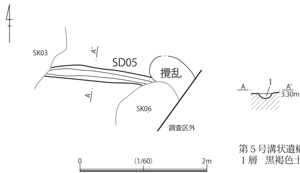
第15図 第5号溝状遺構実測図（SD05）
