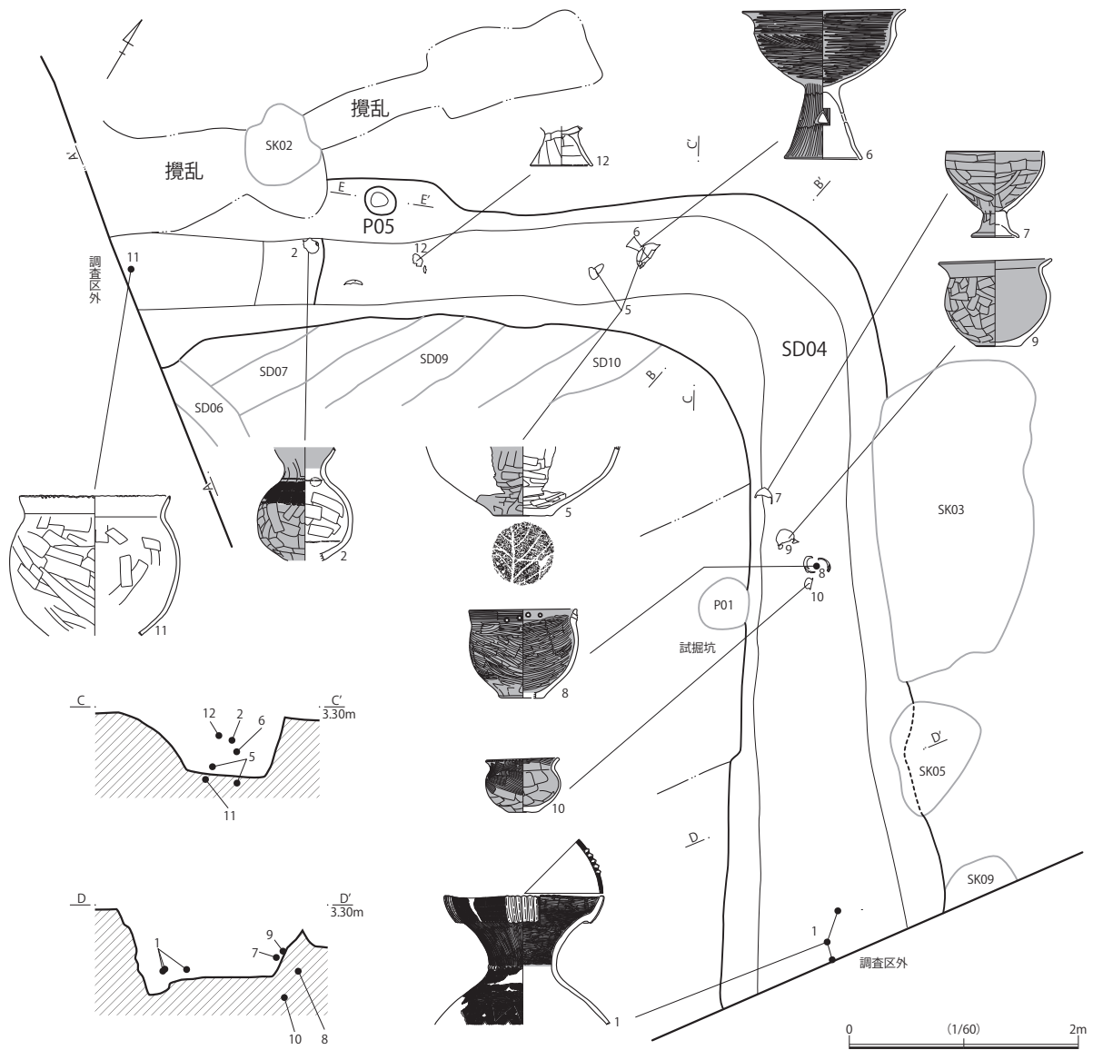
第7図 第1号周溝状遺構 (SD04)・第5号ピット (P05) 実測図 (1)
