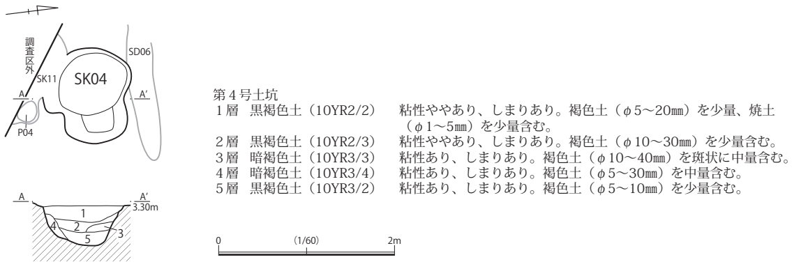
第18図 第4号土坑実測図 (SK04)
