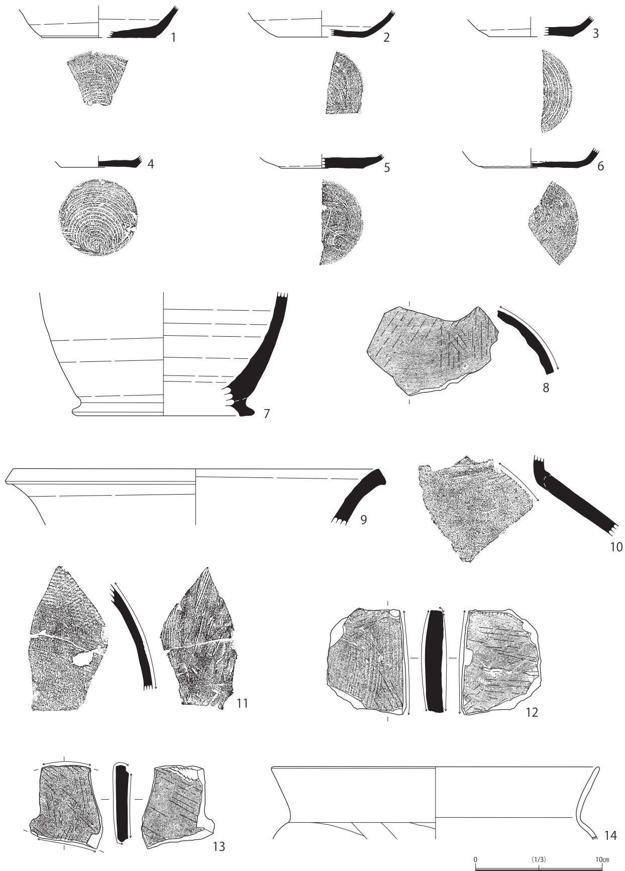
第12图 第1号沟状遺構出土遺物実測図
