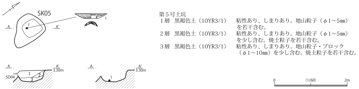
第20図 第5号土坑実測図（SK05）
