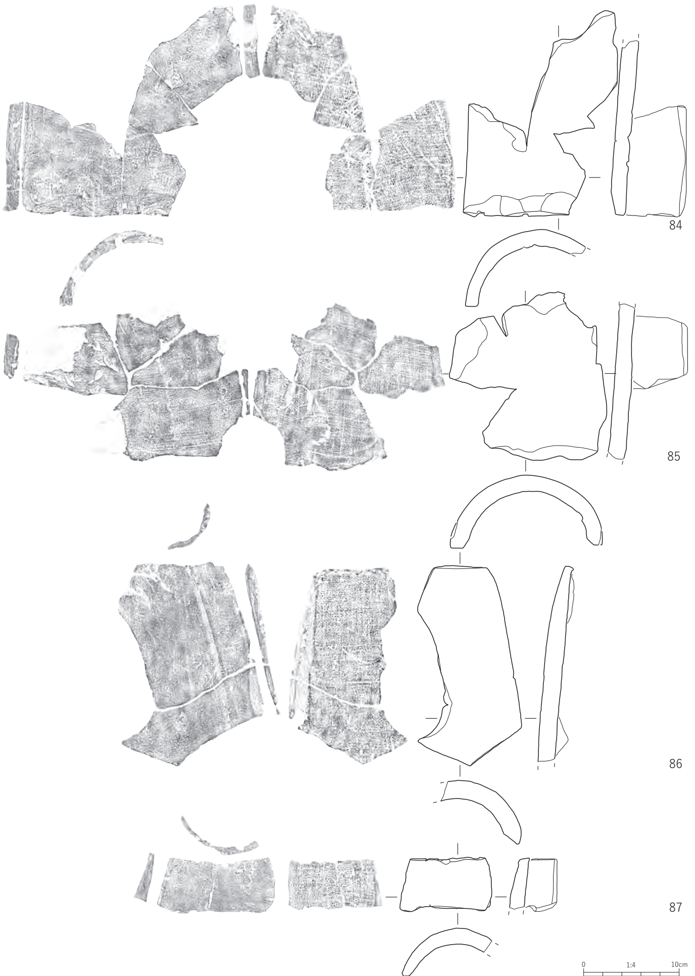
第145図 丸瓦 無段式 粘土帶桶巻づくりⅡ①類
