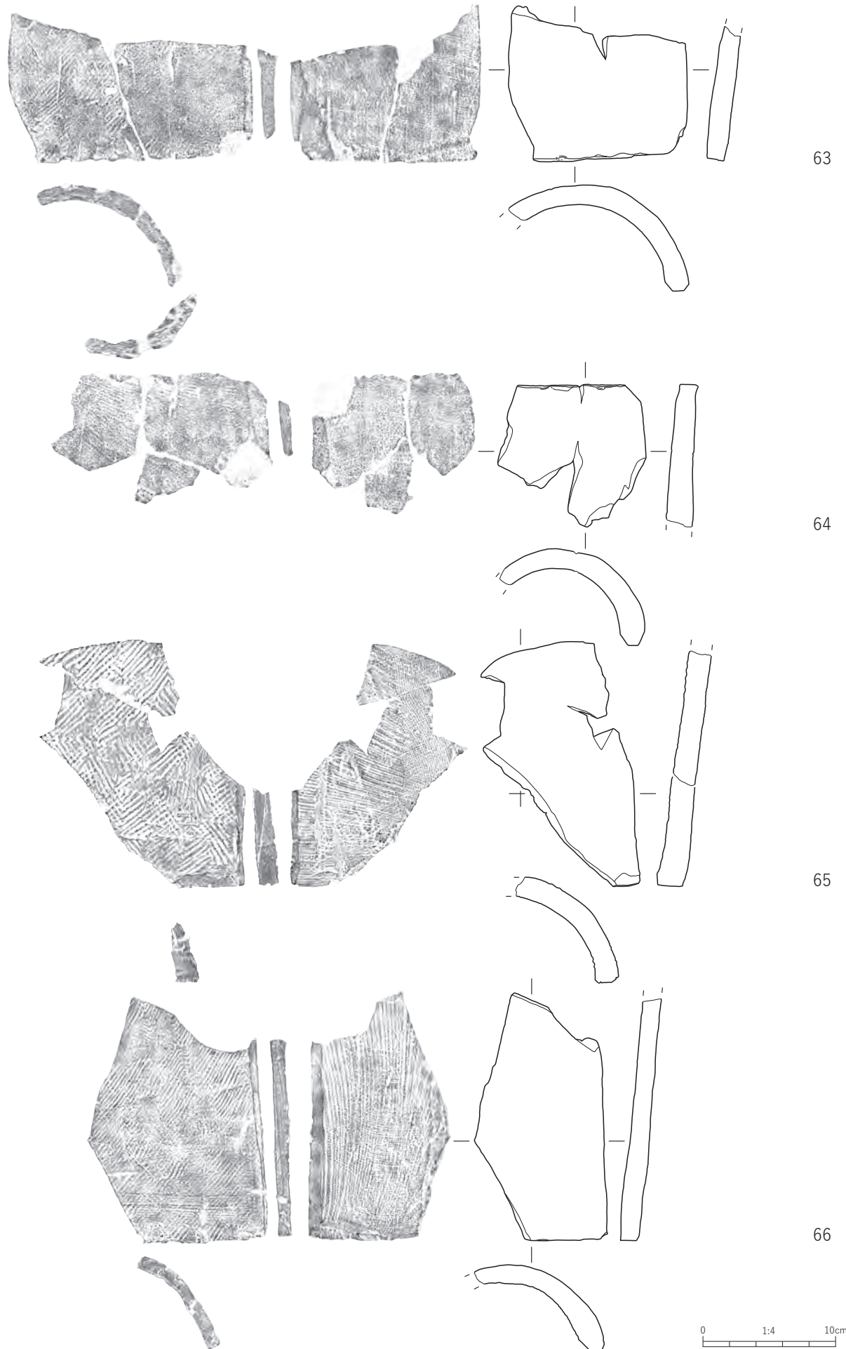
第139図 丸瓦 無段式 粘土板桶巻づくりⅡ③類
