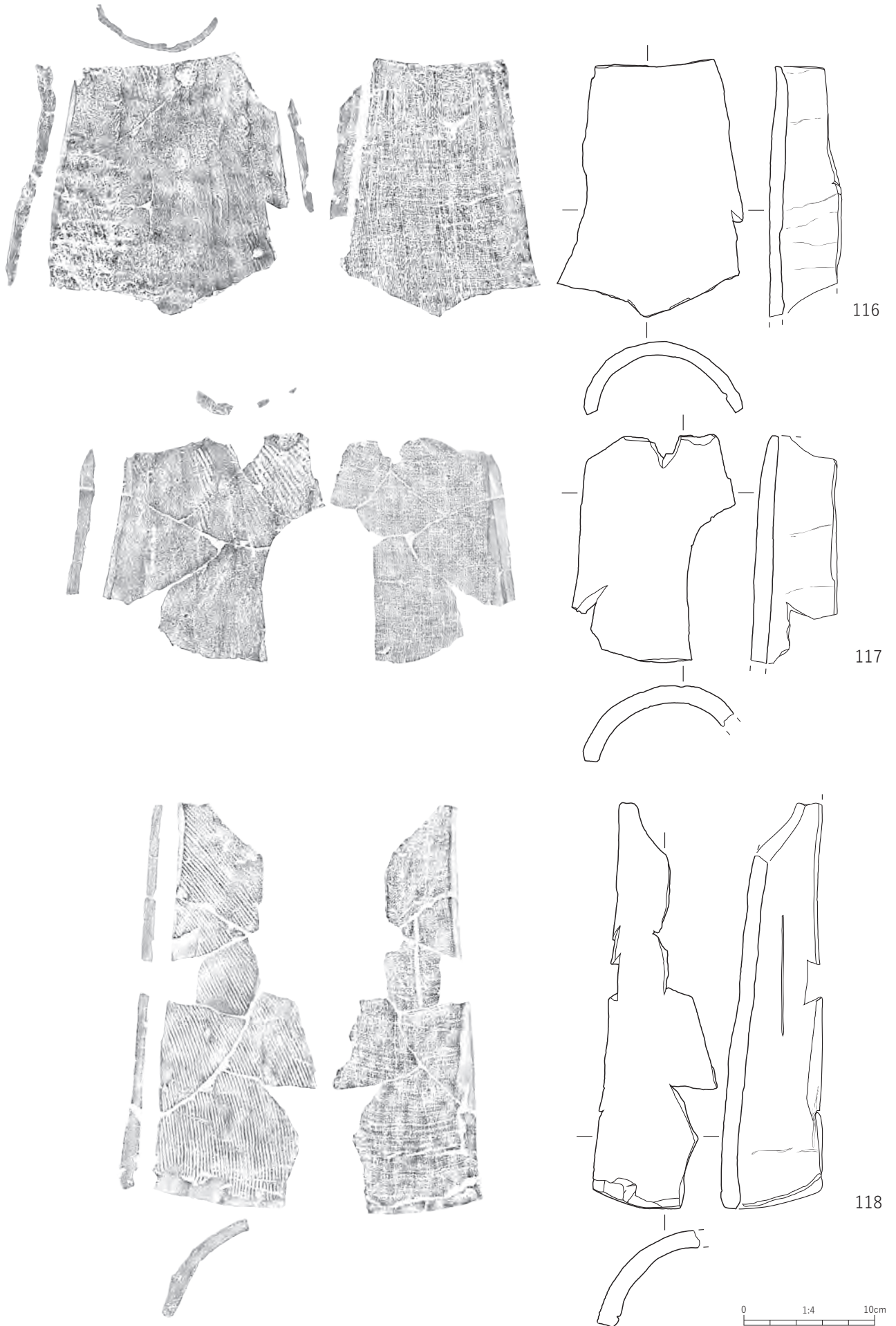
第153図 丸瓦 無段式 粘土帶桶巻づくりⅡ③類
