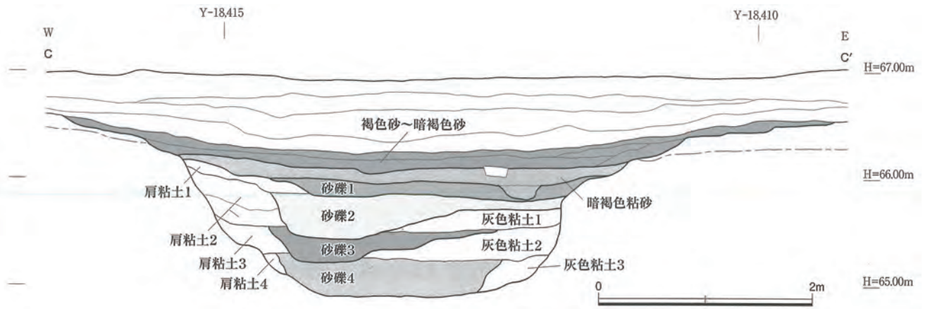
图154 SD2700断面图 1:50
