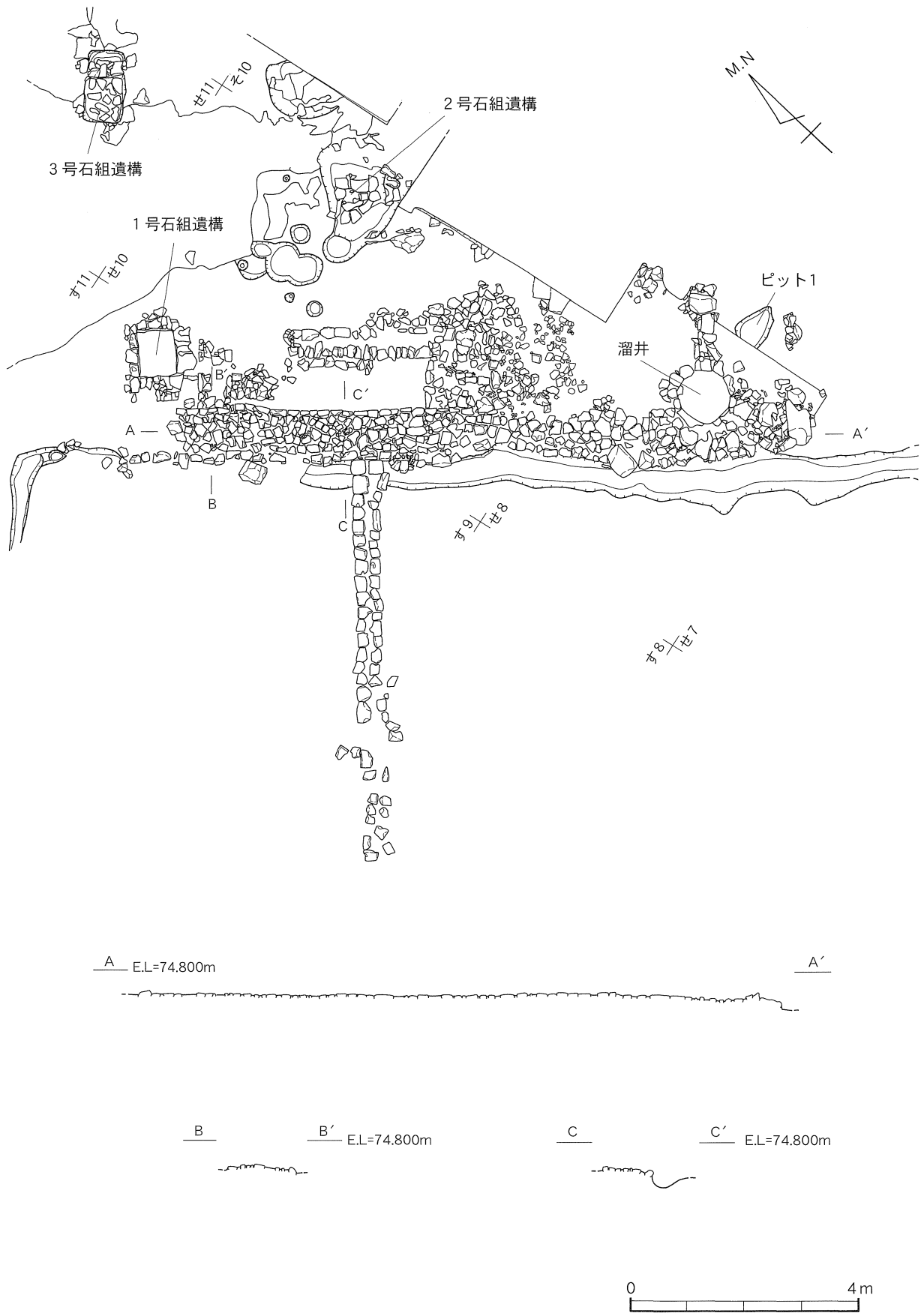
第9図 建物跡 平面図・断面図
