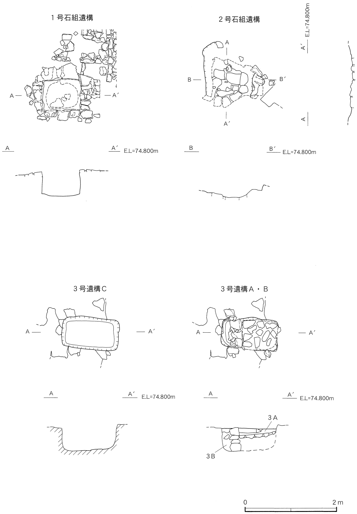
第11図 石組遺構 平面図・断面図
