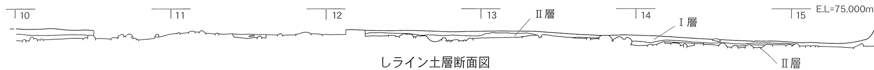
第4図 層序
