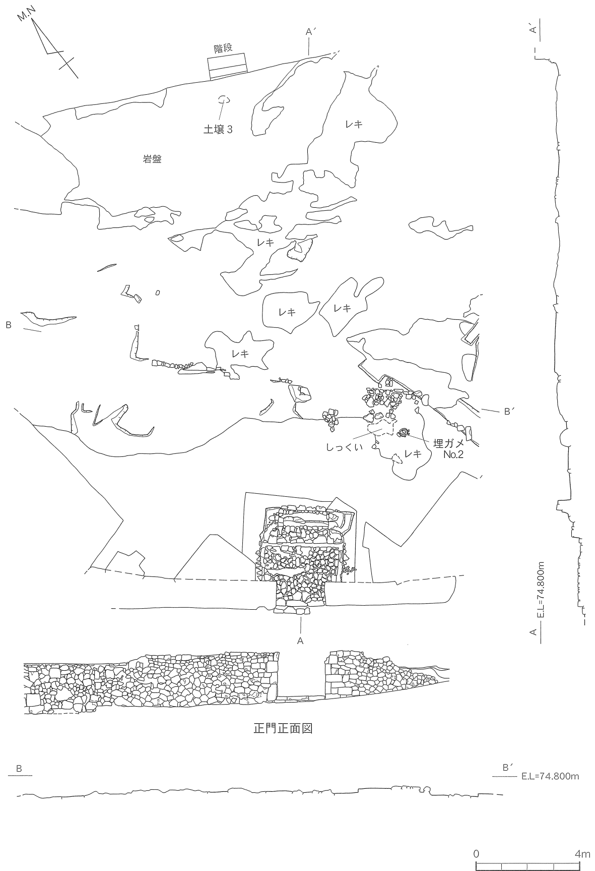
第6図 正門、本堂跡 平面図・断面図
