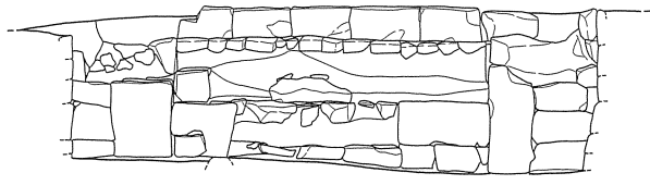
断面見通し図
