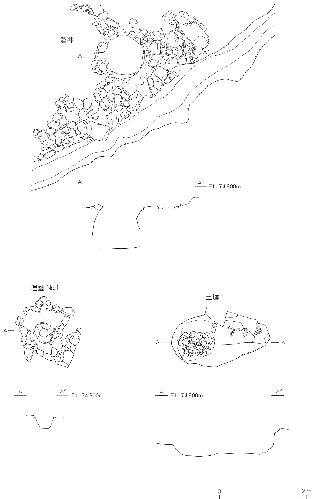
第10図 溜井、埋甕、土坑 平面図・断面図
