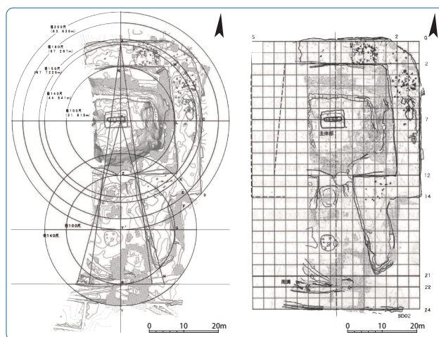
高尾山古墳の設計企画の推定(左:寺澤薫案、右:北條芳隆案)
