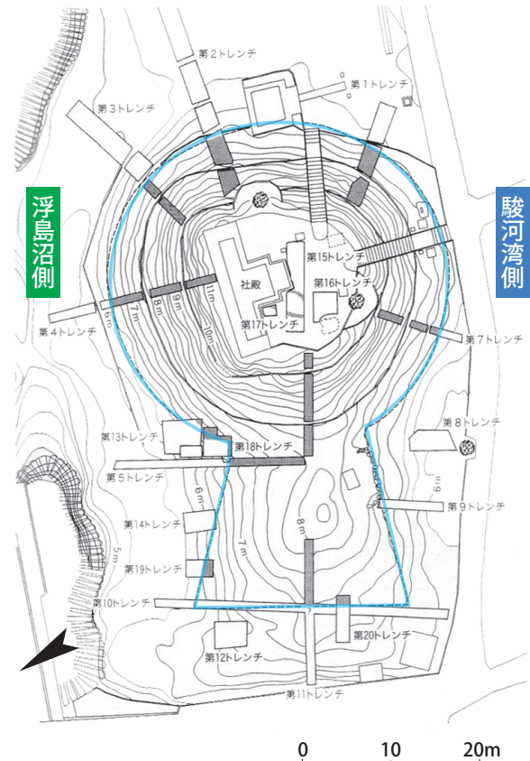
神明塚古墳測量図
