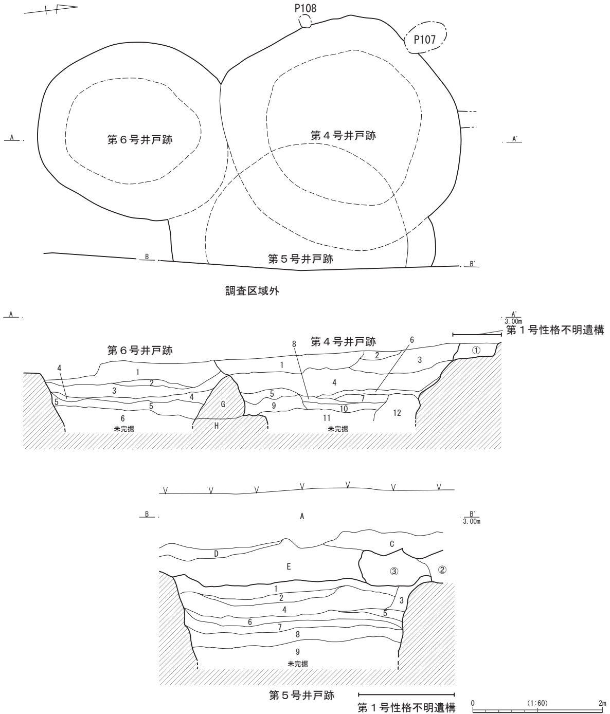
第16図 第4～6号井戸跡実測図 (SE04,SE05,SE06) (1)
