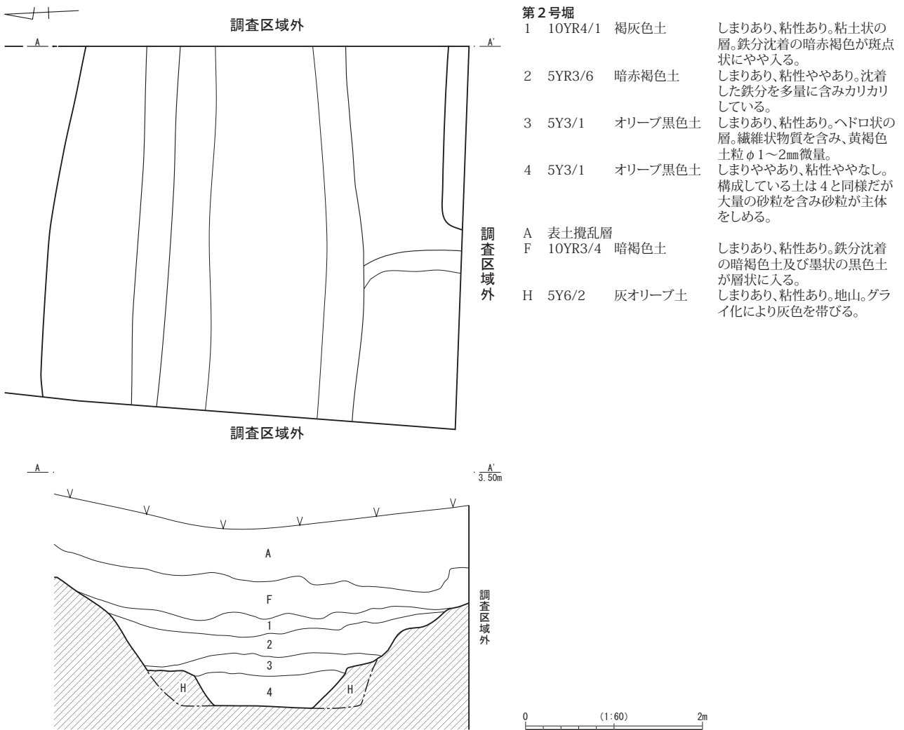
第8図 第2号堀実測図 (SA02)
