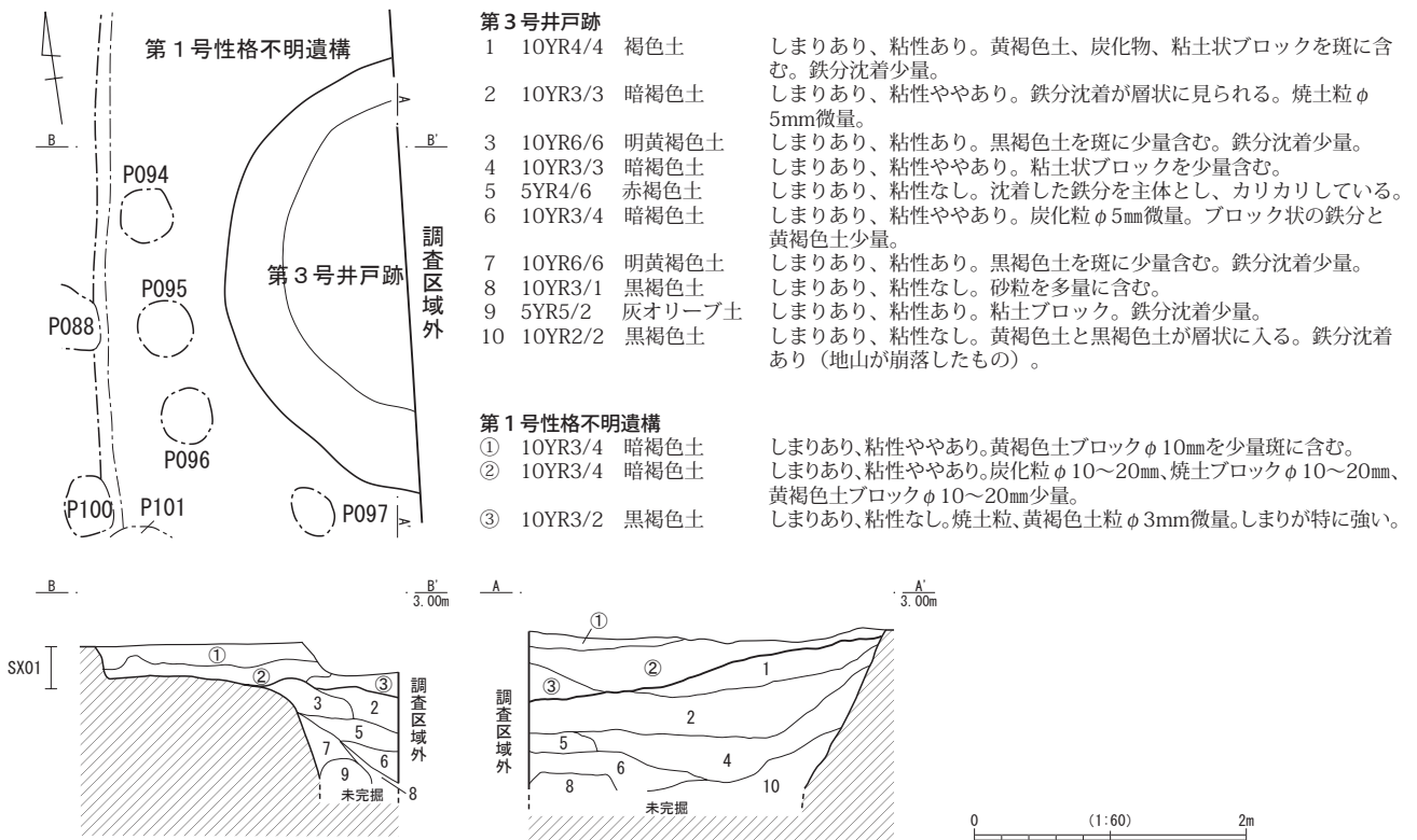
第15図 第3号井戸跡実測図 (SE03)
