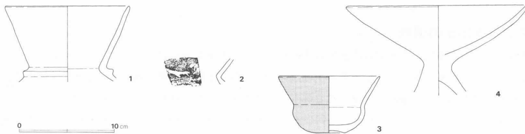
第28図 第4号土壙出土遺物実測図
