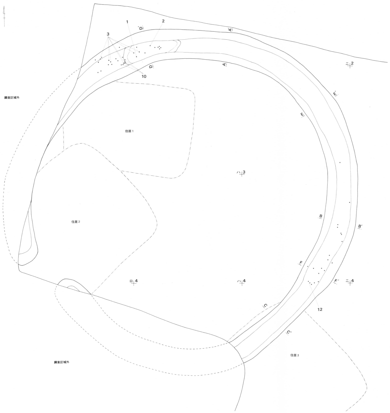
第18図 第1号方形周溝墓実測図及び遺物出土位置図
