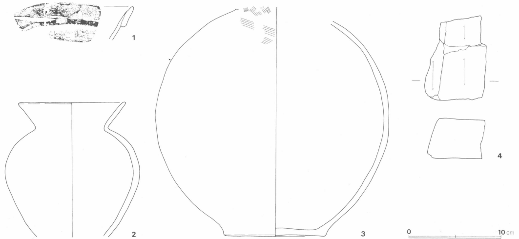
第12図 第3号住居跡出土遺物実測図
