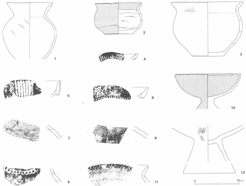
第19図 第1号方形周溝墓出土遺物実測図
