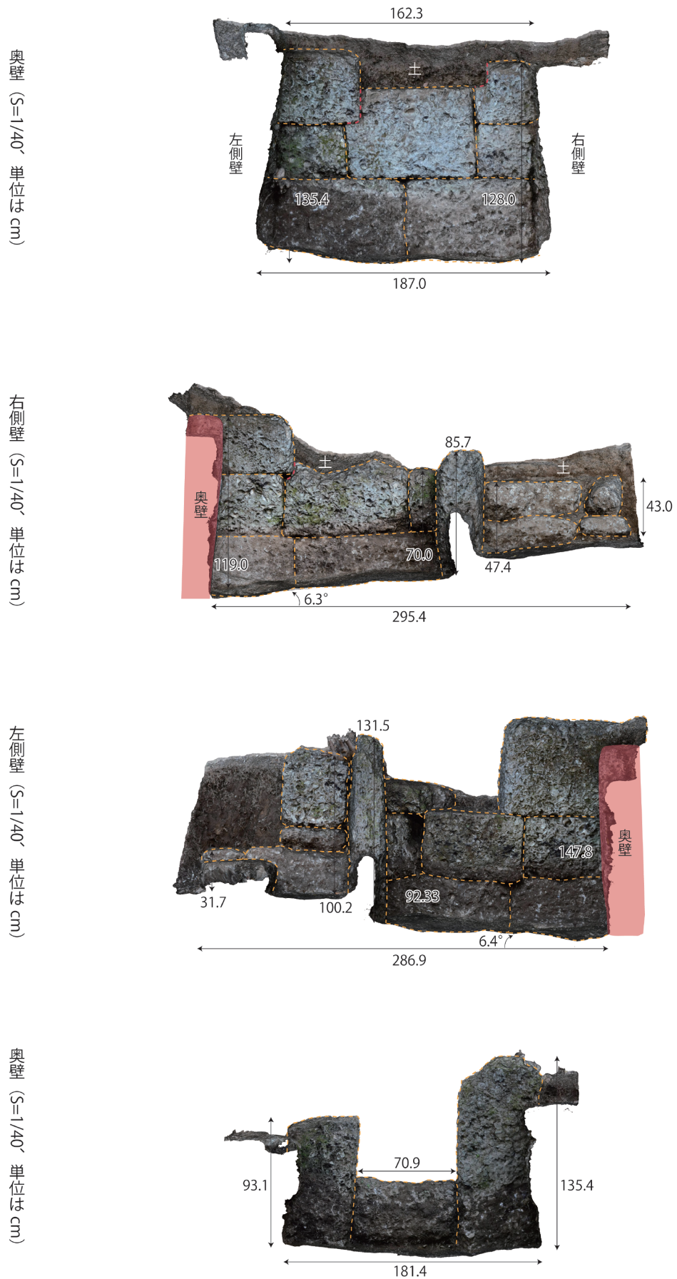
第5図 各部の計測 (S=1/40、単位は cm)
