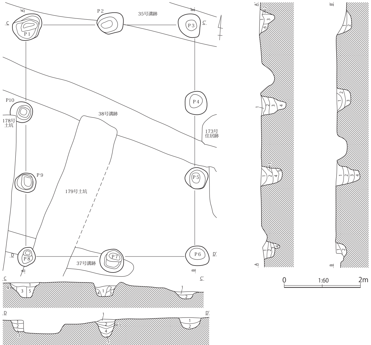
第165図 第7号掘立柱建物跡
