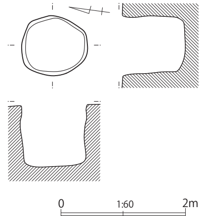
第43図 第13(1)号井戸跡
