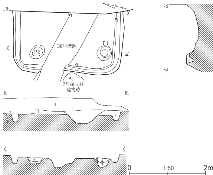
第135図 第173(SI41)号住居跡
