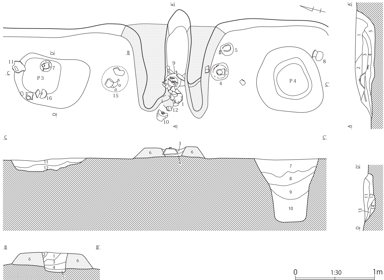
第125図 第169(SI37)号住居跡カマド
