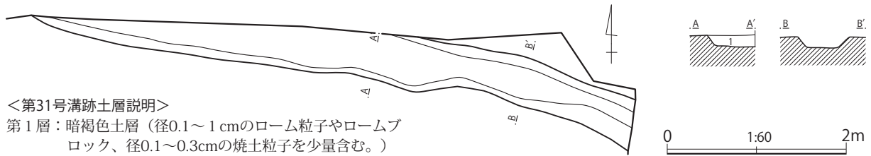
第51図 第31(7)号溝跡
