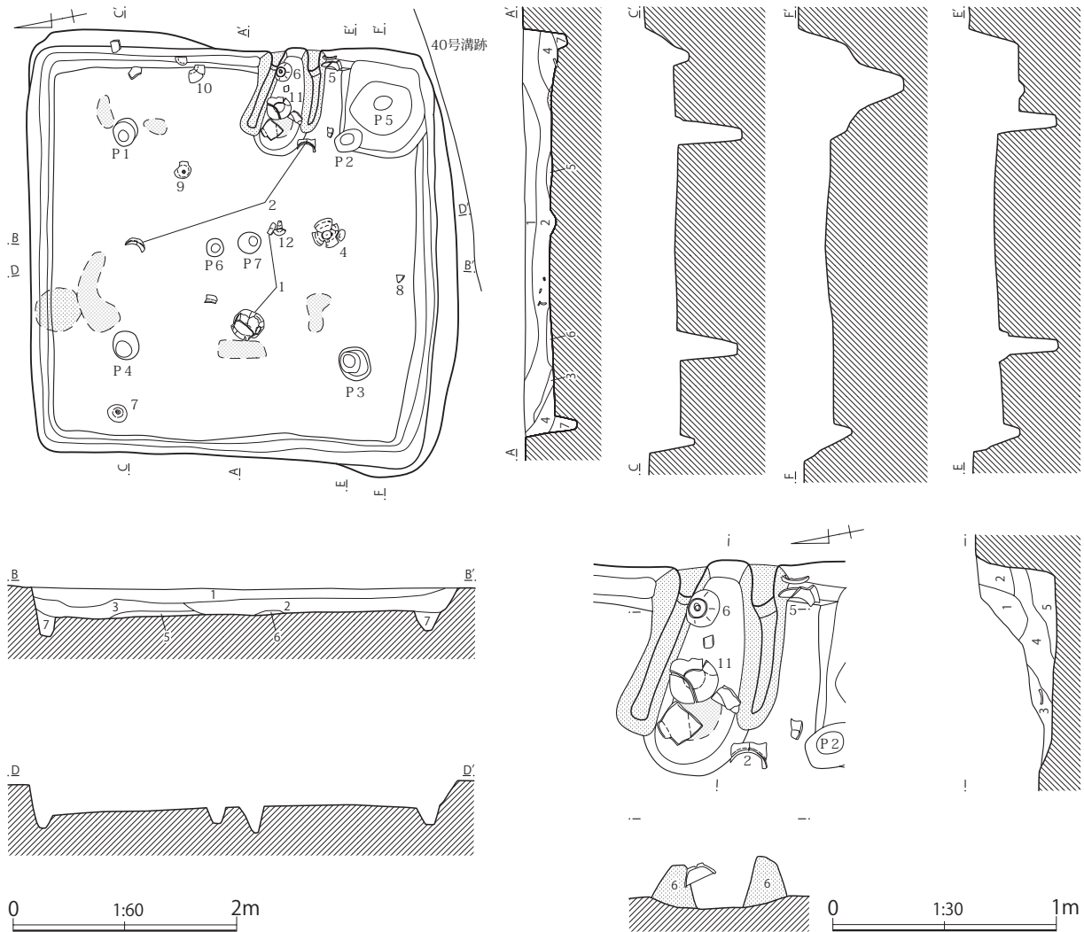
第144図 第176(SI44)号住居跡
