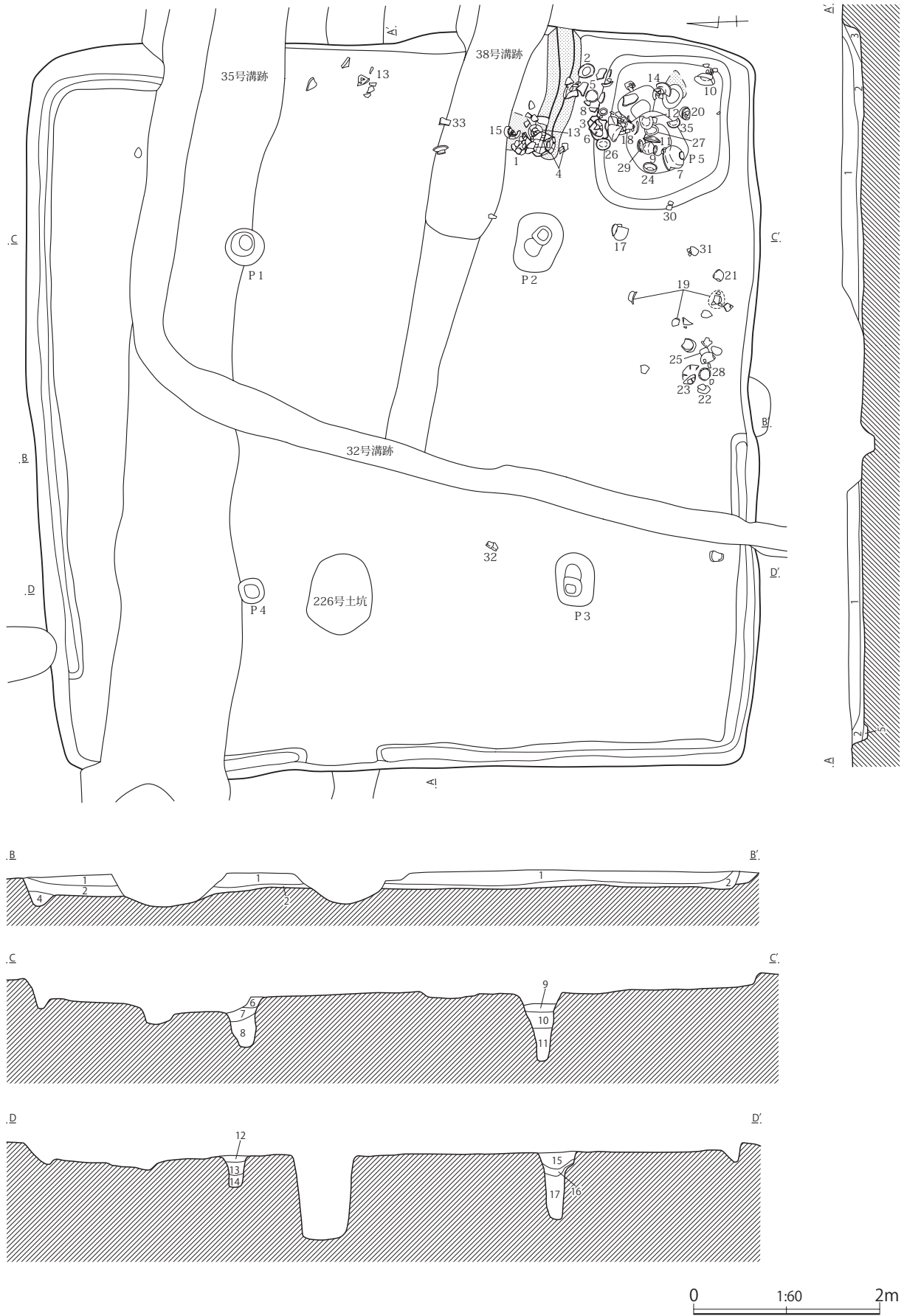
第131图 第172(SI40)号住居跡
