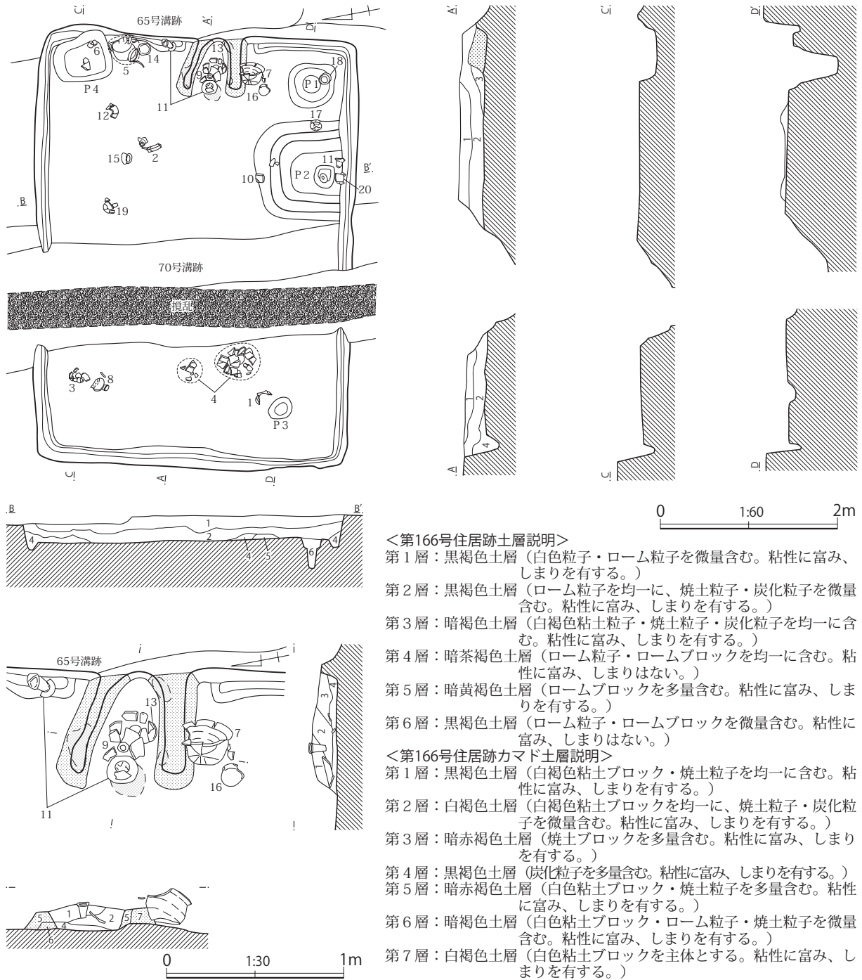
第117図 第166(S134)号住居跡
