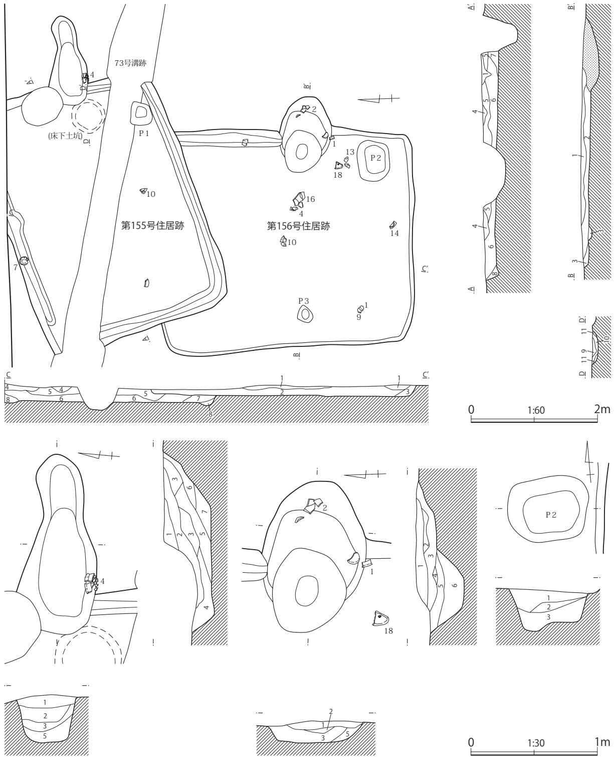
第97図 第155(SI23)・156(SI24)号住居跡
