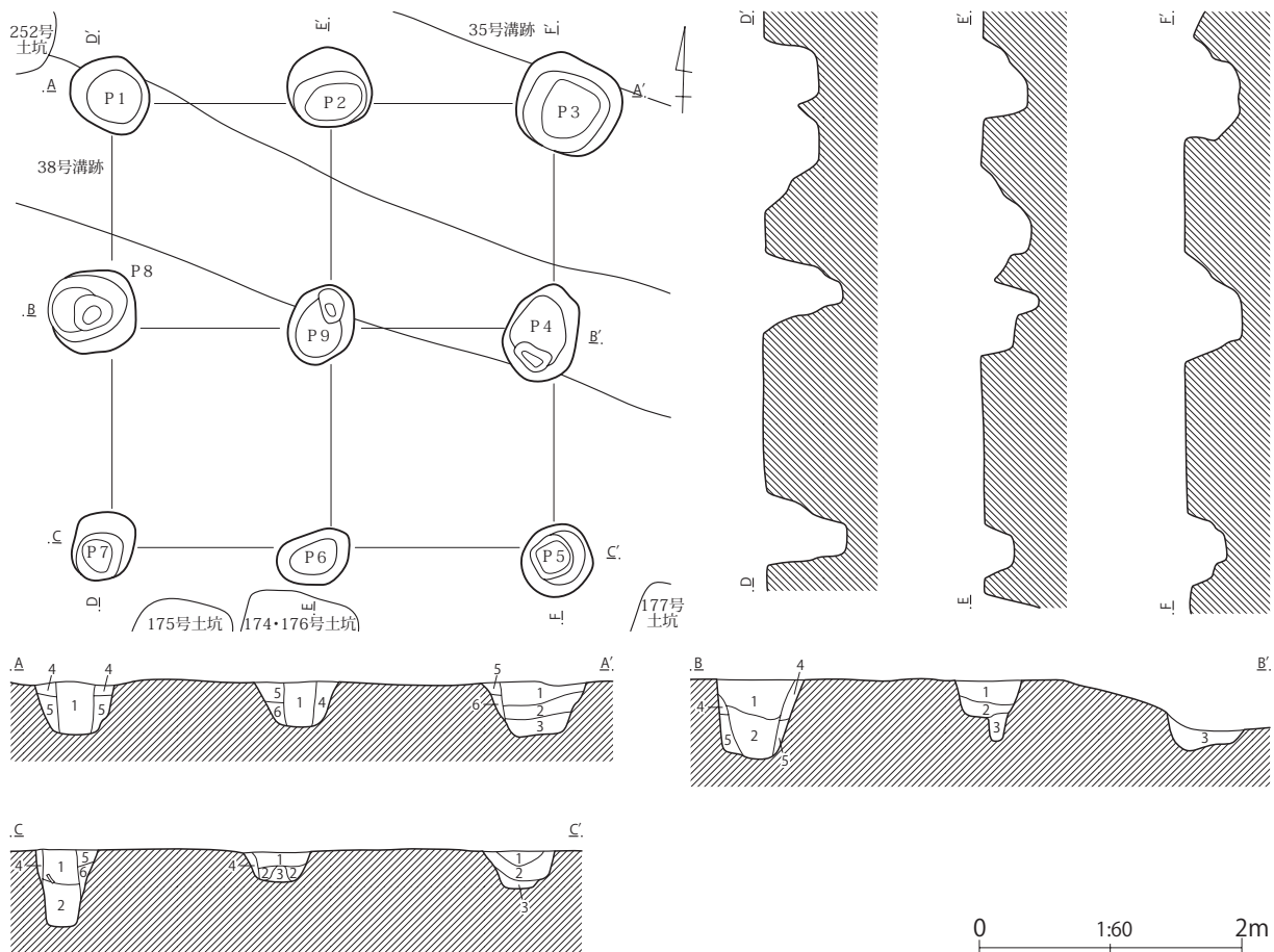
第163図 第6号掘立柱建物跡
