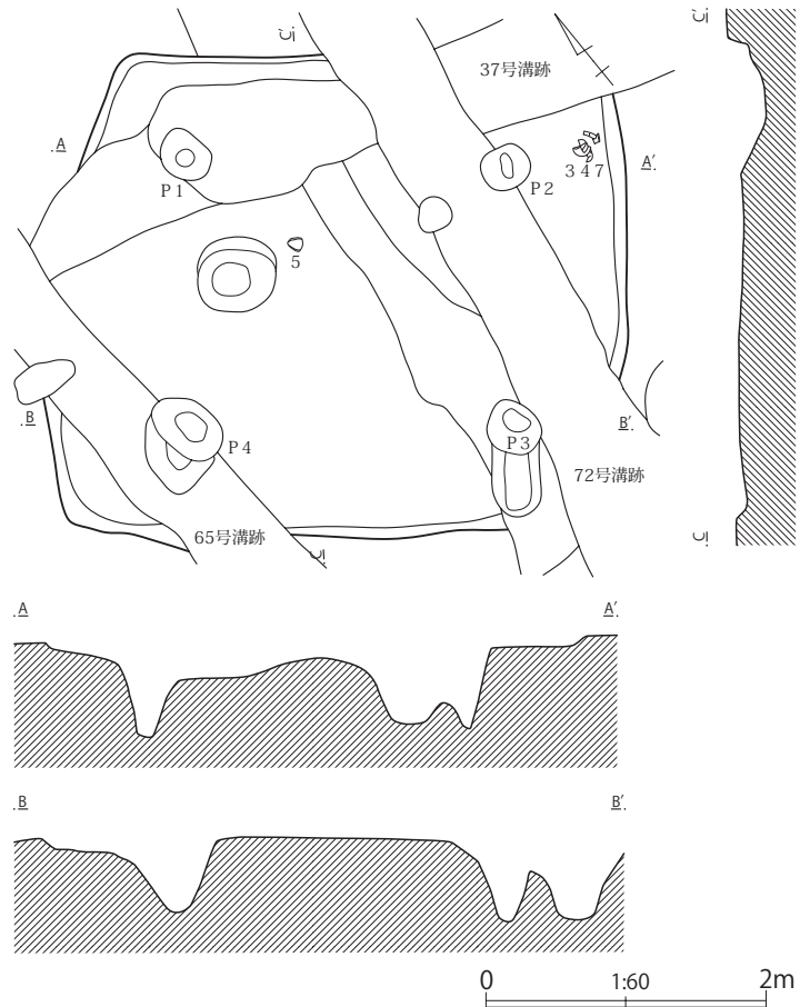
第129図 第171 (SI39) 号住居跡
