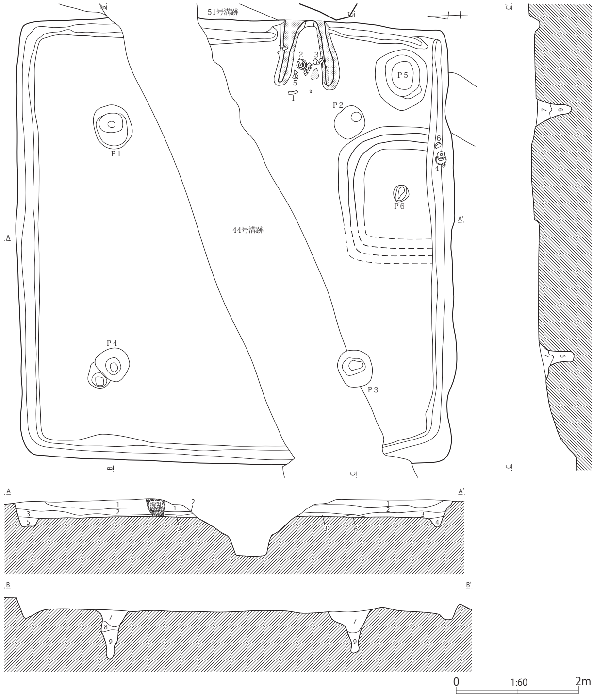
第62図 第135(SI 3)号住居跡
