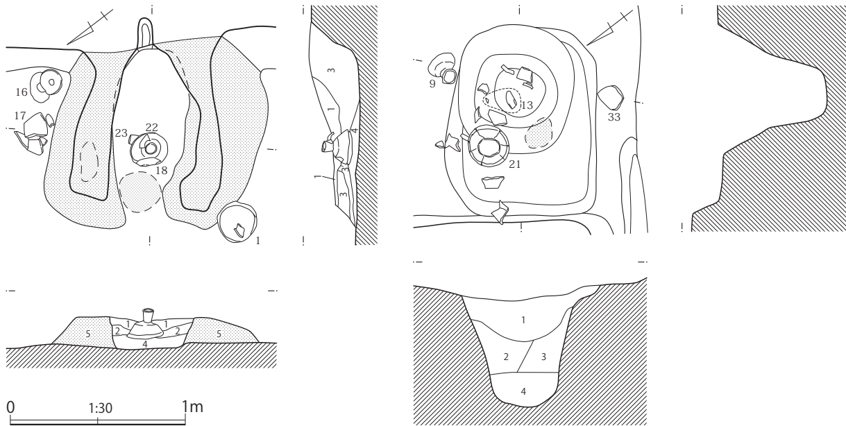
第58図 第134(SI 2)号住居跡カマド・貯蔵穴
