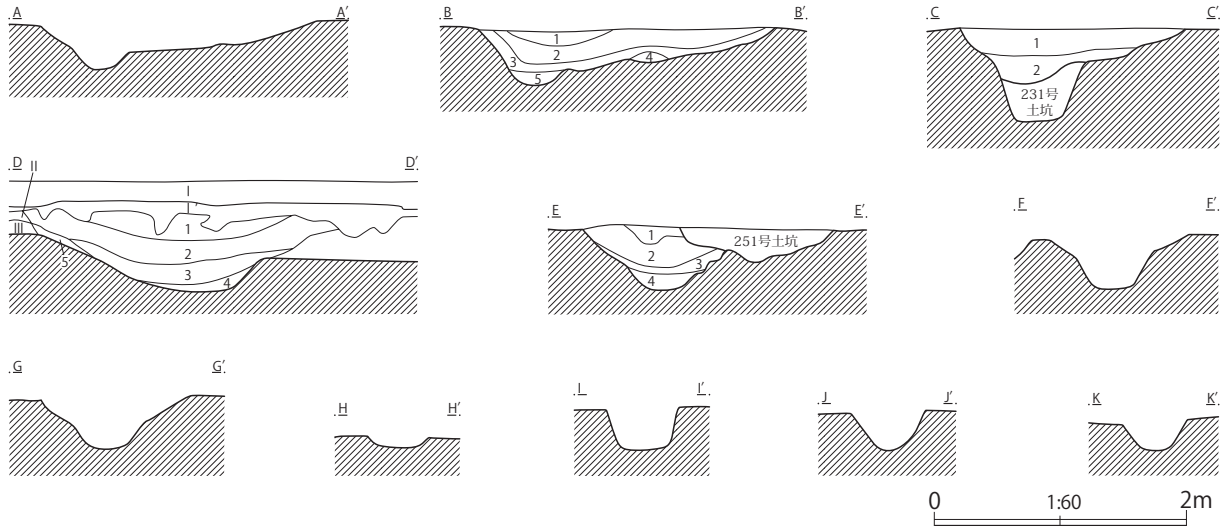
第226図 第32・35・40～42号溝跡断面図
